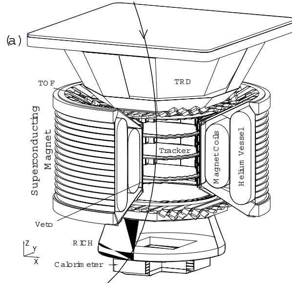
FIG. 1.9 – Vue du détecteur AMS-02.
