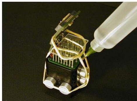
FIG. 5.2 – Injection du polymère autour du photomultiplicateur. Des élastiques et des vis de centrage sont placés au cours de cette opération pour le maintien du photomultiplicateur et de son électronique (photographie de Jean-Pierre Scordilis).
