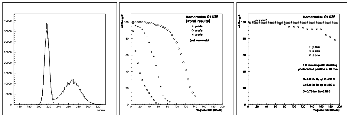
FIG. 2.6 – Résumé des principales mesures effectuées au laboratoire sur le photomultiplicateur R1635. A gauche est représentée l'excellente résolution du photoélectron unique ainsi que le piédestal. L'effet du champ magnétique sur le gain dans les 3 axes est représenté au centre. A droite, cette mesure est présentée avec un blindage de 1 mm.
