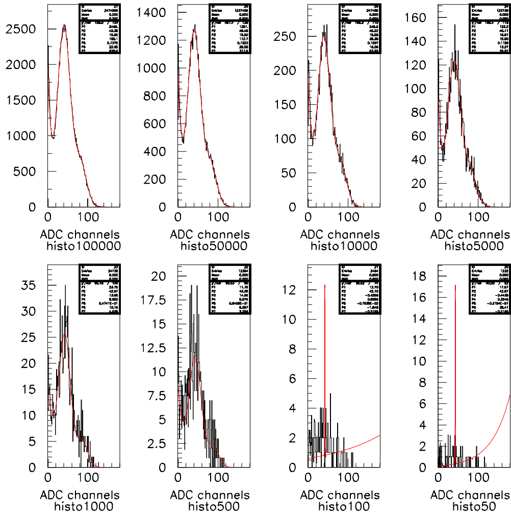
FIG. 2.36 – Simulation d'un spectre de photoélectron unique et reconstruction en fonction du nombre d'événements générés (de 100000 à 50).
