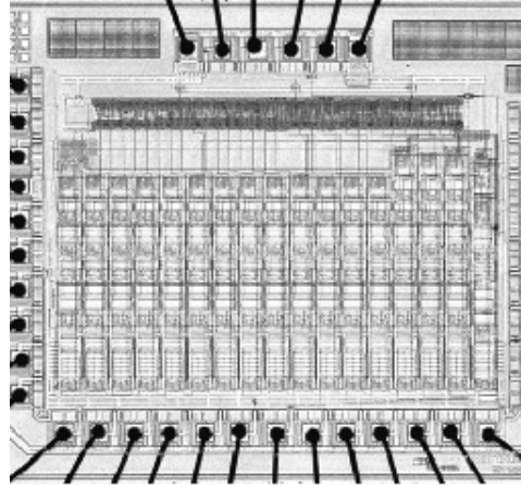
FIG. 3.7 – Photographie de l'ASIC. Sa surface est de 2.9 \times 2.2 \text{mm}^2 .
