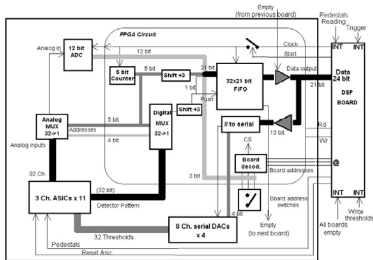
FIG. 4.7 – Architecture détaillée d'une carte de traitement des données sortant des ASICs.
