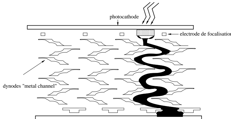
FIG. 2.7 – Vue transversale de la structure des dynodes de type "metal channel". Le principe de l'amplification est également schématisée sur cette figure.
