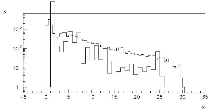
FIG. 5.6 – Comparaison du spectre de charge du faisceau obtenu par la perte d'énergie dans les scintillateurs (histogramme en trait plein) avec la distribution en abondance des rayons cosmiques (traits pointillés)[69]
