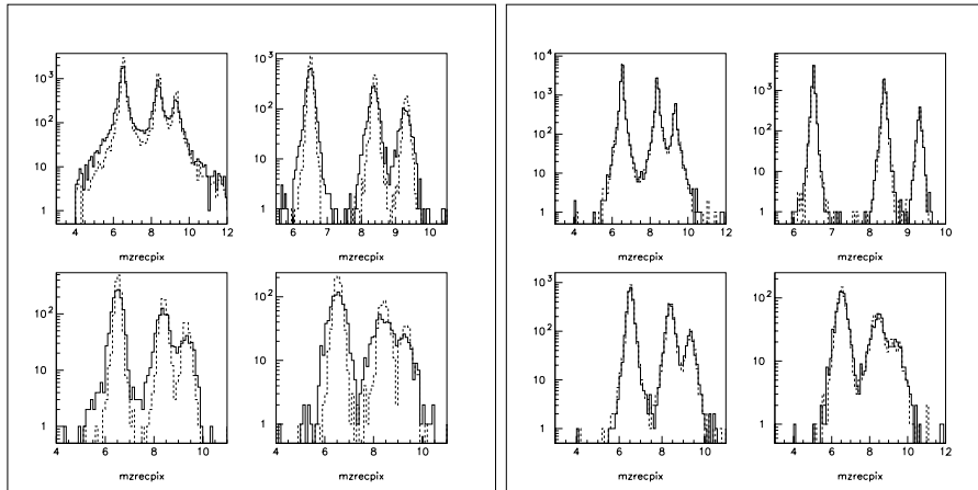
FIG. 2.10 – Comparaison des distributions simulées de masse reconstruite d'un échantillon d'événements de trois isotopes ( {}^7,{}^9,{}^{10}\text{Be} ) pour un radiateur en aérogel 1.025 (Gauche) et en NaF (Droite) pour 2 taille de pixels : 15 mm (Trait pleins) et 7.5 mm (Pointillés). Dans chaque cas les 4 histogrammes correspondent à 4 gammes d'impulsions : 5-13 GeV/c, 5-8 GeV/c, 8-10 GeV/c, 10-12 GeV/c.
