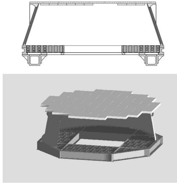
FIG. 1.17 – Vue du détecteur RICH.
