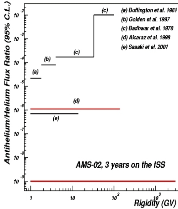
FIG. 1.1 – Sensibilité d'AMS pour la recherche d'antimatière.
