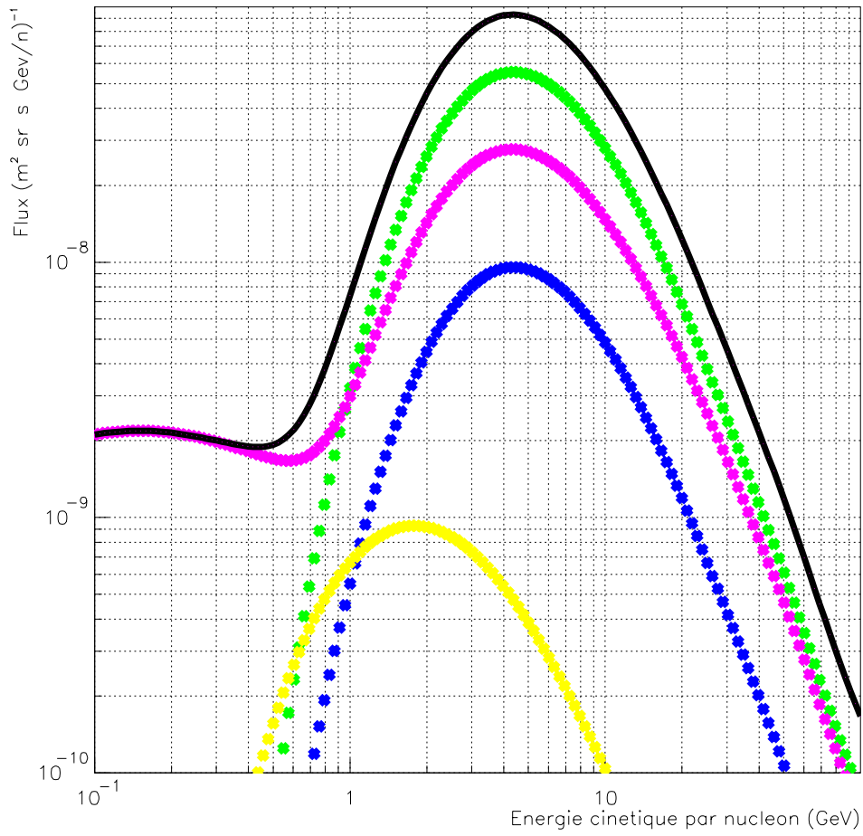
FIG. 9.4 – Contributions au flux de \bar{D} venant (de haut en bas) de tous les processus, des interactions p + p , des pertes d'énergie, des interactions avec les noyaux et des interactions \bar{p} + p .
