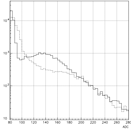
FIG. 2.22 – Comparaison de la réponse du photomultiplicateur à une baisse de la haute tension d'alimentation ( \rightsquigarrow baisse du gain) en traits pleins et à une augmentation du champ magnétique ( \rightsquigarrow baisse du gain \times efficacité quantique) en traits pointillés.
