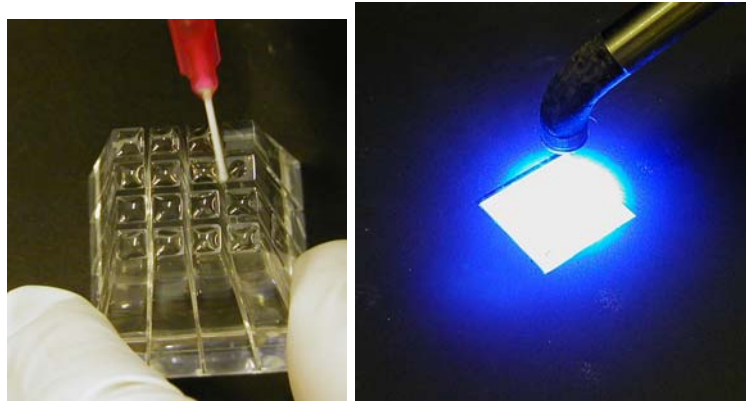
FIG. 5.3 – Installation des guides de lumière sur le photomultiplicateur. Gauche : une croix est dessinée dans la colle optique pour favoriser sa diffusion sur la fenêtre d'entrée; droite : la colle est polymérisée, un cache est placé sur les photomultiplicateurs voisins.
