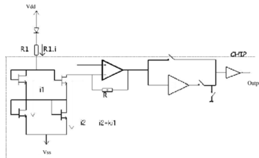
FIG. 3.11 – Schéma du montage de correction de la dérive des piédestaux en fonction de la température.
