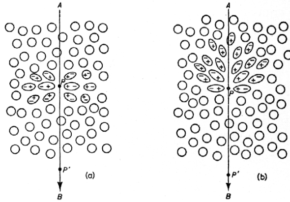
FIG. 1.12 – Polarisation induite par le passage d'une particule chargée (a) à faible vitesse (b) à grande vitesse.
