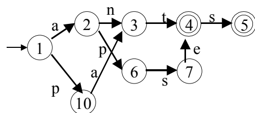
Fig.5. Un automate minimal
