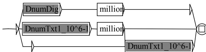
Fig.31. Graphe DnumTxt1_{10^{12}-1} : cardinaux positifs inférieurs à 10^{12} .
