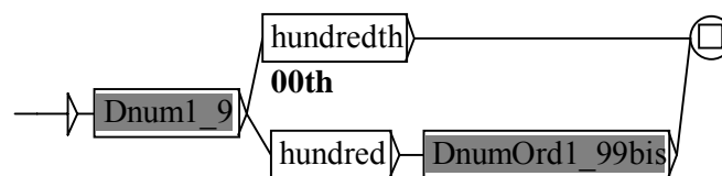
Fig.40. Graphe DnumOrd100_999 : ordinaux de 100 à 999.
