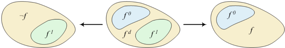
Figure 3.5: Élargissement de la fonction trivaluée f
