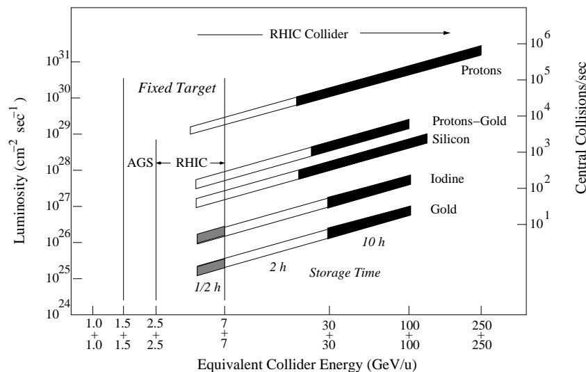
FIG. 2.2: Caractéristiques du RHIC en fonction des systèmes.
