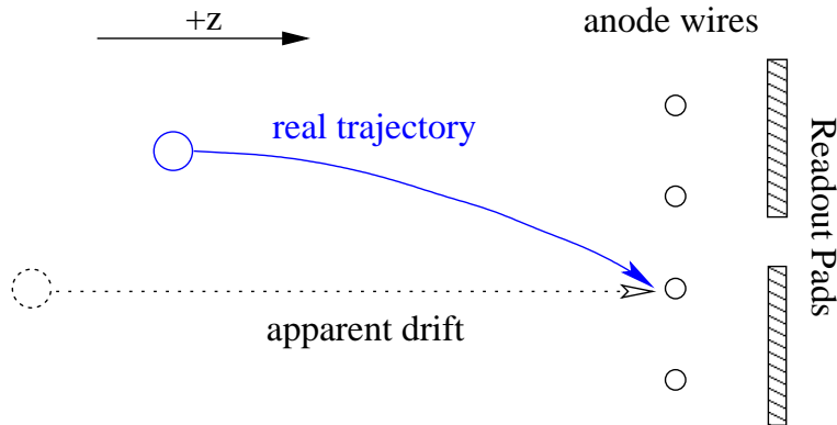
FIG. 3.2: Conséquence d'un champ magnétique non uniforme et corrections \vec{E} \wedge \vec{B} .
