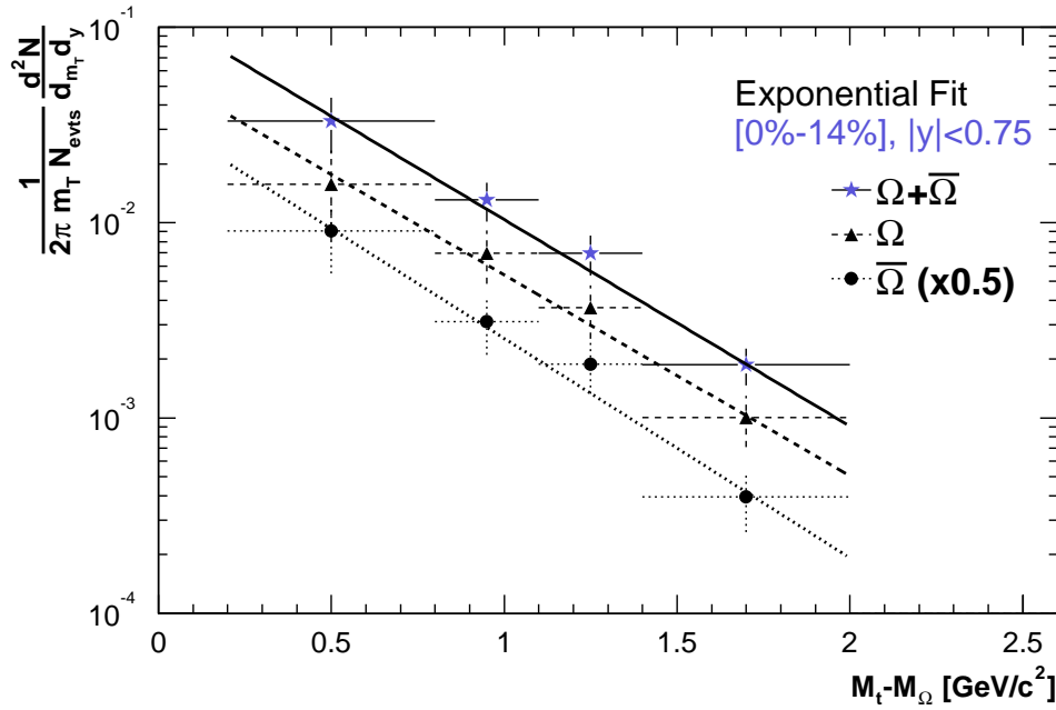
FIG. 5.24: Spectres en masse transverse corrigés et ajustés par une exponentielle pour l'intervalle de centralité [0 % – 14 %]. Un facteur d'échelle de 0,5 est appliqué au spectre des \bar{\Omega}^+ pour des raisons de lisibilité.
