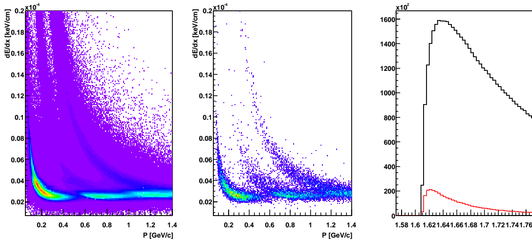
FIG. 5.6: Perte linéique d'énergie des produits de décroissance des \Omega . La distribution de gauche et celle en masse invariante à droite et en noir correspondent à une sélection en dE/dx de 5\sigma . La distribution centrale est celle des produits de décroissance une fois la sélection à 3\sigma appliquée. La distribution en masse invariante des candidats \Omega sélectionnés est représentée en rouge.
