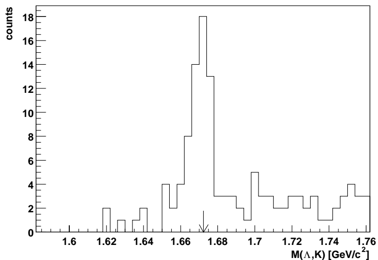
FIG. 5.23: Distribution en masse invariante des \Omega^- + \bar{\Omega}^+ pour les événements "minimum bias".
