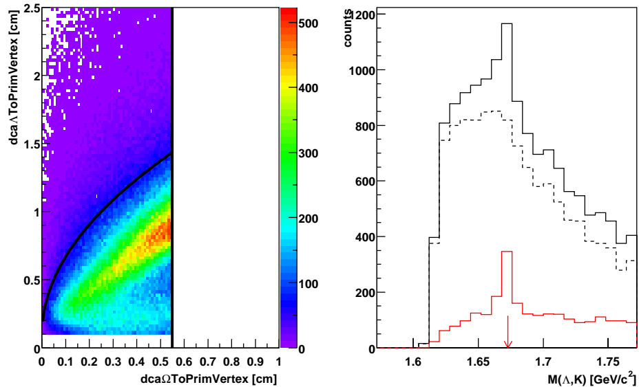
FIG. 5.8: Sélection corrélée sur la dca du \Lambda au vertex primaire en fonction de celle du \Omega .
