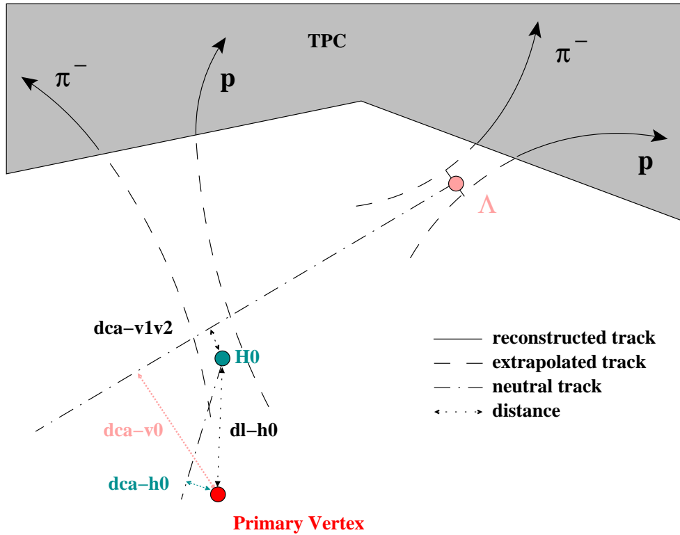
FIG. 3.8: Reconstruction des vertex de type "H0".
