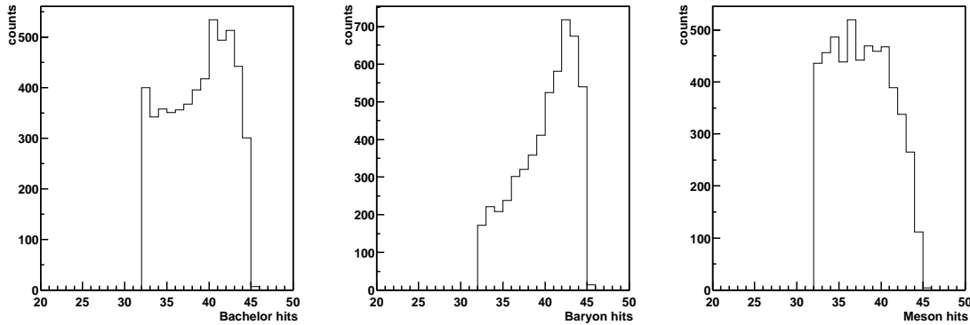
FIG. 5.3: Nombre de points dans la TPC pour les traces des produits de décroissances des \Omega . Les différentes formes s'expliquent par les masses des particules: les particules les plus lourdes (notés Baryons, c'est-à-dire les p et les \bar{p} issus des \Lambda et des \bar{\Lambda} ) laissent en moyenne plus de points dans la TPC.
