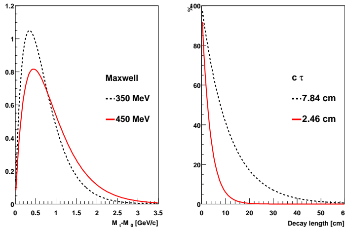
FIG. 4.1: Distributions maxwelliennes de la différence entre la masse transverse et la masse de particule ( M_t - M_0 à gauche, pour T = 350 MeV et T = 450 MeV), et distance de vol en fonction du temps de vie (à droite, c\tau_\Omega = 2.46 cm et c\tau_\Lambda = 7.84 cm).
