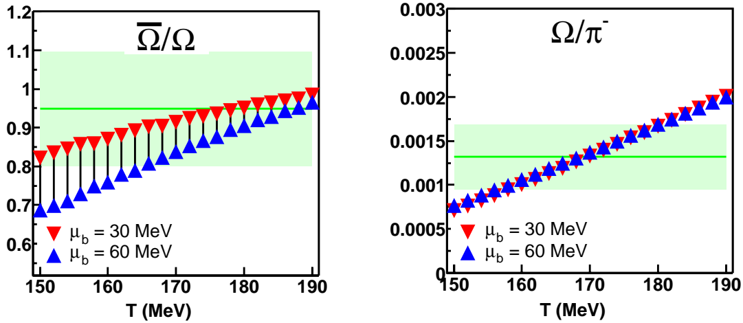
FIG. 6.3: Calcul relatif au modèle statistique montrant la dépendance en température et en potentiel chimique des rapports \bar{\Omega}^+/\Omega^- (à gauche) et \Omega^-/\pi^- (à droite). Les intervalles correspondant aux prédictions du modèle thermique statistique sont représentés par les différents traits et dépendent de la valeur de \mu_B . Les résultats (traits verts) de notre étude sont en accord avec le modèle compte tenu des erreurs statistiques de mesure (bande vert clair).
