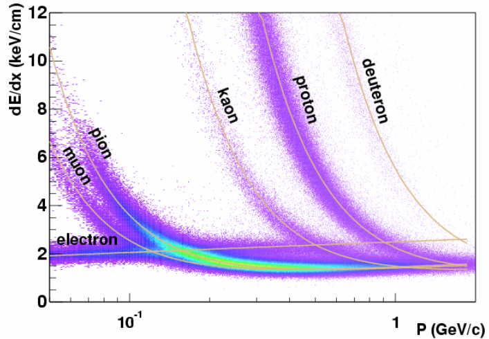
FIG. 5.4: Identification de particule par perte linéique d'énergie dans la TPC.
