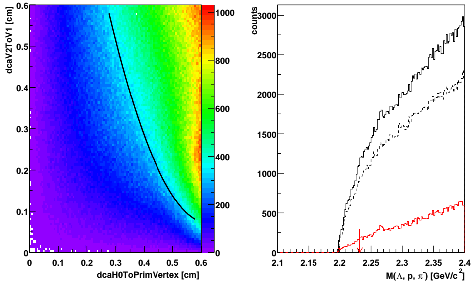
FIG. 5.10: Sélection corrélée sur la dca du \Lambda au vertex primaire en fonction de celle du H0 .
