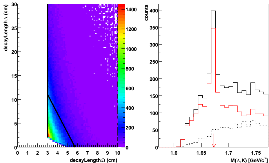
FIG. 5.9: Sélection corrélée sur la distance de vol du \Lambda en fonction de celle du \Omega .
