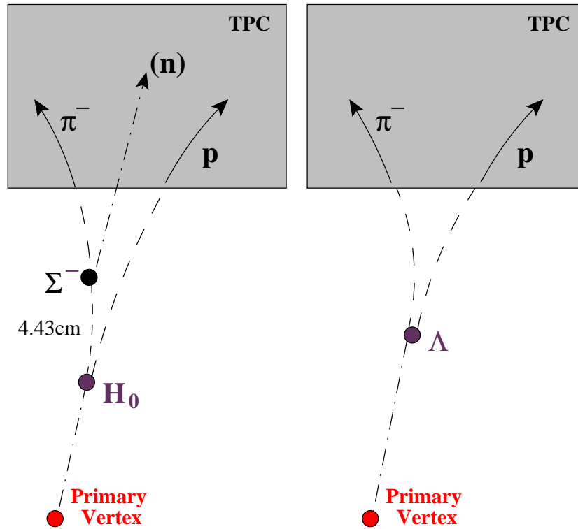
FIG. 3.11: Reconstruction erronée d'un H0 \rightarrow \Sigma^- p (figure de gauche) pouvant donner lieu à un \Lambda (figure de droite).
