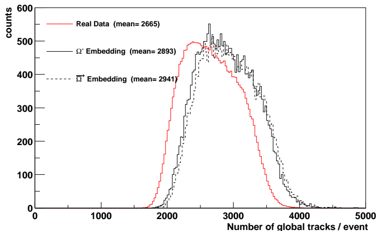
FIG. 4.10: Distribution du nombre de traces globales par événement. Les distributions correspondants aux événements réels sont représentés en rouge tandis que celles des événements d’embedding” sont respectivement en trait plein ( \Omega^- ) et pointillé ( \Omega^+ ).
