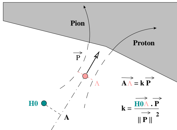
FIG. 3.9: Condition de causalité pour le \Lambda issu d'un H0 .
