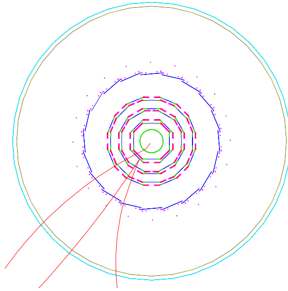
FIG. 4.2: Simulation de la désintégration d'un \Xi^- \rightarrow \Lambda \pi^- en vue de la détermination de l'efficacité du trajectographe interne de STAR (projection transverse extraite de [SUI01]).
