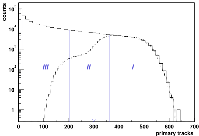
FIG. 5.2: Distribution du nombre de traces primaires par collision dans le cas du déclenchement “minimum bias” en trait plein et “central” en pointillé.
