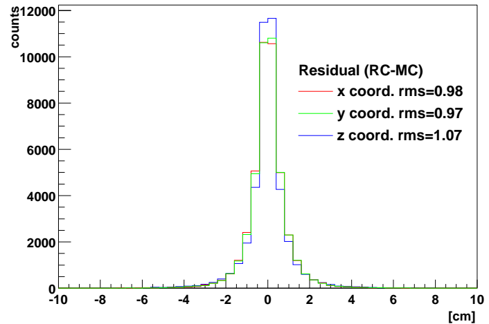
FIG. 4.6: Résolution spatiale de la reconstruction des \Xi vertex dans la TPC.
