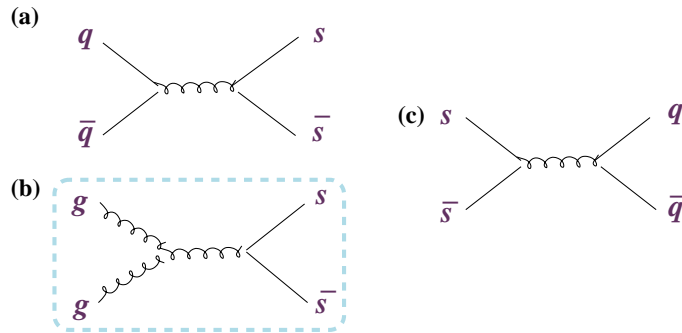
FIG. 1.4: Mécanismes de production de paires s\bar{s} dans un QGP par (a) annihilation q\bar{q} , (b) fusion de gluons et mécanisme d'annihilation de l'étrangeté (c).
