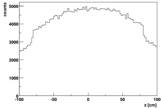
FIG. 5.1: Distribution de la position du point d'interaction suivant l'axe du faisceau dans le cas de l'échantillon des événements centraux et pour la première année de fonctionnement de RHIC.
