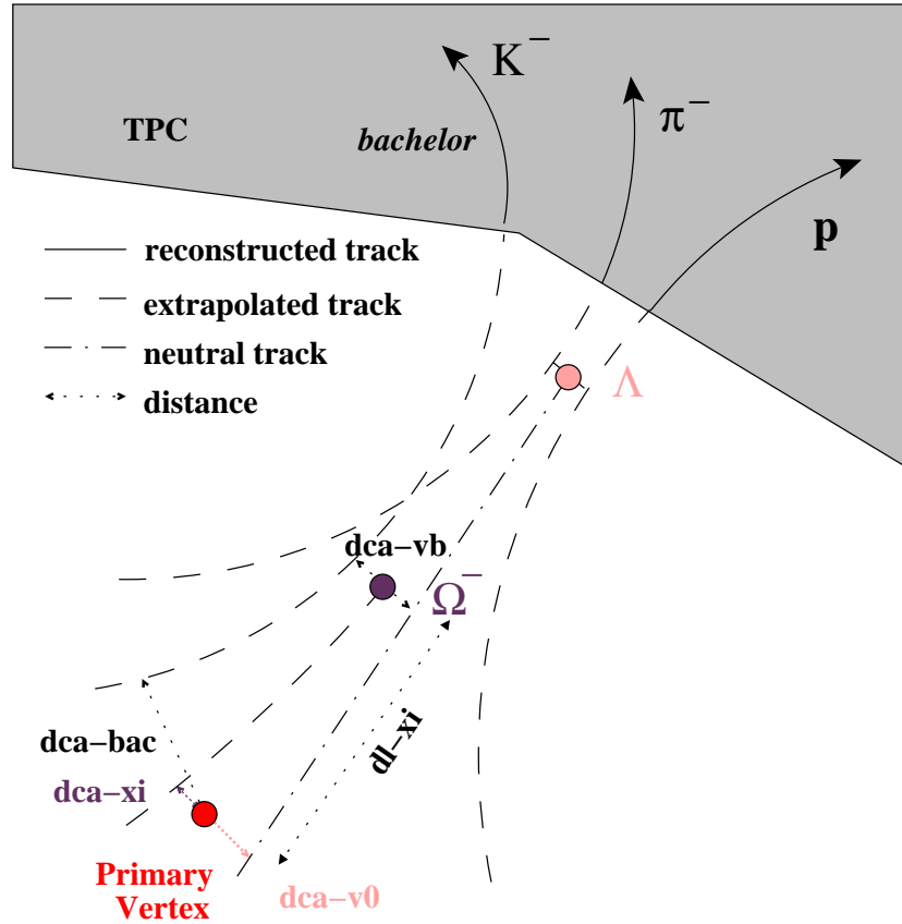
FIG. 3.6: Reconstruction des vertex de type "Xi": cas du \Omega .
