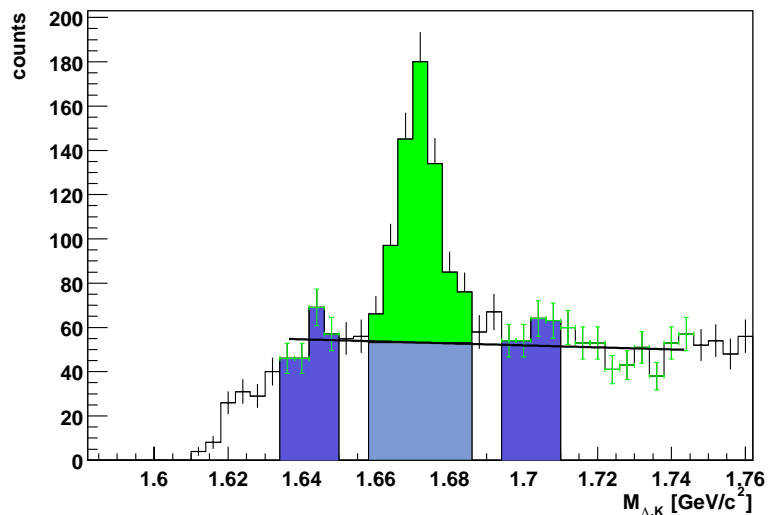
FIG. 5.18: Ajustement de la distribution en masse invariante en comptant le nombre d'entrées.
