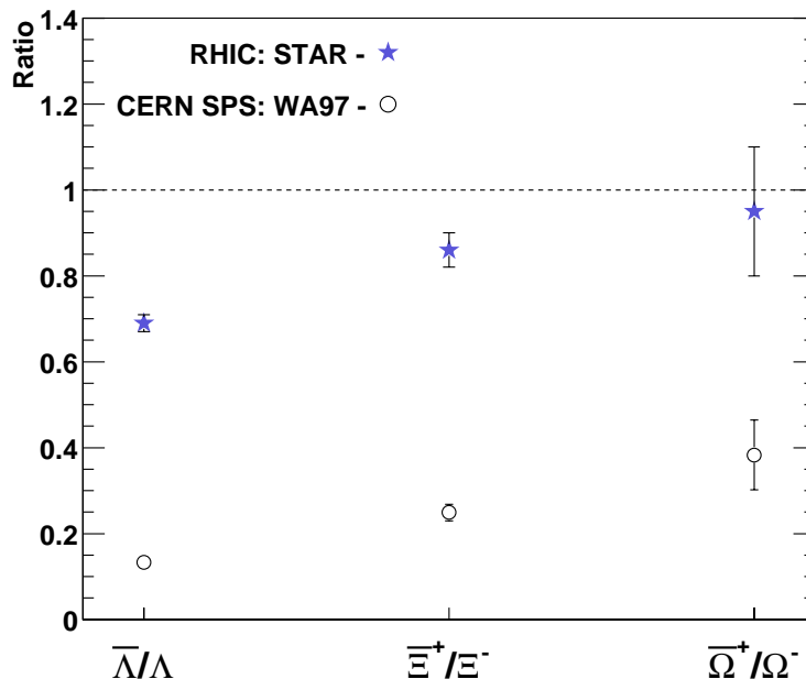
FIG. 6.1: Rapports anti-baryon / baryon étrange. Les étoiles correspondent aux mesures effectuées par STAR pour les collisions Au-Au à \sqrt{s_{NN}} = 130 GeV tandis que les cercles ouverts ont été rapportés par l'expérience WA97 à \sqrt{s_{NN}} = 17,4 GeV.
