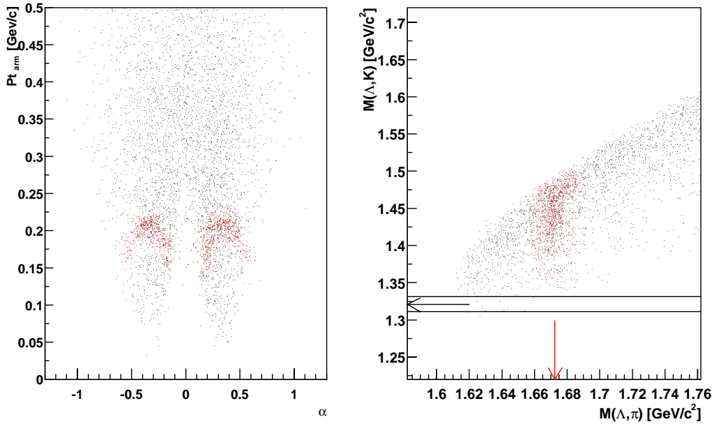
FIG. 5.15: Espace des phases des \Omega en représentation d'Armenteros-Podolanski (à gauche) et représentation des candidats \Omega selon les deux hypothèses de masse (à droite).
