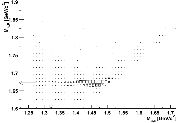
FIG. A.2: Représentation de particules \Omega simulées en fonction des deux hypothèses de masse. Les flèches indiquent les masses effectives des particules \Xi et \Omega . La dispersion et les limites cinématiques sont liées respectivement à la résolution et à l'acceptance du détecteur.
