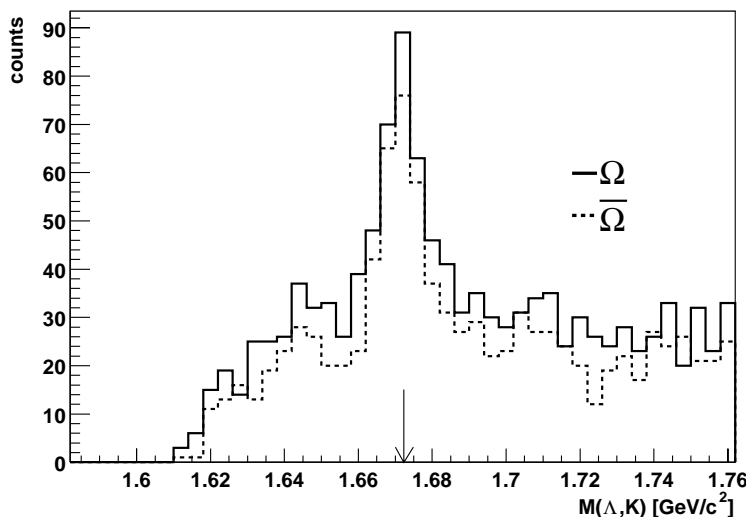
FIG. 5.22: Distribution en masse invariante des \Omega^- (trait plein) et des \bar{\Omega}^+ (pointillés), dans le cas d'une sélection en centralité de 11 % et |y| < 1.0 .
