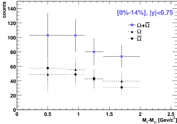
FIG. 5.20: Nombre de particules reconstruites dans les intervalles en (M_t - M_\Omega) pour 14 % des événements les plus centraux et |y| < 0.75 .
