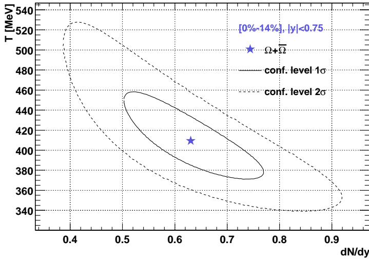
FIG. 5.25: Intervalles de confiance à 1\sigma et (en trait plein) 2\sigma (en pointillé) pour les valeurs du taux de production et de la température relative aux \Omega^- + \bar{\Omega}^+ .
