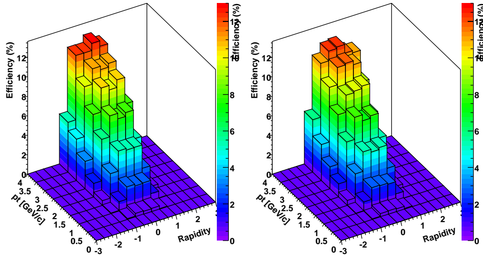
FIG. 4.11: Efficacité de reconstruction des \Omega^- (à gauche) et des \bar{\Omega}^+ (à droite) dans la TPC de STAR.
