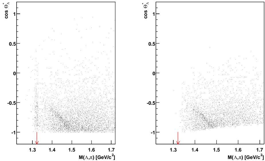
FIG. 5.13: Effet de la sélection en \cos \Theta^* du \Lambda des mêmes candidats \Omega que pour la figure 5.12 mais selon l'hypothèse de la reconstruction d'un \Xi . La figure de gauche correspond à l'espace cinématique sans la sélection tandis que l'effet de la sélection peut être vu sur la figure de droite.
