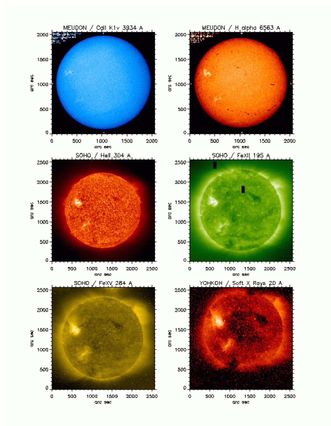
Figure 1.6 – Observation multi-spectrale du Soleil le 9 mars 1997, obtenue par le spectrohéliographe de Meudon (CaII K 1 \gamma et H \alpha ), SoHO/EIT (canaux à 304, 195, et 284 Å) et YOHKOH/SXT (20 Å). Le nord est en haut, l'est est à gauche.
