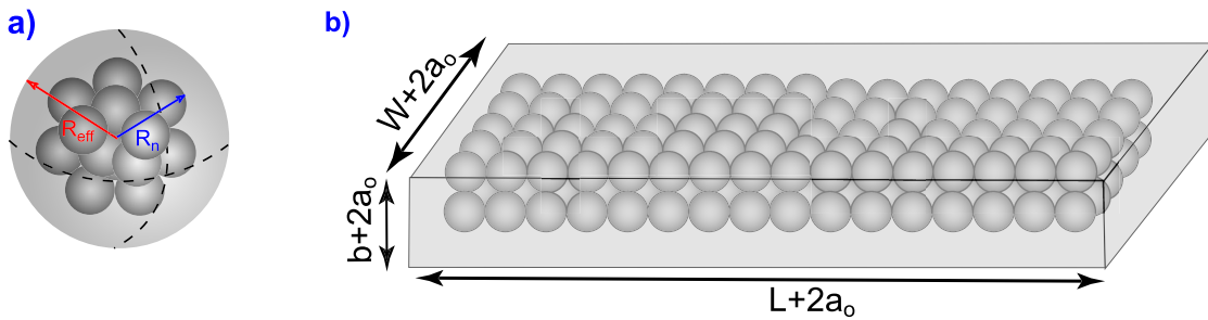
FIG. 4.4 – Schéma de principe illustrant le calcul du rayon de capture efficace a) pour les petits agglomérats et b) pour les défauts \{311\} de dimension L \times W \times b .
