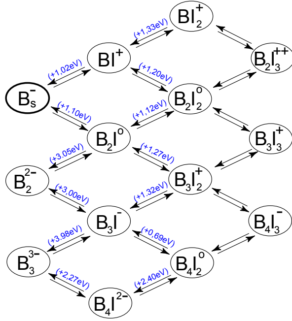
FIG. 4.6 – Schéma de principe illustrant les différents chemins possibles pour la formation d'agglomérats mixtes de bore et d'interstitiels. Les états de charge et les valeurs entre parenthèses des énergies mises en jeu lors des réactions sont issus des estimations de Lenosky et al. [LENO00].
