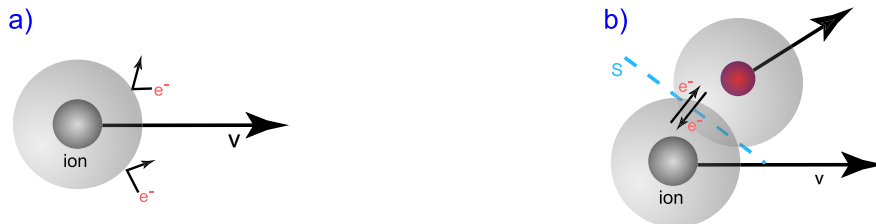
FIG. 3.3 – Illustration schématique du a) pouvoir non-local d'arrêt électronique et b) du pouvoir local d'arrêt électronique. (d'après [CHAK02])
