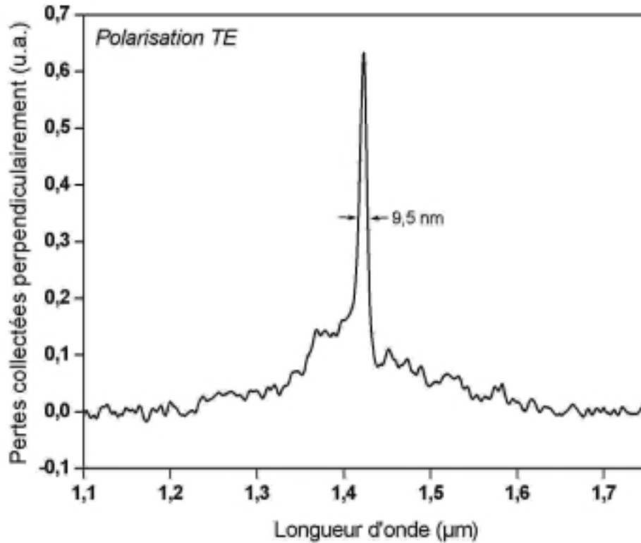
Figure 2-15 : Spectre lumineux collecté sur la cavité avec des miroirs à 6 rangées de trous, hors du plan, perpendiculairement à celui-ci, dans un cône de demi-angle au sommet 24^\circ lorsque de la lumière polarisée TE est injectée dans le guide (résolution 5 nm).
