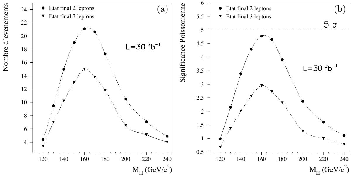
FIG. 6.18 – (a) Variation du nombre d'événements de signal en fonction de la masse du boson de Higgs. (b) Significances statistiques (calculée selon une distribution de Poisson) attendue en fonction de la masse du boson de Higgs. Les distributions sont normalisées pour une luminosité de 30 \text{ fb}^{-1} .
