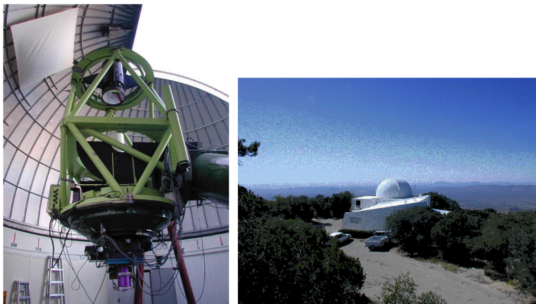
Figura 2.1: Il telescopio McGraw-Hill e il sito delle osservazioni.
