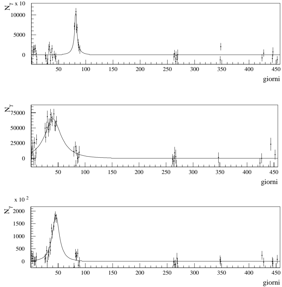
Figura 3.17: Esempi di curve di luce simulate
