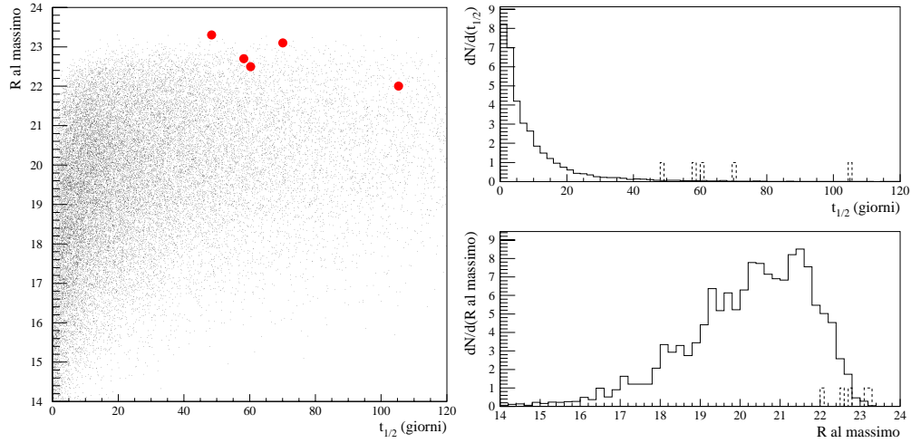
Figura 4.25: Le curve di luce selezionate nello spazio dei parametri t_{1/2}, R_{max} , caso con m_{alone}^{MACHO} = 0.01 M_{\odot} . Le unità sull'asse verticale delle distribuzioni (a destra) sono arbitrarie.
