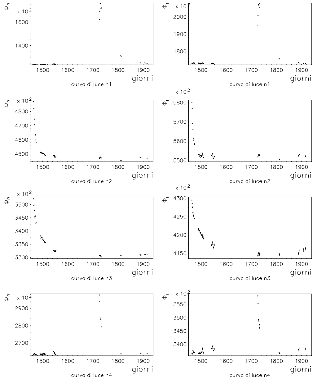
Figura 4.2: 4 curve di luce attribuibili a delle novae . In ascissa, il tempo espresso in giorni (J-2449624.5), in ordinate il flusso espresso in ADU.
