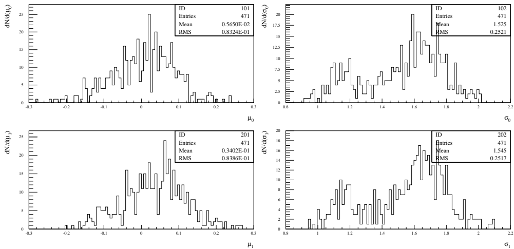
Figura 2.21: Distribuzioni per il valor medio, a sinistra, e la dispersione della (2.17), in basso i risultati ottenuti con il nuovo approccio di correzione.
