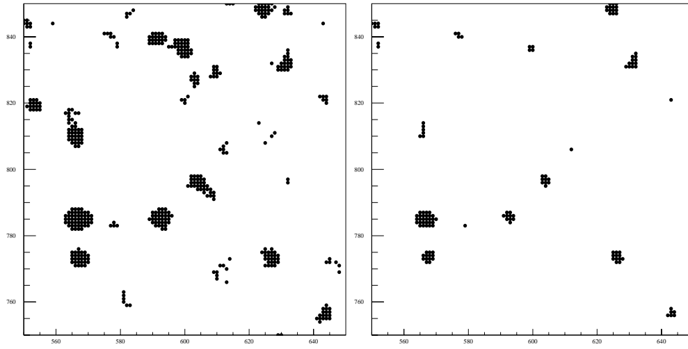
Figura 4.11: Esempio di clusters . In una regione di 100 \times 100 pixel, sono evidenziati in nero i pixel rappresentativi delle corrispondenti curve di luce dove risulta, con L_2/L_1 < 0.1 , L_1 > 100 (a sinistra) e L_1 > 300 . Dove a un valore elevato di L corrisponde solo una fluttuazione statistica, il cluster corrispondente tende a scomparire aumentando il valore di soglia della selezione.
