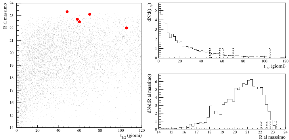
Figura 4.26: Le curve di luce selezionate nello spazio dei parametri t_{1/2}, R_{max} , caso con m_{alone}^{MACHO} = 0.5 M_{\odot} . Le unità sull'asse verticale delle distribuzioni (a destra) sono arbitrarie.
