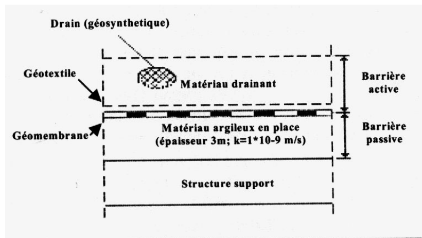
Figure I.9. Exemple type de structure de fond d'un CSD, classe II, avec son dispositif d'étanchéité-drainage
