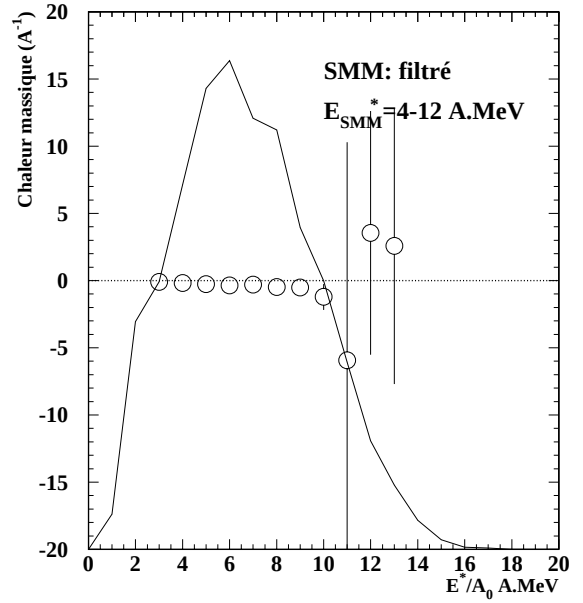
Figure VI.4: SMM: évolution de la chaleur massique totale C_t , points blancs, en fonction de l'énergie d'excitation par nucléon E^*/A_0 , pour un mélange de neuf "sources" de multifragmentation statistique SMM, filtrées par le dispositif expérimental, à des énergies d' E_{SMM}^* différentes entre 4 et 12 A.MeV par pas de 1 A.MeV. Les histogrammes représentent la distribution d' E^*/A_0 évaluée par calorimétrie.
