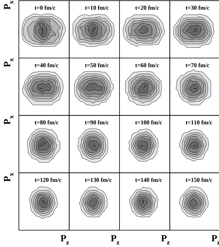
Figure IV.25: Evolution des contours de densité dans l'espace des impulsions pour un calcul BNV Xe + Sn à 32 A.MeV à b=0 fm. L'axe z correspond à l'axe du faisceau.
