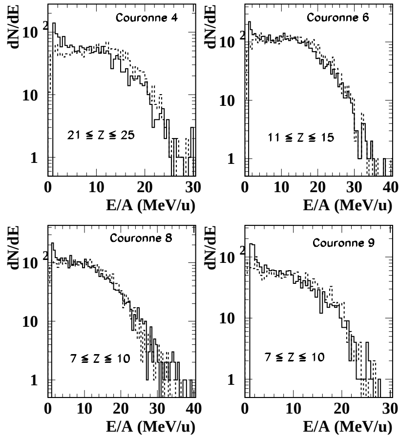
Figure II.8: Comparaison des spectres en énergie CsI par nucléon obtenus d'une part grâce à la calibration du Si( 300\mu m ) (trait pointillé) et d'autre part avec la conversion quantité de lumière-énergie (trait plein).
