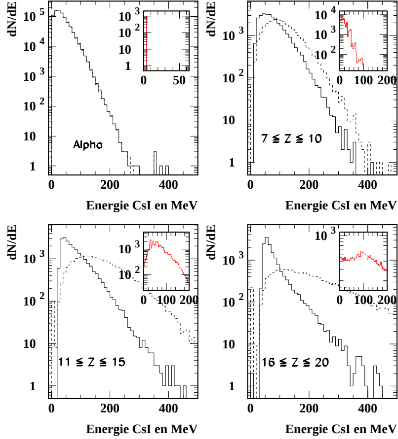
Figure II.14: Comparaison des spectres en énergie CsI, dans la couronne 11 pour la réaction ^{155}_{64}\text{Gd} + ^{238}_{92}\text{U} à 36 \text{ MeV/u} , pour différentes classes de fragments. Le trait plein correspond à la nouvelle calibration en énergie, qui tient compte des électrons \delta et le trait pointillé à l'ancienne. les spectres en haut à droite de chaque figure représentent la différence entre les deux méthodes pour chaque ion ou groupe d'ions.
