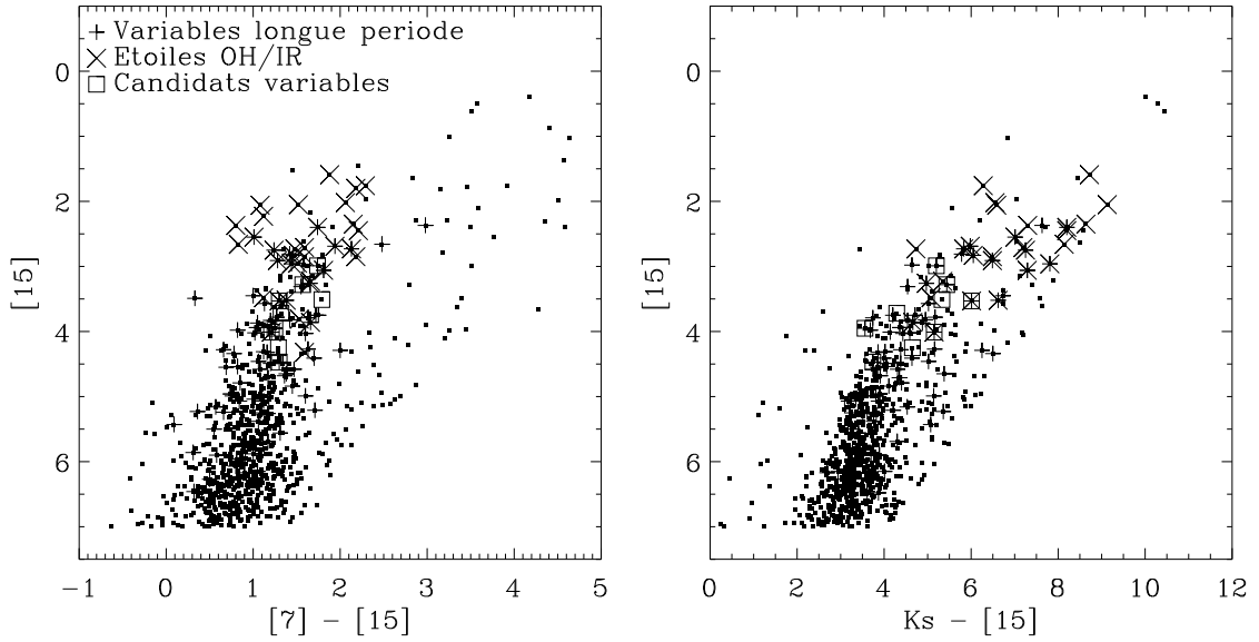
FIG. 3.7: Diagrammes magnitude couleur [15] / [7]-[15] (gauche) et [15] / K_s-[15] (droite) de toutes les sources du champ FC-00027-00006. Les sources associées à des étoiles variables et à des OH/IR sont indiquées par différents symboles.
