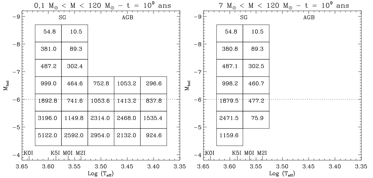
FIG. 3.26: Nombre d'étoiles par unité de SFR ( M_{\odot}/\text{an} ) et par intervalle de M_{bol} et \log(T_{eff}) après 10^9 ans de formation stellaire, pour une IMF de Salpeter normalisée entre 0,1 et 120 M_{\odot} (gauche) ou entre 7 et 120 M_{\odot} (droite), d'après les modèles de Padoue. La ligne pointillée montre la limite M_{bol} = -6 que nous nous sommes fixée pour la présente étude. Les types spectraux des supergéantes sont indiqués en regard des températures (voir Table 3.11).
