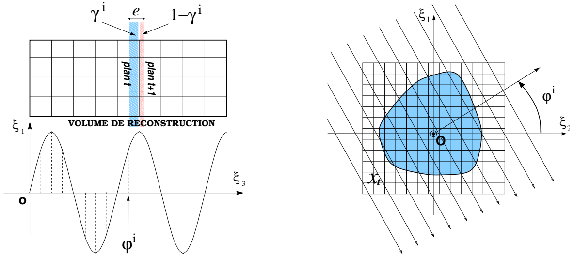
FIG. VIII.3: Projection en géométrie hélicoïdale dans le plan \xi_2 O \xi_3 ( \leftarrow ) et dans le plan \xi_1 O \xi_2 ( \rightarrow ).
