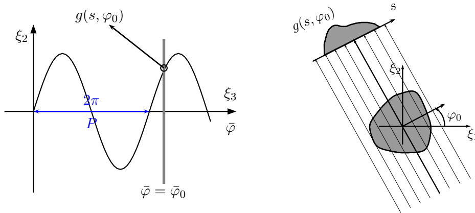
FIG. IV.2: Trajectoire de la source en mode hélicoïdal suivant l'axe du tomographe ( \leftarrow ), et dans le plan de l'image \xi_1 O \xi_2 associé à l'angle \bar{\varphi}_0 sur l'hélice ( \rightarrow ). Pour une position angulaire \bar{\varphi} = \bar{\varphi}_0 selon l'axe du tomographe, l'angle de projection dans le plan de l'image est \varphi_0 = \text{mod}_{2\pi}(\bar{\varphi}_0) .
