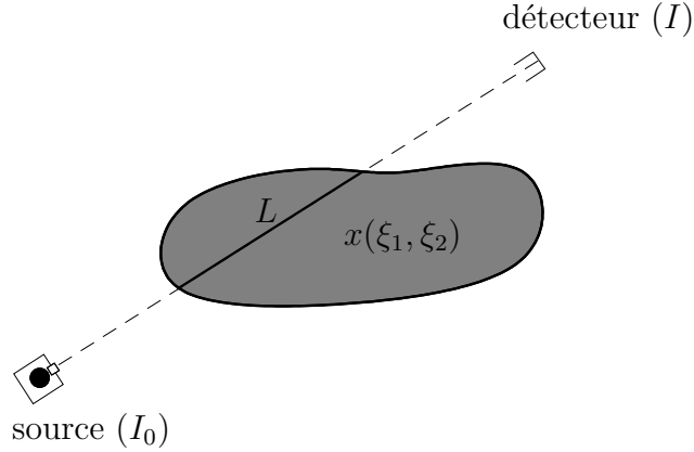
FIG. II.1: Transmission du faisceau X infiniment mince au travers d'une couche de matériaux
