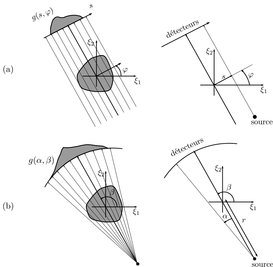
FIG. II.2: Géométrie d'acquisition en mode axial : (a) rayons parallèles ou (b) rayons divergents.
