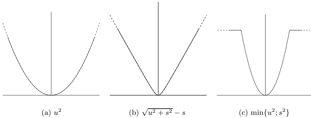
FIG. V.1: Exemples de fonctions coût proposées dans la littérature : (a) quadratique, (b) compromis convexe \ell_2\ell_1 , (c) non convexe \ell_2\ell_0 .
