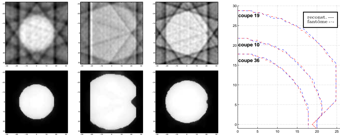
FIG. VIII.10: Reconstruction des coupes 36, 19 et 10 par LI-180° + RPC (haut) ou par approche pénalisée \ell_2\ell_1 (bas) et tracé des courbes segmentées à 0,7 pour le volume reconstruit par approche pénalisée. La RPC a été mise en œuvre avec un filtre de reconstruction de type cosinus et une fréquence de coupe réduite \nu_c = 0,3 ; les hyperparamètres de l'approche pénalisée ont été ajustés manuellement.
