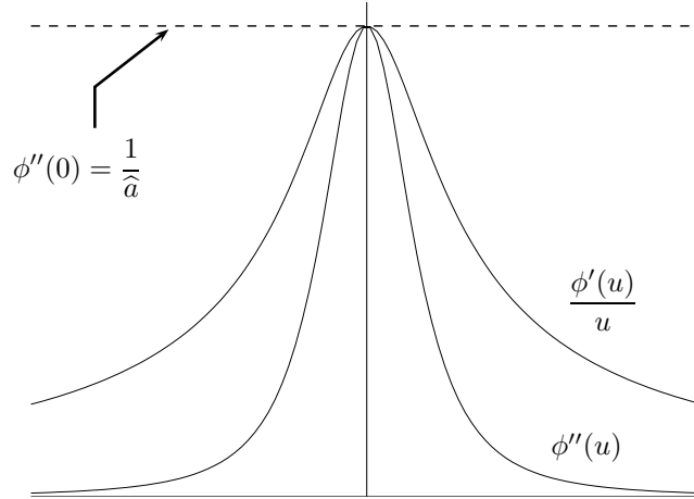
FIG. X.3: Tracé de \phi''(u) et de \phi'(u)/u pour \phi(u) = \sqrt{u^2 + s^2} ; on remarquera que le maximum de \phi'(u)/u est atteinte en zéro et qu'elle correspond à la courbure maximale de \phi .
