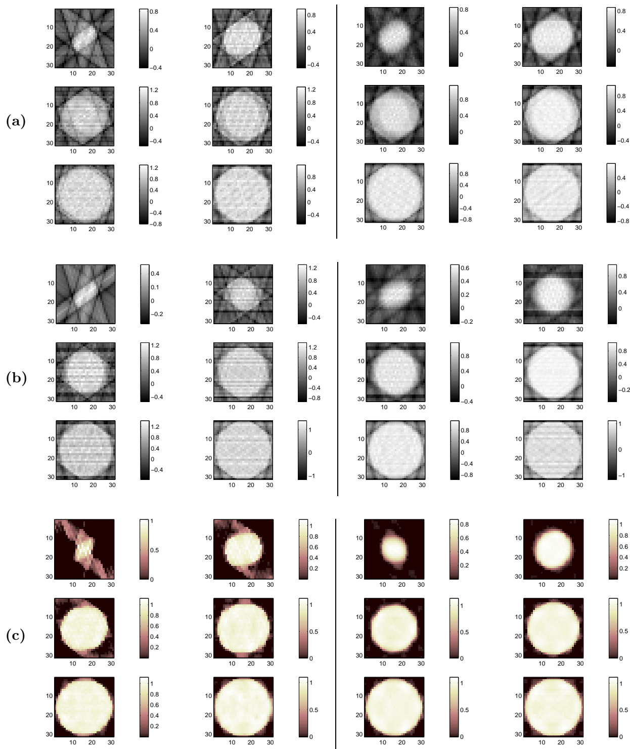
FIG. VIII.6: Reconstruction du fantôme de la figure VIII.4 pour un faisceau sans épaisseur (←) ou d'épaisseur égale au côté d'un voxel (→) : par RPC+LI-360° (a), RPC+LI-180° (b), approche pénalisée l_2l_1 (c). La RPC a été mise en œuvre avec un filtre de reconstruction de type HAMMING et une fréquence de coupure réduite \nu_c = 0,2 ; les hyperparamètres de l'approche pénalisée ont été ajustés manuellement.
