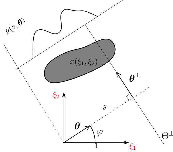
FIG. II.4: Illustration de la TR en dimension 2.
