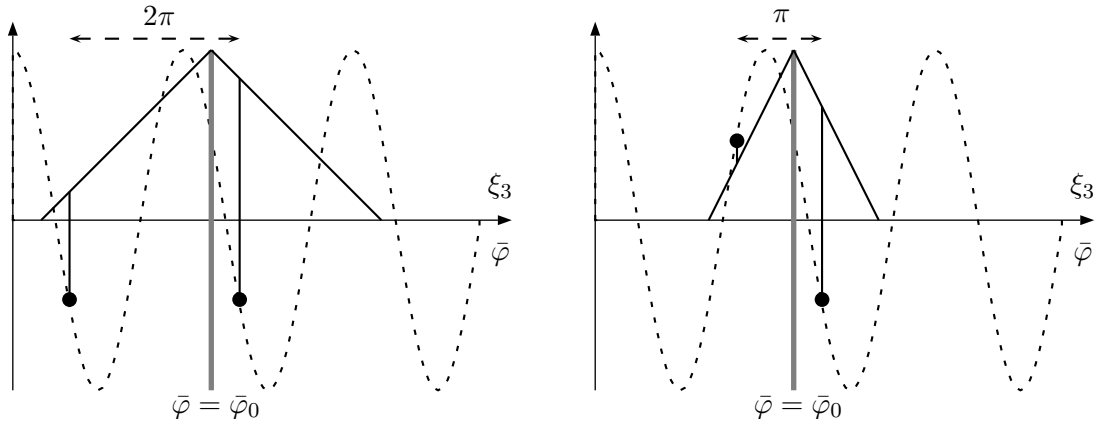
FIG. IV.3: Procédés usuels d'interpolation adoptés pour recréer un jeu « axial consistant » dans le plan défini par \bar{\varphi} = \bar{\varphi}_0 . Chaque pseudo projection axiale d'angle \varphi découle de deux projections obtenues dans les plans \bar{\varphi}_0 + \Delta\varphi et \bar{\varphi}_0 - 2\pi + \Delta\varphi pour le mode « full-scan » ( \leftarrow ), ou \bar{\varphi}_0 + \Delta\varphi et \bar{\varphi}_0 - \pi + \Delta\varphi pour le mode « half-scan » ( \rightarrow ); \Delta\varphi = \varphi - \text{mod}_{2\pi}(\bar{\varphi}_0) .
