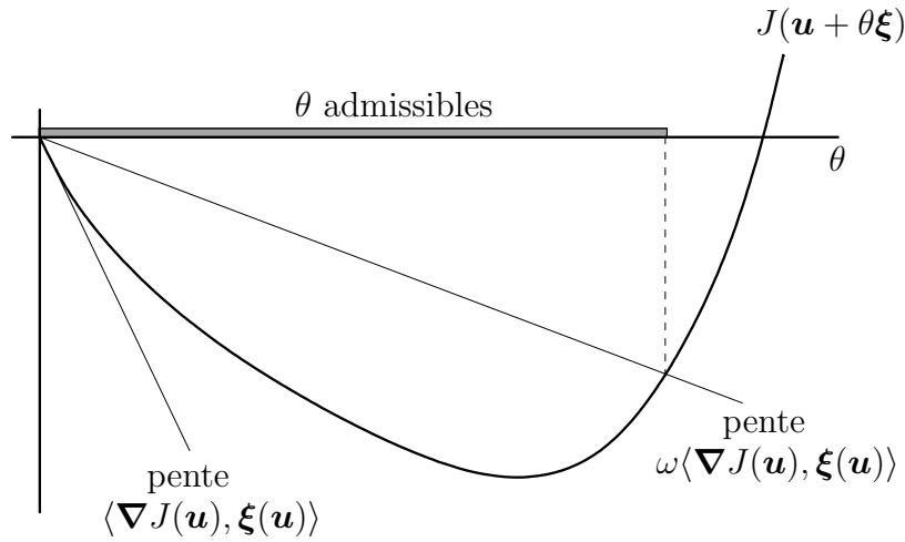
FIG. X.1: Illustration de la règle d'ARMIJO.
