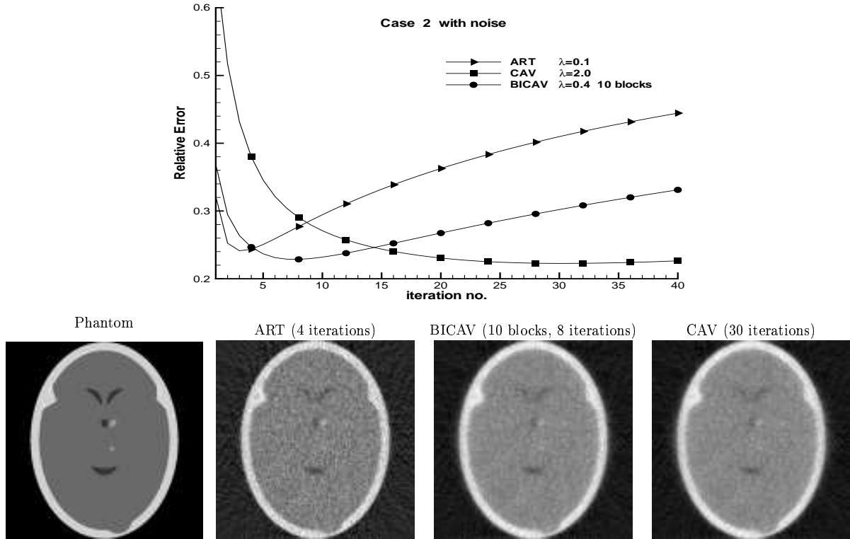
FIG. III.3: Mise en œuvre extraite de [Censor et al. , 2001] des algorithmes ART, BICAV et CAV sur données bruitées ; (haut) : évolution de l'erreur relative mesurée sur la reconstruction du fantôme ; bas : fantôme synthétique utilisé, et meilleures reconstructions obtenues pour les trois algorithmes.
