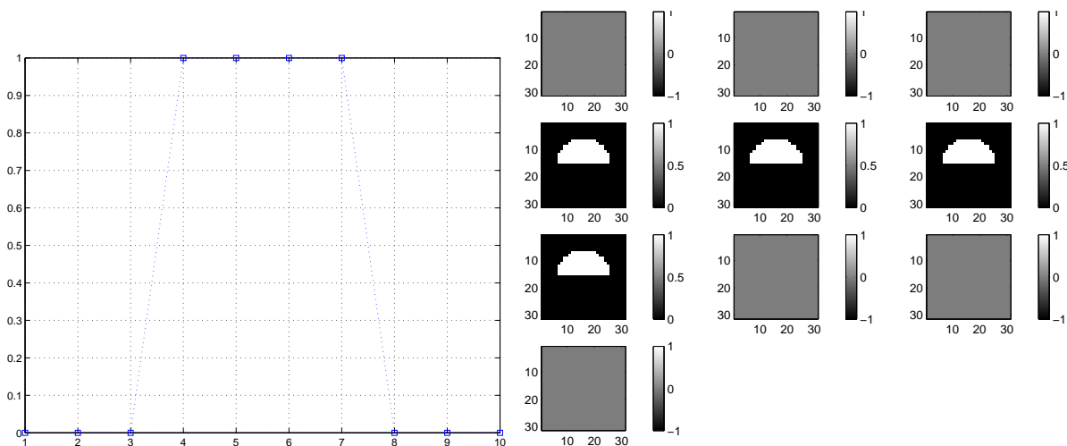
FIG. VIII.5: Fantôme synthétique utilisé pour l'estimation de la SSP ( \leftarrow ) ; plans de reconstruction du fantôme choisis ( \uparrow ) et énergie normalisée contenue dans chacun des plans du fantôme destinés à être reconstruit.
