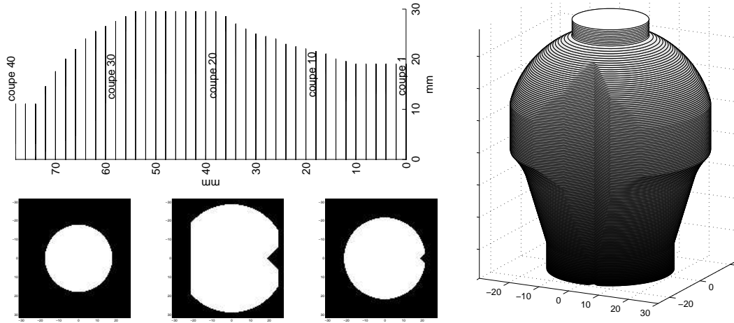
FIG. VIII.9: Fantôme 3D de grande taille : ( \rightarrow ) vue en perspective, ( \leftarrow haut) variation du profile suivant l'axe du tomographe, ( \leftarrow bas) coupes 10, 19 et 36 extraite du fantôme.
