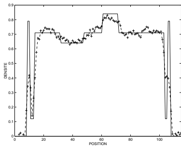
FIG. VII.4: Cas ③ : reconstructions par RPC du fantôme à un niveau de perturbation « limite » pour la robustesse de la méthode (bruit additif gaussien décorrélé, centré et d'écart type \sigma = 0,008 ).
