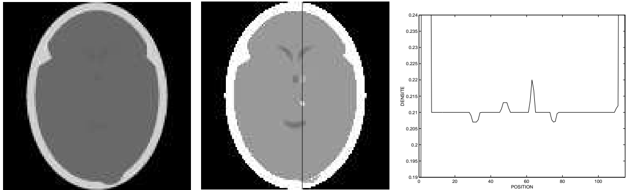
FIG. VII.6: Cas ③ : limite de robustesse au bruit de la reconstruction pénalisée (bruit additif décorrélé, gaussien centré d'écart type \sigma = 0,01 ) ; cas ④ test de robustesse à une excursion angulaire incomplète : 151 projections produites uniformément dans [0; 5\pi/6[ perturbées par un bruit additif décorrélé, gaussien centré d'écart type \sigma = 0,001 . La colonne de gauche illustre les performances de la RPC (filtre de Hamming, \nu_c = 0,8 ), celle de droite illustre celles de l'approche pénalisée (modèle l_2l_1 , \alpha = 2,5 \cdot 10^{-3} ; s = 8 \cdot 10^{-5} ).
