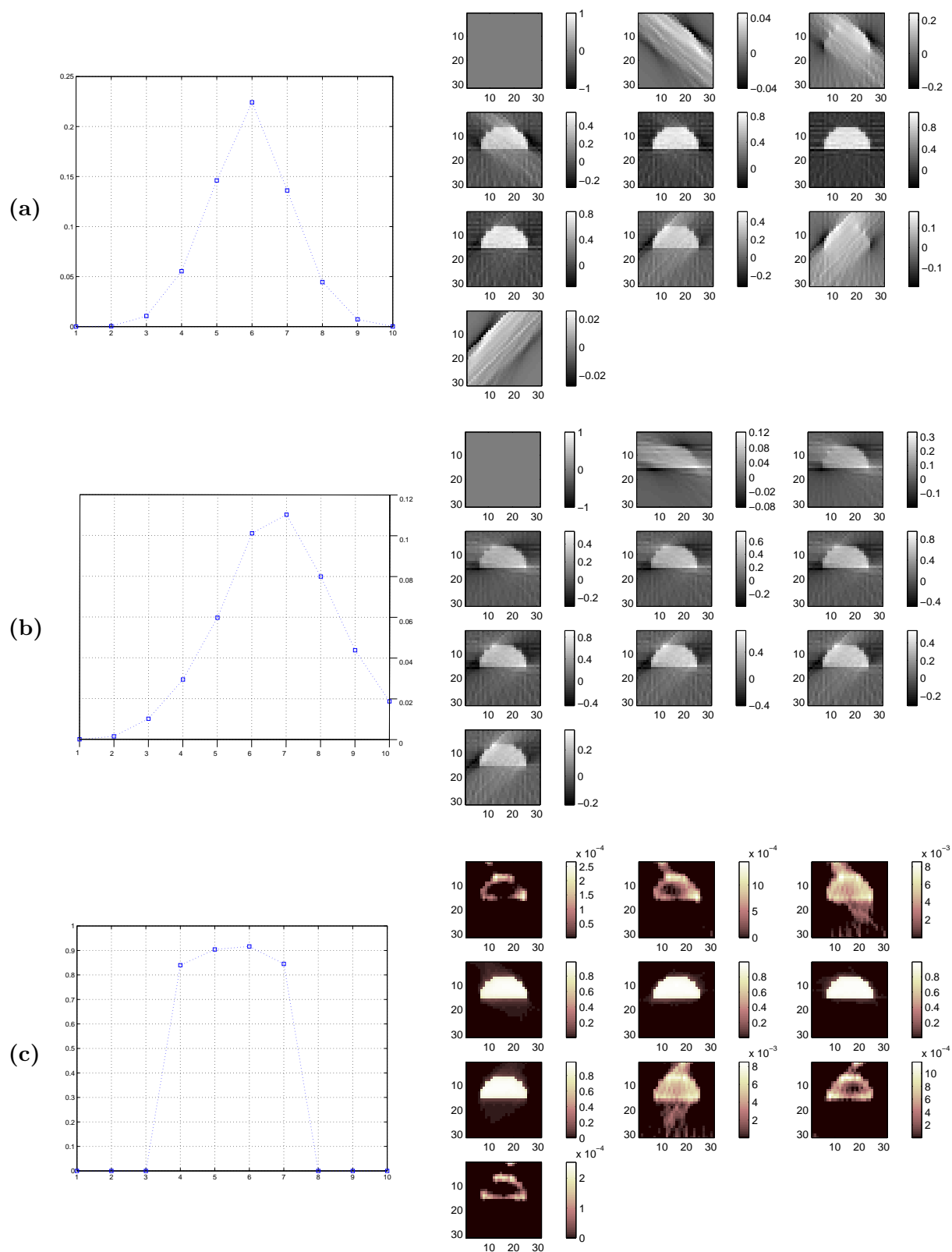
FIG. VIII.8: Tracés des SSP pour des données non bruitées et un faisceau d'épaisseur nulle : RPC+LI-180° (a), RPC+LI-360° (b), ou approche pénalisée l_2l_1 (c).
