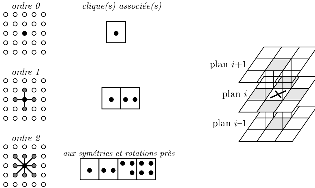
FIG. VI.1: Voisinages d'ordre zéro, un et deux dans le plan avec les cliques associées ( \leftarrow ); voisinage du premier ordre en 3D ( \rightarrow ); cette figure est reproduite avec l'aimable autorisation de Nicolas Villain.
