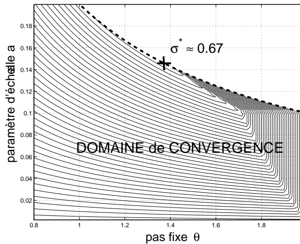
FIG. X.5: Courbes de niveaux pour \sigma_{\text{GY}}(\theta, a) à l'intérieur du nouveau domaine de convergence défini par \theta \in ]0; 2[ et a \in ]2\hat{a}/\theta[ pour \hat{a} = 0,1 ; le meilleur taux de convergence noté \sigma^* est atteint sur la frontière.
