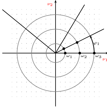
FIG. III.1: Échantillonnage radiale de la TF de x .
