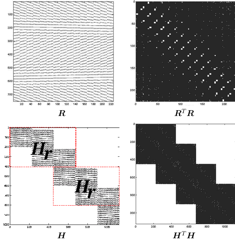
FIG. VIII.13: Opérateur d'observation et matrice Q obtenue en géométrie axiale (haut) et en géométrie hélicoïdale (bas) sur un problème de petite taille ( 15 \times 15 pixels en axial et 5 plans de 15 \times 15 voxels en hélicoïdal); dans H , l'opérateur H_r a été délimité par des pointillés afin de simplifier l'interprétation de sa structure.
