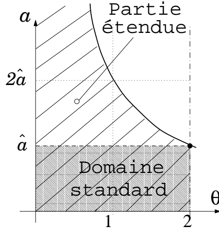
FIG. X.2: Domaines de convergence découlant de l'étude de convexité du critère primal/dual (domaine standard en gris) et de l'admissibilité du pas fixe pour la règle d'ARMIJO (domaine étendu achuré).
