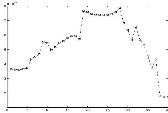
FIG. VIII.11: Tracé de l'EQM dans chaque tranche pour la reconstruction exacte.
