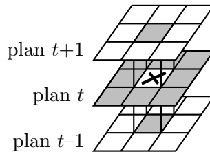
FIG. VIII.2: Système de voisinage 3D retenu : le voxel courant (croix) interagit avec 8 voisins dans le plan de l'image et 2 voisins dans l'axe du tomographe.
