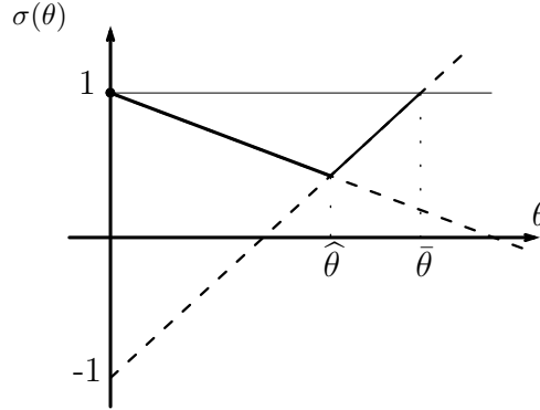
FIG. X.4: Évolution du rayon spectral \sigma(\theta, \mathbf{u}) en fonction du pas fixe \theta .
