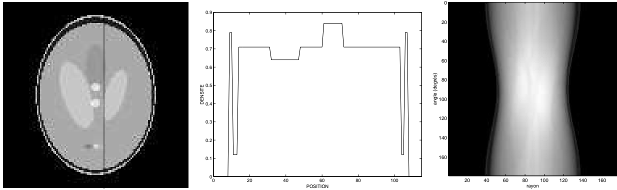
FIG. VII.2: Fantôme de SHEPP et LOGAN utilisé pour les mises en œuvre ( \leftarrow ); tracé de la 63-ème colonne de ce fantôme ( \uparrow ); Sinogrammes composé de 151 projections échantillonnées sur 175 rayons obtenu pour un faisceau d'épaisseur nulle et sans bruit d'observation ( \rightarrow ).
