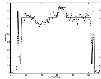
FIG. VII.4: Cas ③ : reconstructions par RPC du fantôme à un niveau de perturbation « limite » pour la robustesse de la méthode (bruit additif gaussien décorrélé, centré et d'écart type \sigma = 0,008 ).
