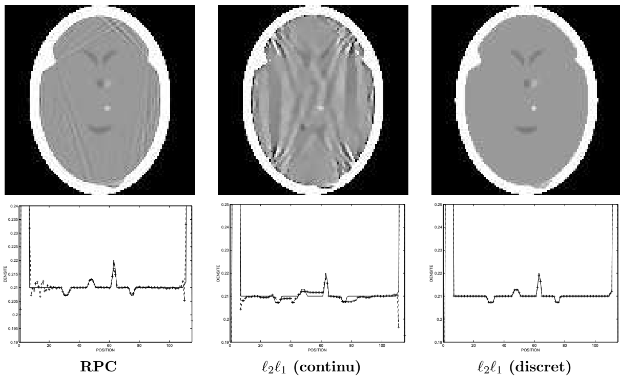
FIG. VII.8: Cas ① : reconstruction du fantôme de la figure VII.7 par RPC ( \leftarrow ), par approche pénalisée à partir des mêmes projections ( \uparrow ) et pour des projections produites pour le fantôme pixelisé.
