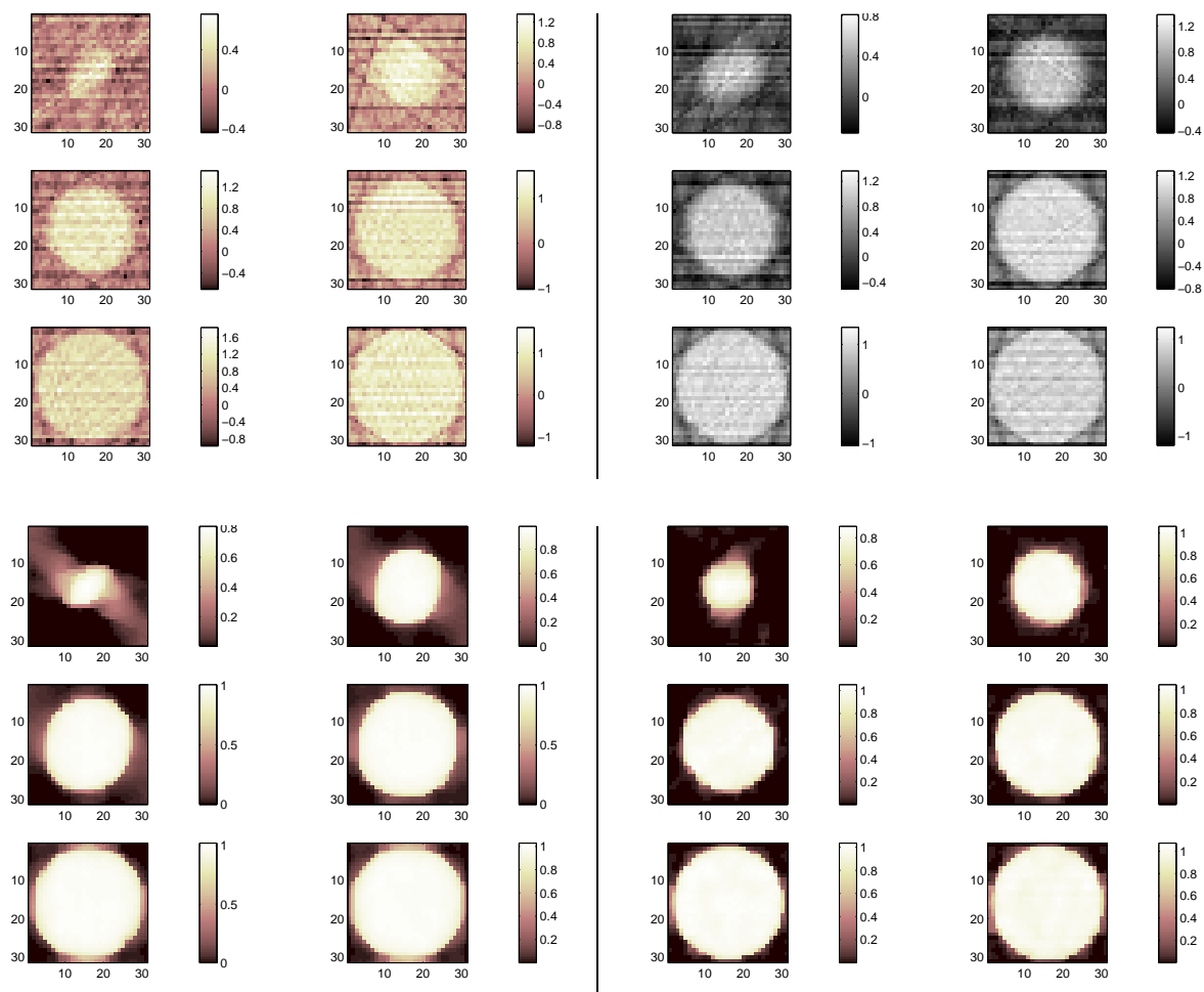
FIG. VIII.7: Reconstruction du fantôme VIII.4 pour des données bruitées ( \sigma = 1 ) et une épaisseur de faisceau nulle ( \leftarrow ) ou égale à la largeur d'un plan de voxels ( \rightarrow ) : RPC+LI-180° (haut) ou approche pénalisée \ell_2\ell_1 (bas). La RPC a été mise en œuvre avec un filtre de reconstruction de type HAMMING et une fréquence de coupure réduite \nu_c = 0, 2 .
