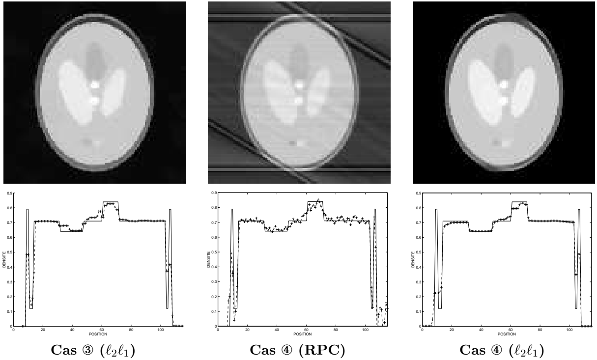
FIG. VII.6: Cas ③ : limite de robustesse au bruit de la reconstruction pénalisée (bruit additif décorrélé, gaussien centré d'écart type \sigma = 0,01 ) ; cas ④ test de robustesse à une excursion angulaire incomplète : 151 projections produites uniformément dans [0; 5\pi/6[ perturbées par un bruit additif décorrélé, gaussien centré d'écart type \sigma = 0,001 . La colonne de gauche illustre les performances de la RPC (filtre de Hamming, \nu_c = 0,8 ), celle de droite illustre celles de l'approche pénalisée (modèle l_2l_1 , \alpha = 2,5 \cdot 10^{-3} ; s = 8 \cdot 10^{-5} ).
