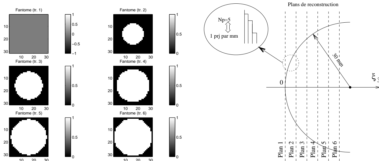
FIG. VIII.4: Fantôme utilisé pour créer le jeux de projections hélicoïdales (haut) ; plans du fantôme choisis pour la reconstruction ( \leftarrow ) et emplacement par rapport au fantôme ( \rightarrow ).
