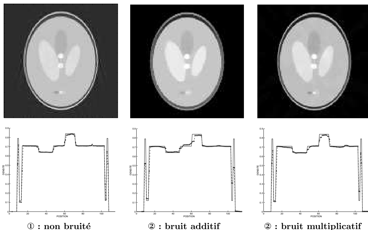
FIG. VII.5: Cas ① et ② : reconstruction par approche pénalisée du fantôme à partir de projections obtenues pour une épaisseur de faisceau nulle et sans bruit (①) ; une épaisseur de faisceau égale à la largeur d'un pixel et un bruit additif (②) ou multiplicatif (②). Les paramètres de régularisation \alpha et s ont été ajustés manuellement de manière à obtenir le meilleur compromis visuel entre la résolution et le niveau de bruit.
