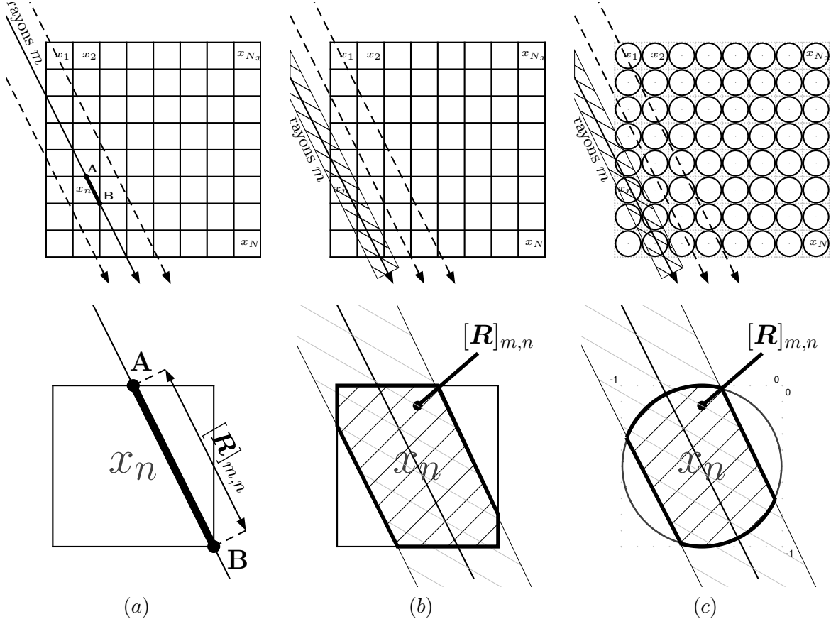
FIG. III.2: Calcul des éléments de \mathbf{R} pour un modèle à base d'indicatrices sur les pixels avec indexation lexicographique; (a) représente le cas d'un faisceau sans épaisseur avec des « pixels carrés », (b) le cas d'un faisceau de type « bande », et (c) le cas d'un faisceau de type « bande » avec des « pixels cylindriques ».
