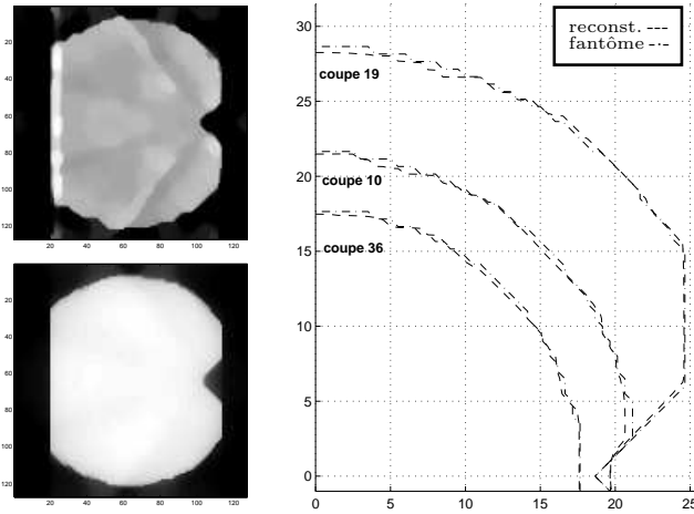
FIG. VIII.14: Reconstruction de la coupe 19 par approche pénalisée \ell_2\ell_1 après 70 itération de l'algorithme (—) pour une initialisation par RPC (haut) et par une image uniformément nulle (bas) ; tracés segmentés à 0,7 extraits des coupes 10, 19 et 36 obtenues après 70 itération pour l'initialisation par un vecteur nul.
