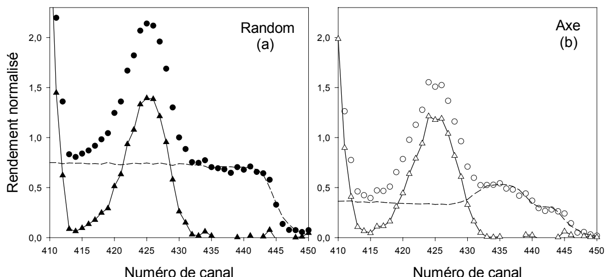
Figure 3 : Procédure utilisée pour l'analyse du pic de Cs dans un monocristal de zircon implanté (a) en direction aléatoire ; (b) selon l'axe \langle 100 \rangle . Les lignes pointillées représentent le signal de Hf à soustraire des pics de Cs (cercles). Les triangles donnent le résultat final.
