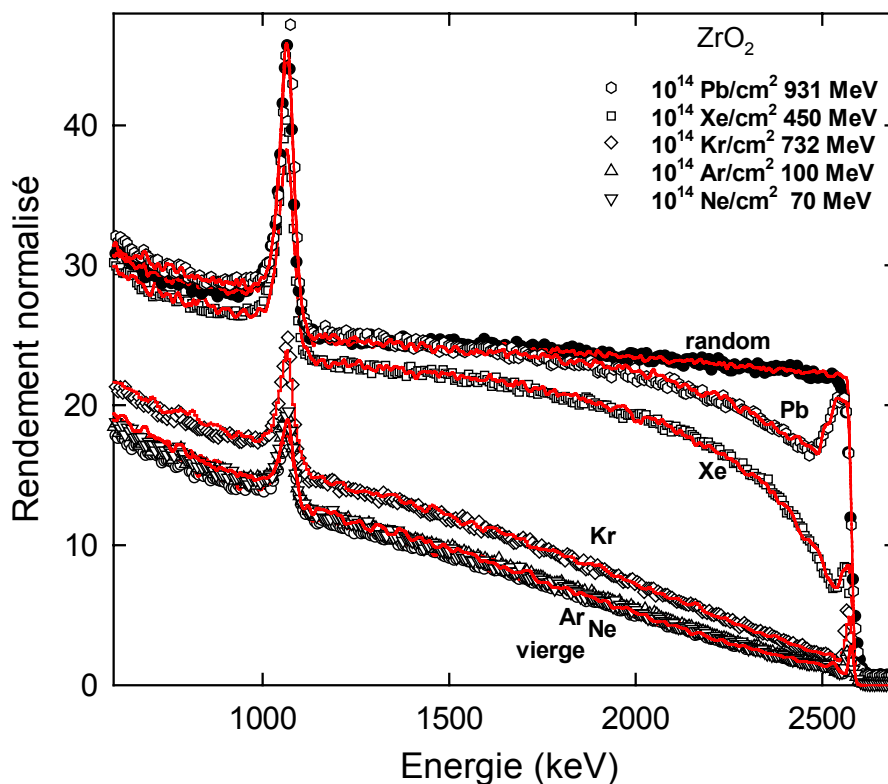
Figure 37 : Simulations numériques (lignes continues) des spectres RBS enregistrés sur les échantillons irradiés avec les différents ions à une fluence de 10^{14} \text{ cm}^{-2} (symboles fermés : direction aléatoire, symboles ouverts : axe \langle 100 \rangle ).
