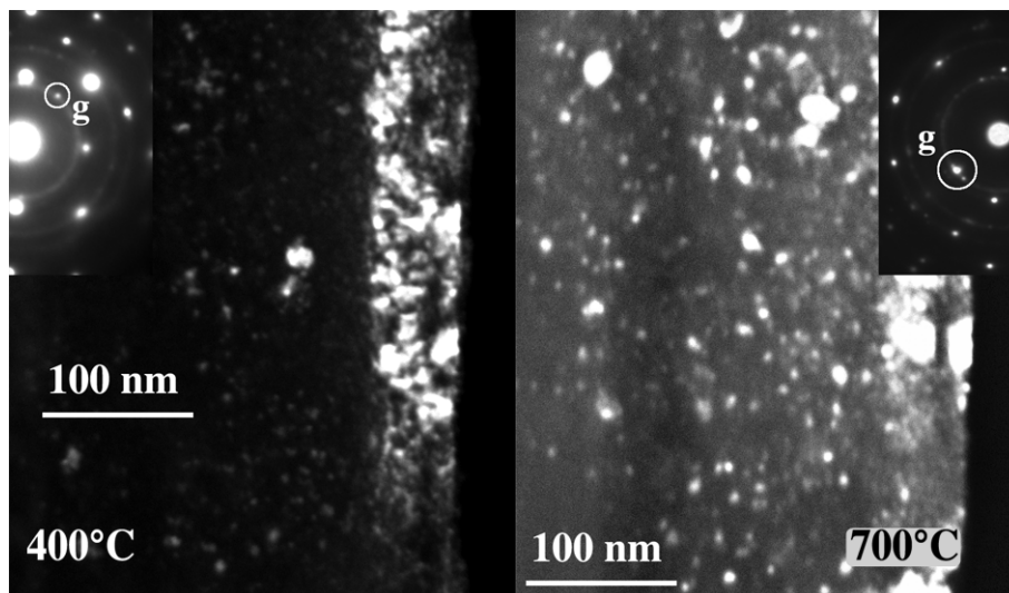
Figure 13 : Evolution de la recrystallisation d'un monocristal de zircone implanté avec des ions Cs à une fluence de 10^{16} \text{ cm}^{-2} en fonction de la température.
