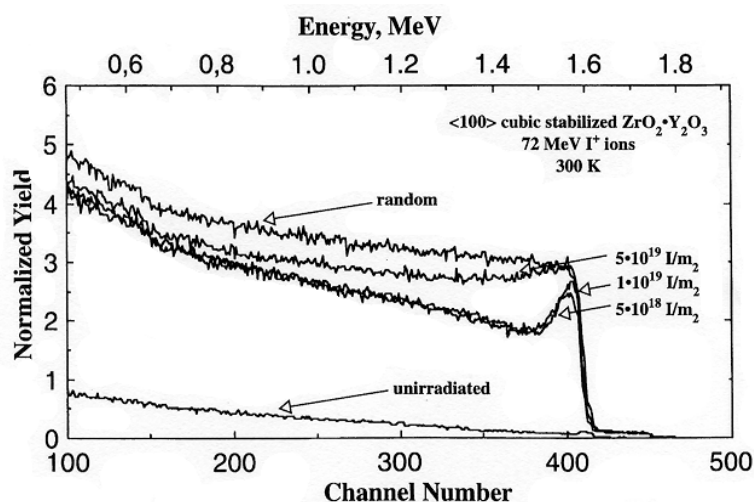
Figure 10 : Spectres RBS/C enregistrés sur un monocristal de zirconie irradié à température ambiante avec des ions I^+ de 72 MeV à trois fluences : 10^{14} , 10^{15} et 5 \times 10^{15} \text{ cm}^{-2} , d'après la référence [11].
