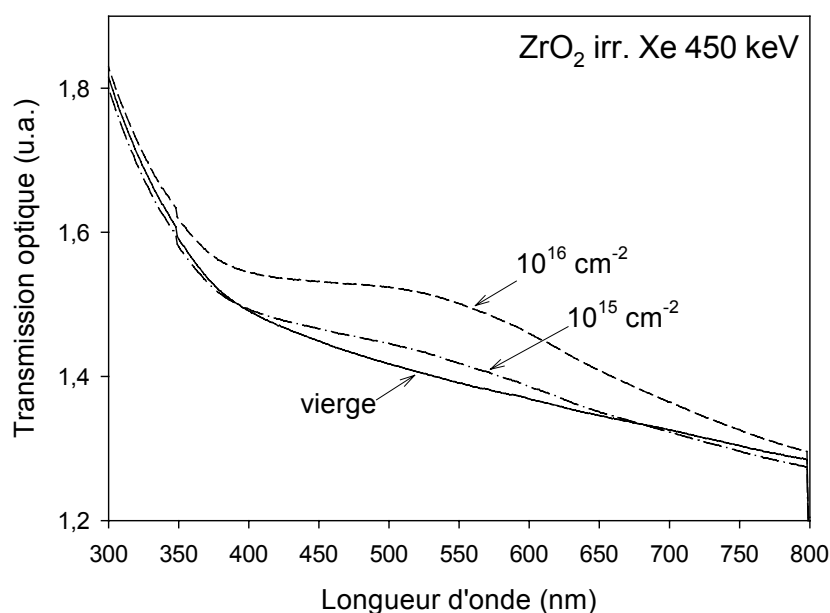
Figure 23 : Bandes d’absorption optique observées sur un monocristal de zircone irradié avec des ions Xe de 450 keV, aux fluences indiquées sur la figure.
