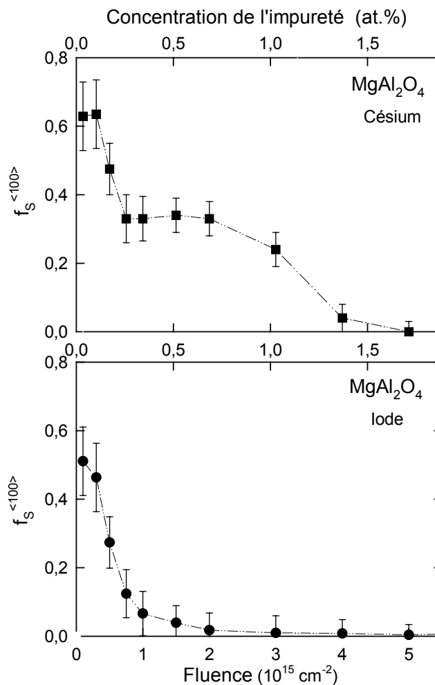
Figure 15 : Fraction substitutionnelle mesurée pour l'axe \langle 100 \rangle en fonction de la fluence (échelle du bas) ou de la concentration (échelle du haut) d'ions implantés.
