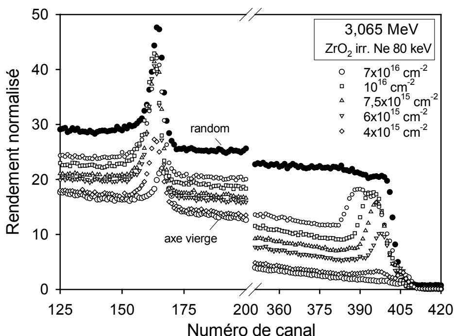
Figure 18 : Spectres RBS/C enregistrés à 3,065 MeV en directions aléatoire (symboles fermés) et alignée selon l’axe \langle 100 \rangle (symboles ouverts) dans la zircone irradiée avec différentes fluences d’ions Ne d’énergie 80 keV.
