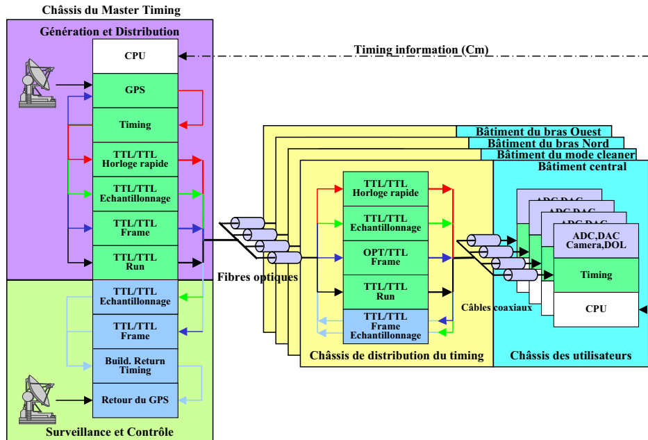
FIG. 3.1 – Organisation du système de synchronisation. (figure : Alain Masseur)
