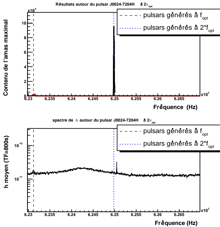
FIG. 7.18 – Moyenne des transformées de Fourier et résultat de l'analyse pour le pulsar J0024-7204H autour de 2 fois sa fréquence de rotation.
