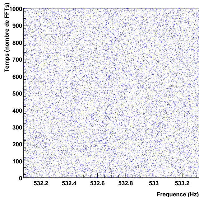
FIG. 6.4 – Diagramme temps-fréquence.
