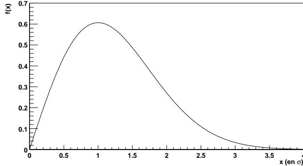
FIG. A.2 – Représentation graphique de f(x) .
