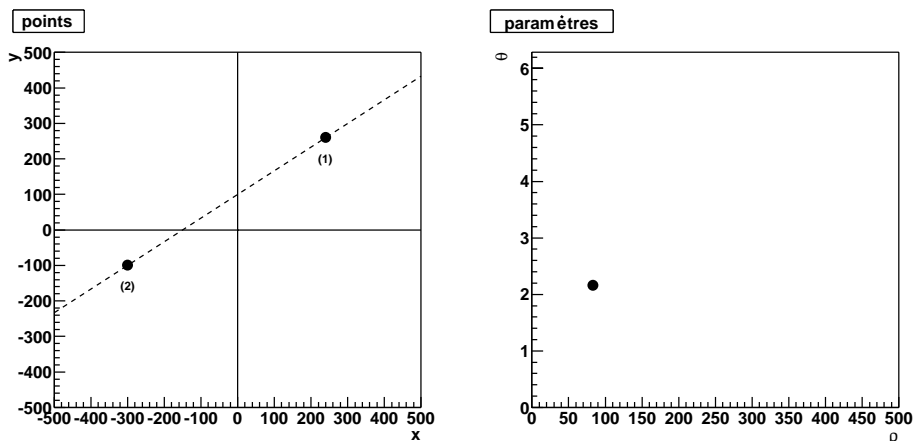
FIG. B.4 – Transformée de Hough à 2 points. La droite à laquelle appartiennent les 2 points est représentée par un point dans l'histogramme (\rho, \theta) .
