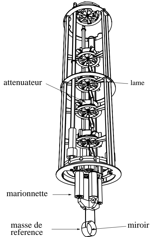
FIG. 2.3 – Super atténuateur de Virgo.
