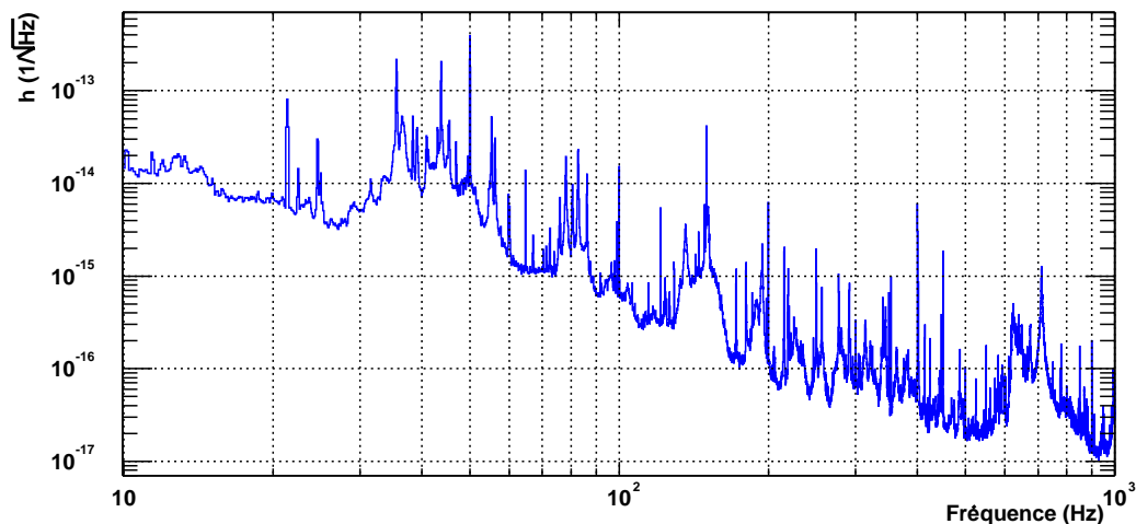
FIG. 7.6 – Courbe de sensibilité de Virgo pendant le run E4.
