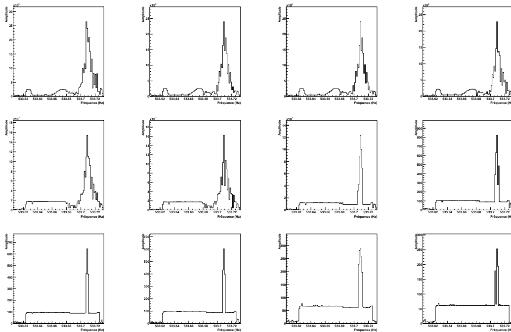
FIG. 7.13 – Résultats de l’algorithme sur des diagrammes temps-fréquence ne différant que par la hauteur de sélection des points. Le nombre de points gardé varie de 1.2‰ (en haut à gauche) à 1‰ (en bas à droite).
