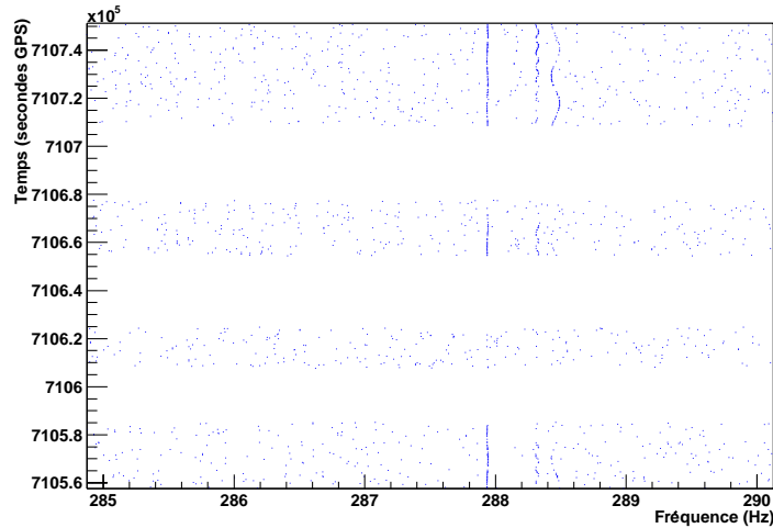
FIG. 7.7 – Un exemple de diagramme temps-fréquence où il a fallu trouver un compromis pour l'amplitude du signal, et où la variation du niveau de bruit avec le temps apparaît.
