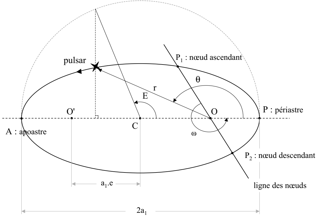
FIG. 5.1 – Éléments orbitaux d'un système binaire, dans le plan orbital.
