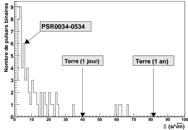
FIG. 6.2 – Valeur de \Xi = (1 - e).P_b/\sqrt{a_1}.\sin i pour les pulsars binaires détectés et valeur de T_o/\sqrt{R_o} pour la rotation de la Terre sur elle-même et sa révolution autour du Soleil.
