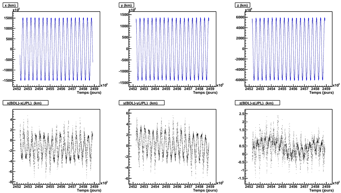
FIG. 5.6 – Superposition des composantes (x,y,z) de la position de la Terre par rapport au barycentre du Système Solaire en sortie des algorithmes du BDL et du JPL, pendant la période 2002-2020, et différences.
