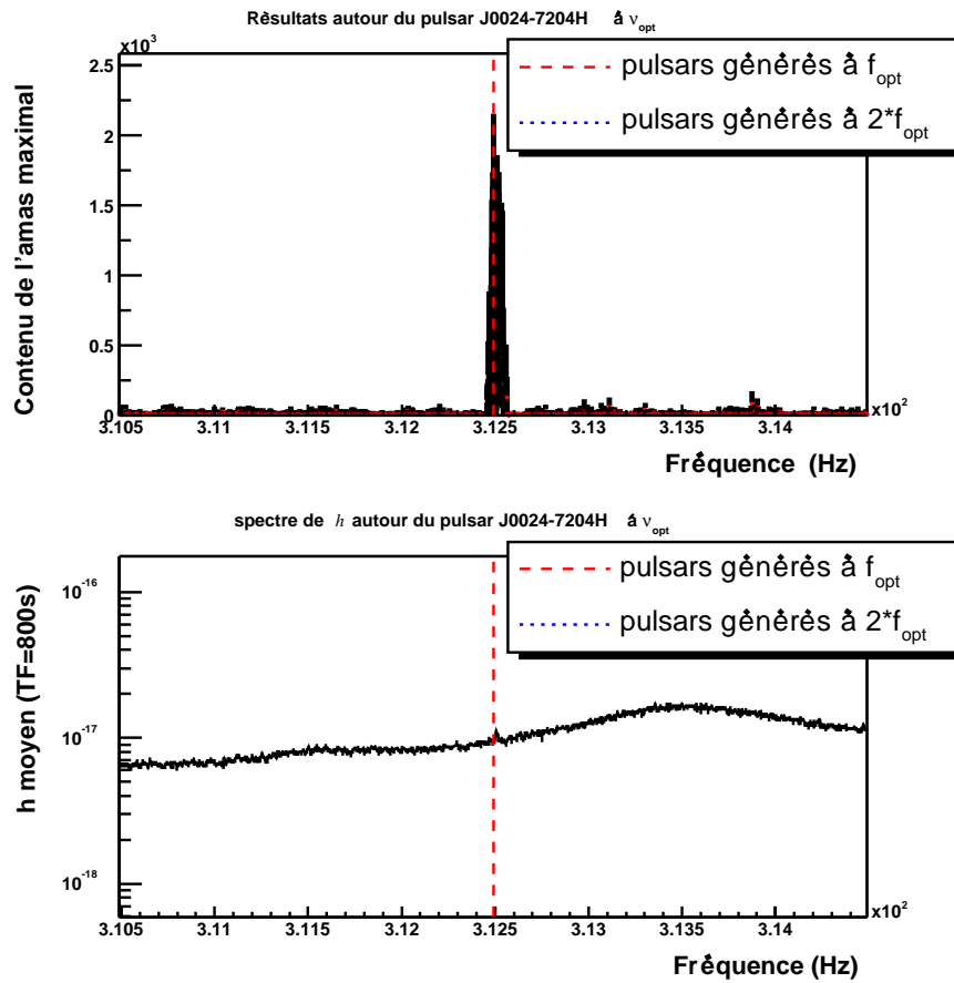
FIG. 7.17 – Moyenne des transformées de Fourier et résultat de l'analyse pour le pulsar J0024-7204H autour de sa fréquence de rotation.
