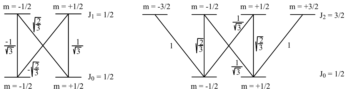
FIG. A.2 – Coefficients de Clebsch-Gordan pour une transition |J_0 = 1/2\rangle \rightarrow |J_1 = 1/2\rangle et pour une transition |J_0 = 1/2\rangle \rightarrow |J_2 = 3/2\rangle
