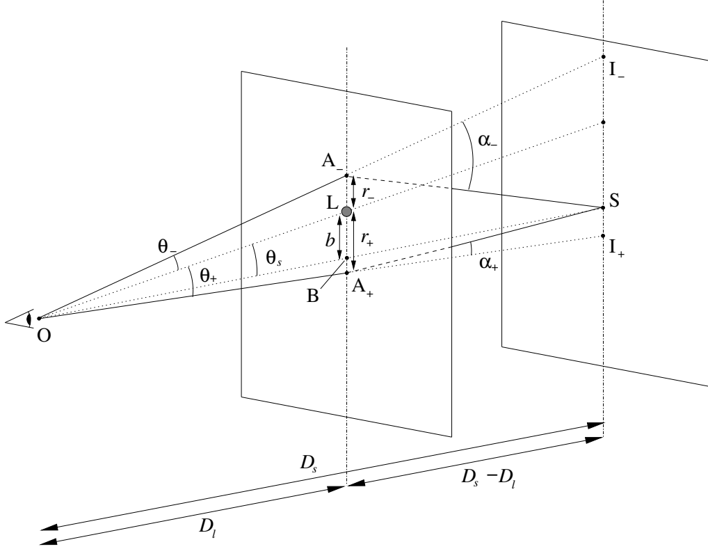
FIG. 2.1 – Déflexion de la lumière entre la source S et l'observateur O par un corps massif L, généralement désigné comme le défecteur ou la lentille. A_+ et A_- sont les intersections des rayons avec le plan du défecteur et I_+ et I_- les deux images dans le plan de S. La distance entre la lentille L et la ligne de visée est le paramètre d'impact b .
