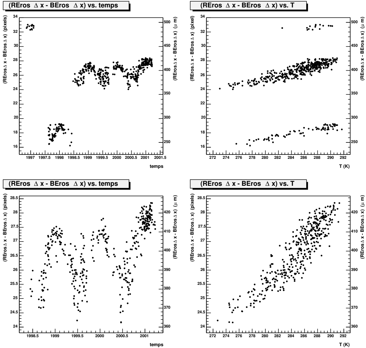
FIG. 5.7 – Évolution de l'écart (\Delta x)^{REROS} - (\Delta x)^{BEROS} en fonction du temps (à gauche) et en fonction de la température du télescope (à droite). Cet écart, converti en \mu m , correspond à la distance entre les régions pointées par les deux caméras. Son évolution en fonction du temps traduit les variations de l'écartement physique entre les caméras rouge et bleue. Il est intéressant de constater que cet écart évolue de façon saisonnière, avec un maximum vers janvier pendant l'été austral, et un minimum vers juin-juillet de chaque année (à gauche). Cet effet semble directement lié à la dilatation thermique de l'armature qui supporte les caméras, comme l'indiquent les deux figures de droite. Les variations brutales correspondent aux opérations de maintenance ayant conduit à démonter les caméras au printemps 1997 et en avril-mai 1998. Les figures supérieures utilisent toutes les données traitées, tandis que les figures inférieures n'utilisent que les données postérieures à mai 1998, pour s'affranchir des effets des opérations de maintenance.
