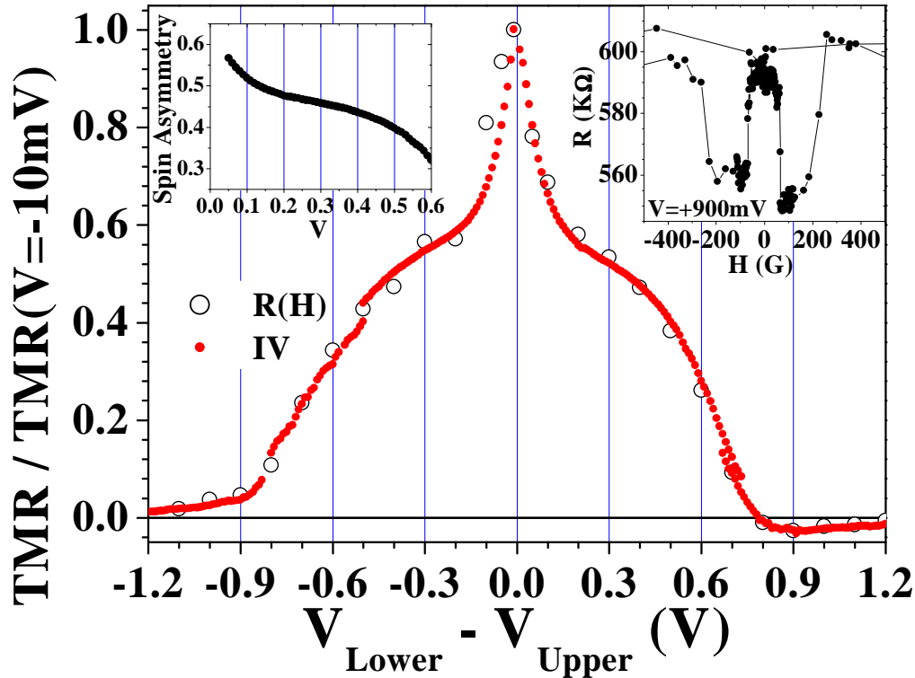
Figure 9.9: LSMO/STO/LSMO: dépendance en tension de la TMR à T=4 K. Inset de gauche: dépendance en tension de P^2 . Inset de droite: cycle R(H) à V=+900 mV montrant une TMR de -8%.
