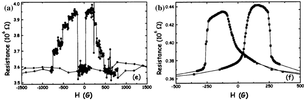
Figure 9.5: LSMO/I/Co: cycles R(H) à V=10\text{mV} pour (a) I=Al_2O_3 et (b) I=Al_2O_3/SrTiO_3 .
