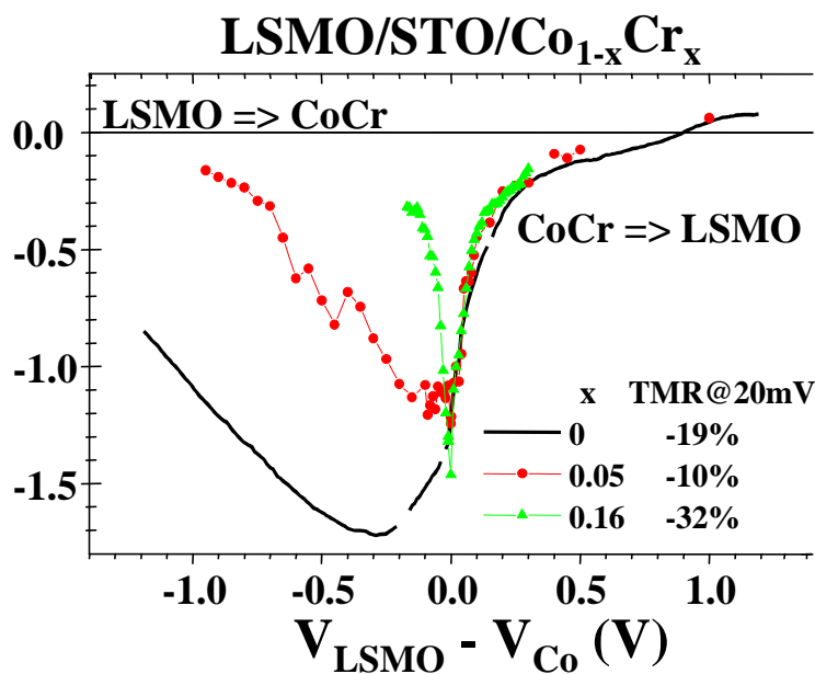
Figure 9.13: Dépendance en tension normalisée de jonctions \text{LSMO}/\text{STO}/\text{Co}_{1-x}\text{Cr}_x à T=30\text{K} . Les valeurs de TMR observées sont rapportées dans la légende. Les flèches indiquent le sens du transport d'électrons.
