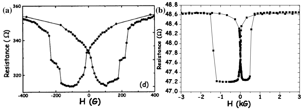
Figure 9.4: LSMO/I/Co: cycles R(H) à V=10\text{mV} pour (a) I=\text{Ce}_{0.69}\text{La}_{0.31}\text{O}_{1.845} et (b) I=\text{TiO}_2 . Le cycle asymétrique dans le cas \text{TiO}_2 reflète le couplage antiferromagnétique de \text{CoO} sur \text{Co} .
