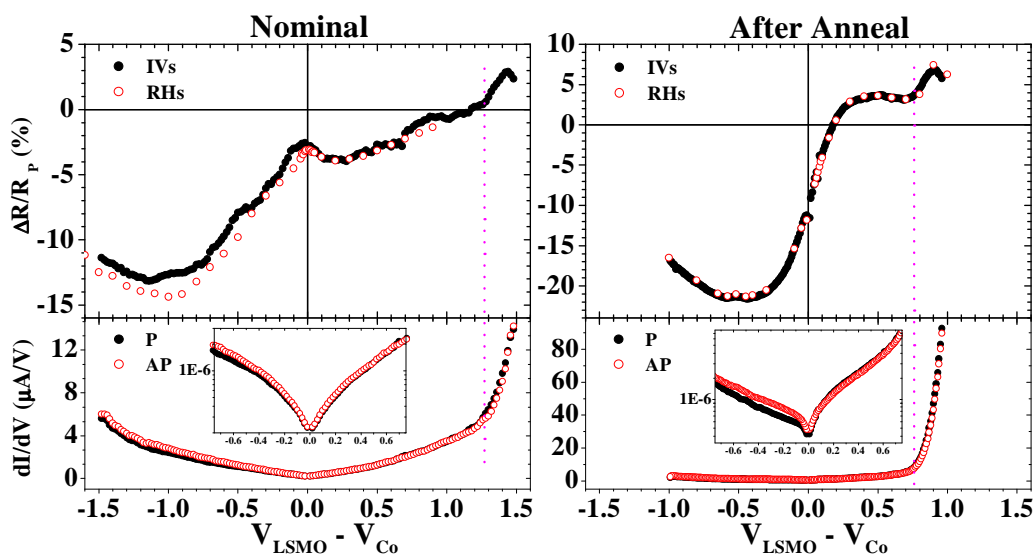
Figure 9.25: LSMO/STO/Co: Évolution des propriétés de magnéto-transport d'une jonction atypique (a) vierge et (b) après recuit : dépendance en tension de la TMR et de la conductance dans les états parallèle (P) et antiparallèle (AP). Les inserts aux panneaux inférieurs représentent les mêmes données à faible tension sur une échelle logarithmique.
