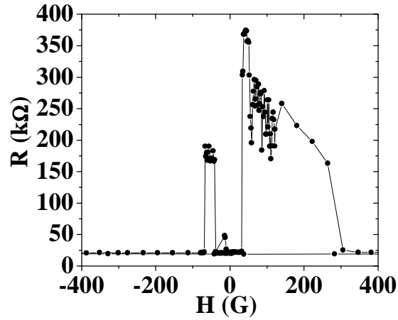
Figure 9.3: Magnétotransport de LSMO/STO/LSMO à T=4\text{K} . Jonction A de surface 64\mu\text{m}^2 : résistance en fonction du champ appliqué à V_{DC}=1\text{mV} .
