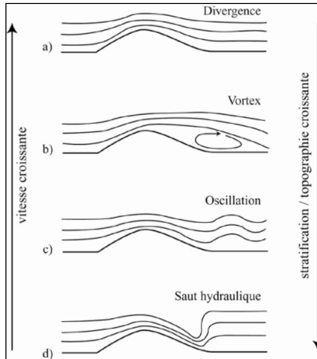
Figure 35 : Effet de la topographie, de la stratification en densité et de la vitesse de l'écoulement sur le comportement d'un écoulement en aval d'un obstacle a) divergences des lignes d'écoulement b) séparation des lignes d'écoulement (vortex) c) oscillation d) saut hydraulique (modifié d'après Kneller & Buckee 2000).
