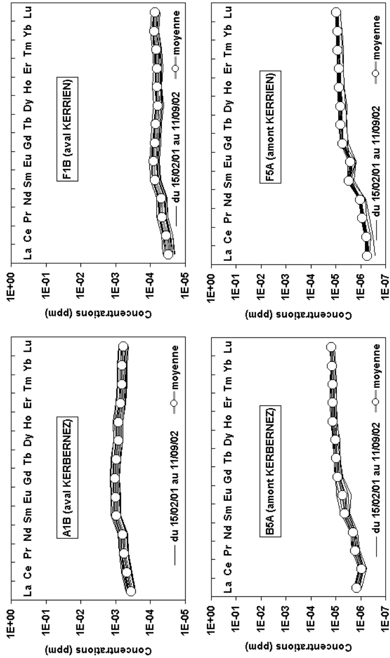
FIG. 3.22 – Spectres de REE dans les eaux souterraines des bassins versants de Kerbernez et Kerrien : domaines amont et aval. Les courbes noires représentent les spectres calculés à une fréquence mensuelle du 15/02/01 au 11/09/02.
