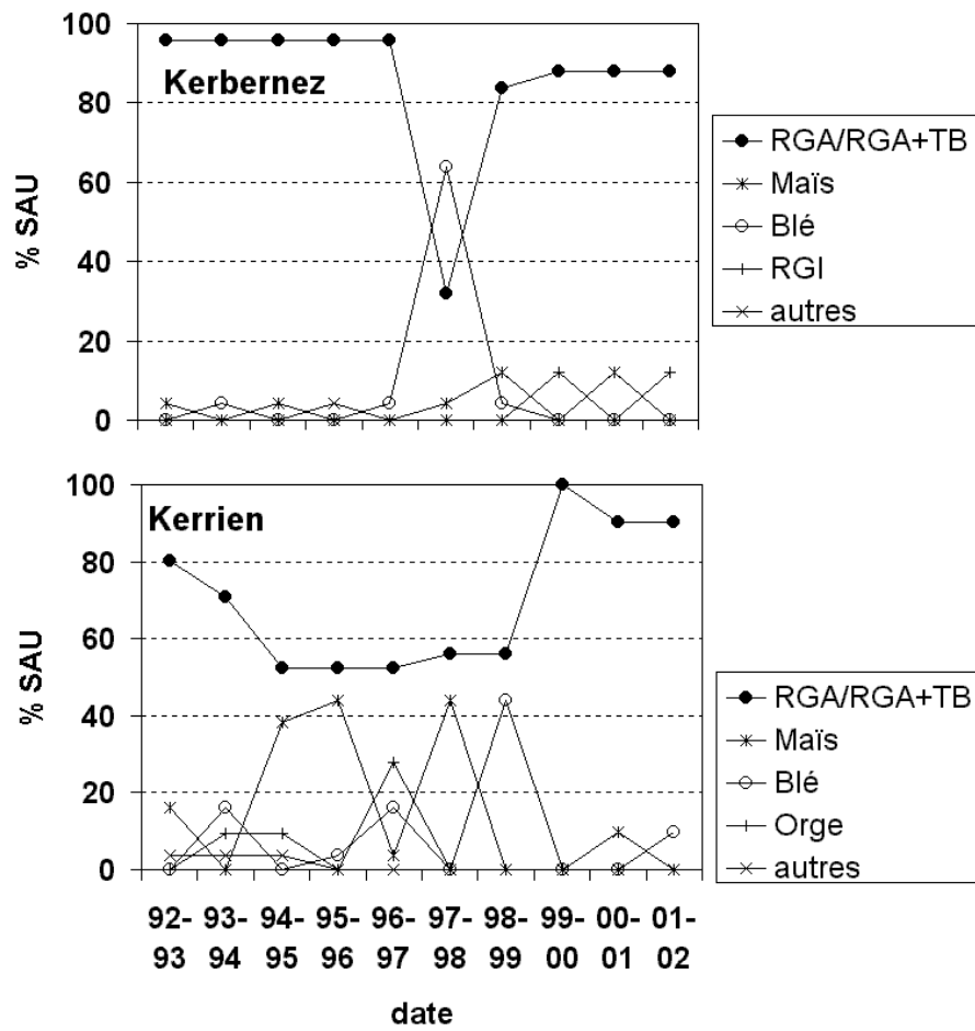
FIG. 2.9 – Evolution de l'assolement sur les bassins versants de Kerbernez et Kerrien. RGA = Ray-Grass Anglais, TB = Trèfle Blanc, RGI = Ray-Grass Italien.
