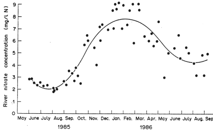
FIG. 1.3 – Exemple de cycle classique : concentrations en nitrate dans la rivière Burren (Irlande), années 1985 et 1986. Les mois de décembre à février représentent les périodes de fort drainage pendant lesquelles les teneurs en nitrate sont les plus fortes. D'après Neill (1989).
