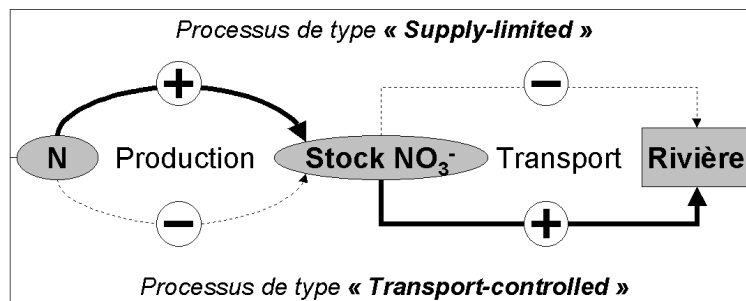
FIG. 1.6 – Processus de contrôle des variations saisonnières des concentrations en nitrate dans les eaux superficielles des bassins versants : Processus de type "Supply-limited", quand le stock d'azote est lié à la production annuelle (minéralisation), processus de type "transport-controlled" quand la production annuelle est inférieure au stock existant.
