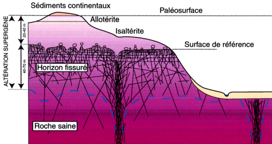
FIG. 1.7 – Représentation schématique des bassins versants armoricains. D'après Wyns (1998), cité dans Brault (2002).
