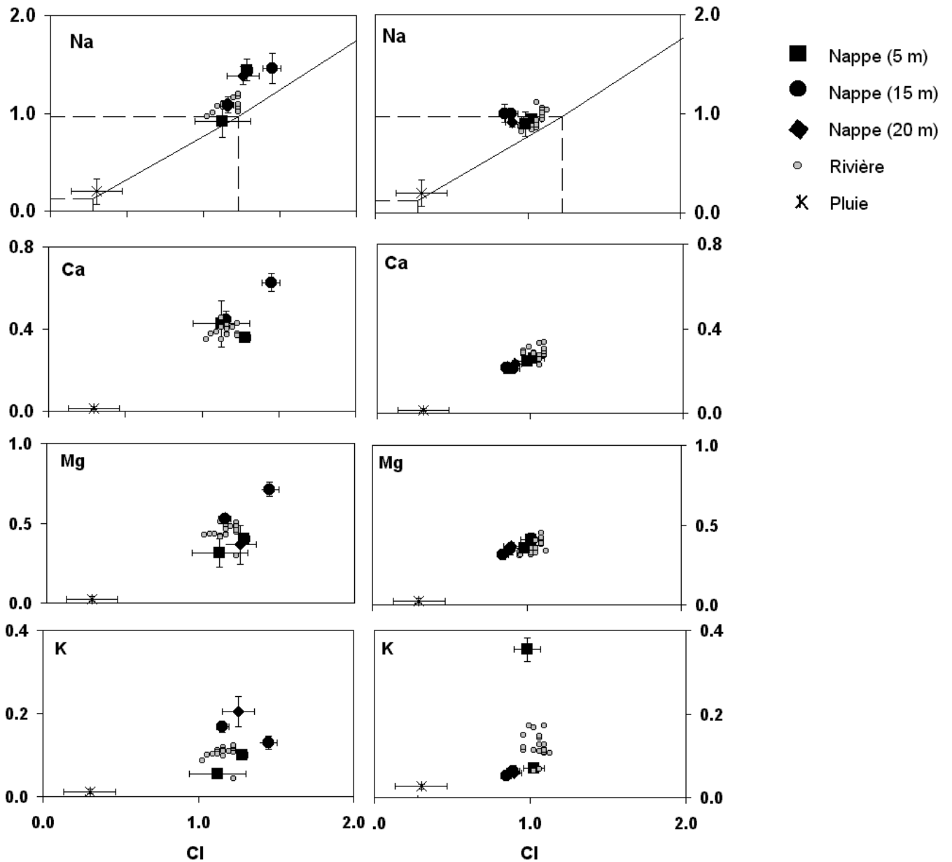
FIG. 3.27 – Concentrations ( \text{mmol.L}^{-1} ) en cations majeurs et chlorure dans les eaux de pluie, rivière et nappe des bassins versants de Kerbernez (diagrammes de gauche) et Kerrien (diagrammes de droite), pour les années 2000-2001 et 2001-2002. La droite de concentration de l'eau de pluie par évapotranspiration (trait plein), calculée avec un facteur de concentration égal à 2, ainsi que les valeurs attendues par concentration de l'eau de pluie par évapotranspiration (traites pointillés) sont indiquées sur le graphique \text{Na}=\text{f}(\text{Cl}) .
