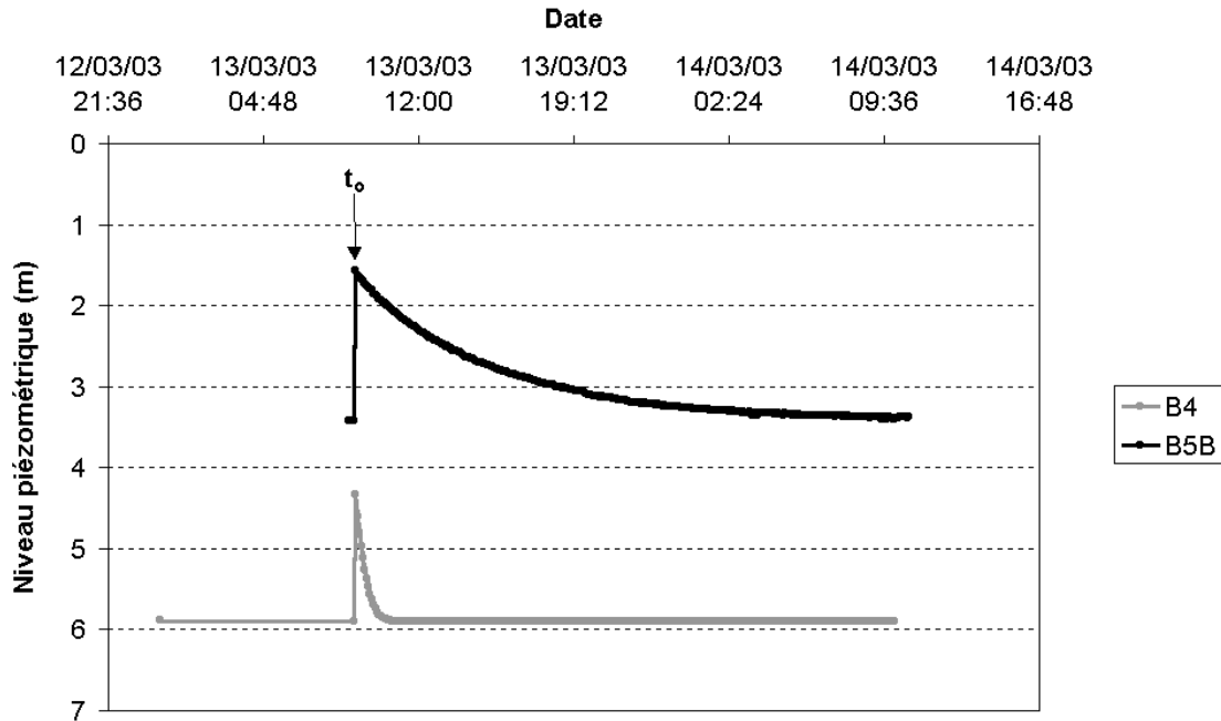
FIG. 2.15 – Mesure de choc hydraulique sur les piézomètres B4 et B5B. La méthode est appliquée en injectant au temps t_0 un volume d'eau dans les piézomètres et en mesurant à une fréquence de 15 minutes la descente du niveau piézométrique.
