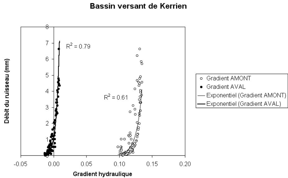
FIG. 3.10 – Relation entre débit et gradient piézométrique à l'amont et à l'aval du bassin versant de Kerrien.
