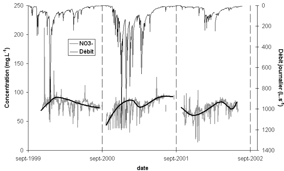
FIG. 1.10 – Teneurs en nitrate dans les eaux superficielles du bassin versant du Coët-Dan pour trois années hydrologiques contrastées. D'après Gruau et al. (2003).
