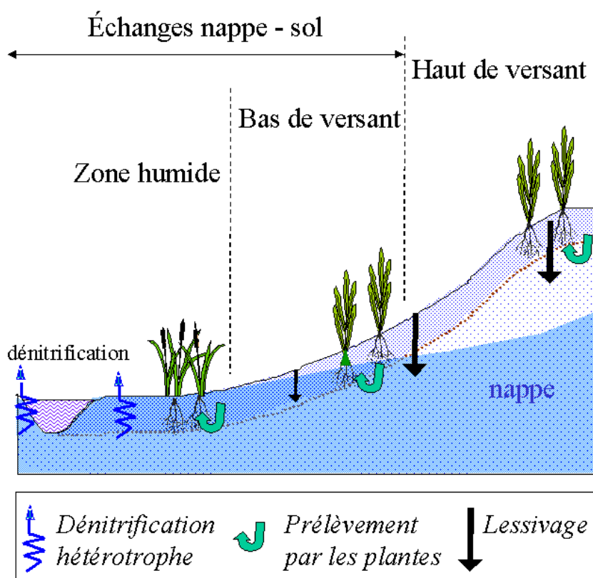
FIG. 1.8 – Chemins de l'eau et transformations d'azote associées dans un bassin versant sur socle.
