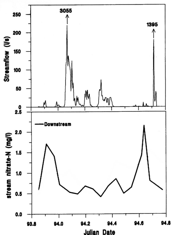
FIG. 1.4 – Exemple de cycle inversé : concentrations en nitrate dans la rivière du bassin versant de Logan (Ecosse), années 1993 et 1994. Les mois de décembre à avril représentent les périodes de fort drainage pendant lesquelles les teneurs en nitrate sont les plus faibles. D'après Hooda et al. (1997).
