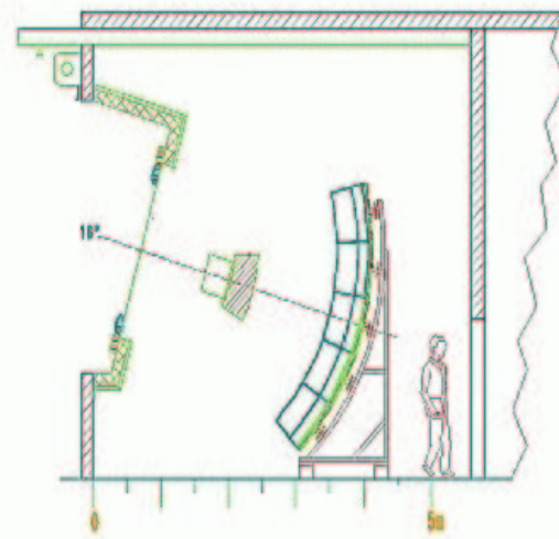
(b) Schéma.
