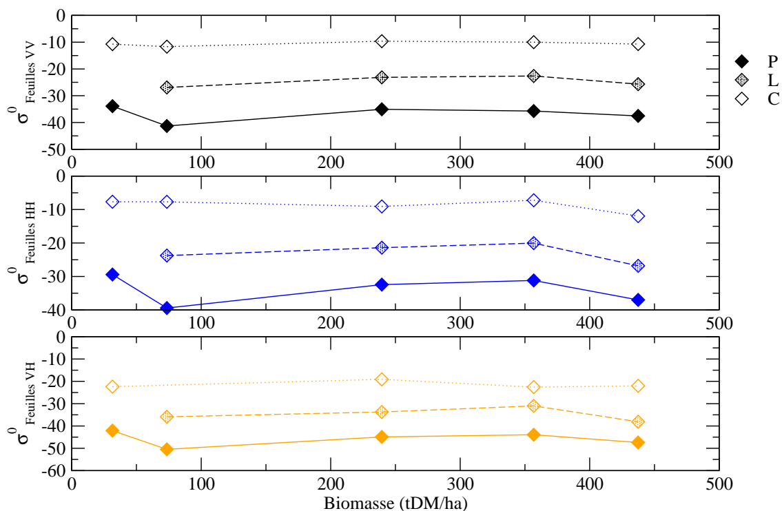
FIG. II.17 – Comparaison des contributions des feuilles au coefficient de rétrodiffusion pour différentes fréquences.
