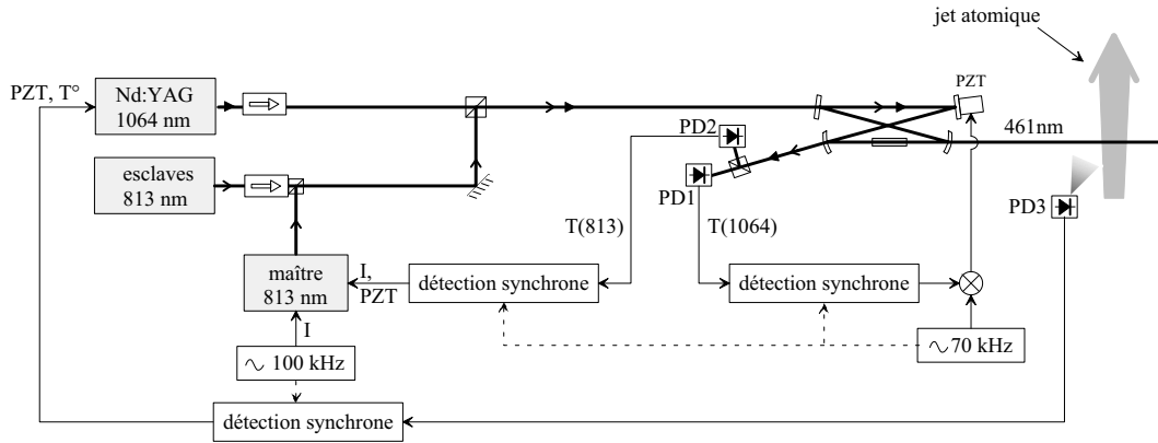
FIG. 1.13 – Schéma de principe des trois asservissements en fréquence utilisés pour la somme de fréquence.
