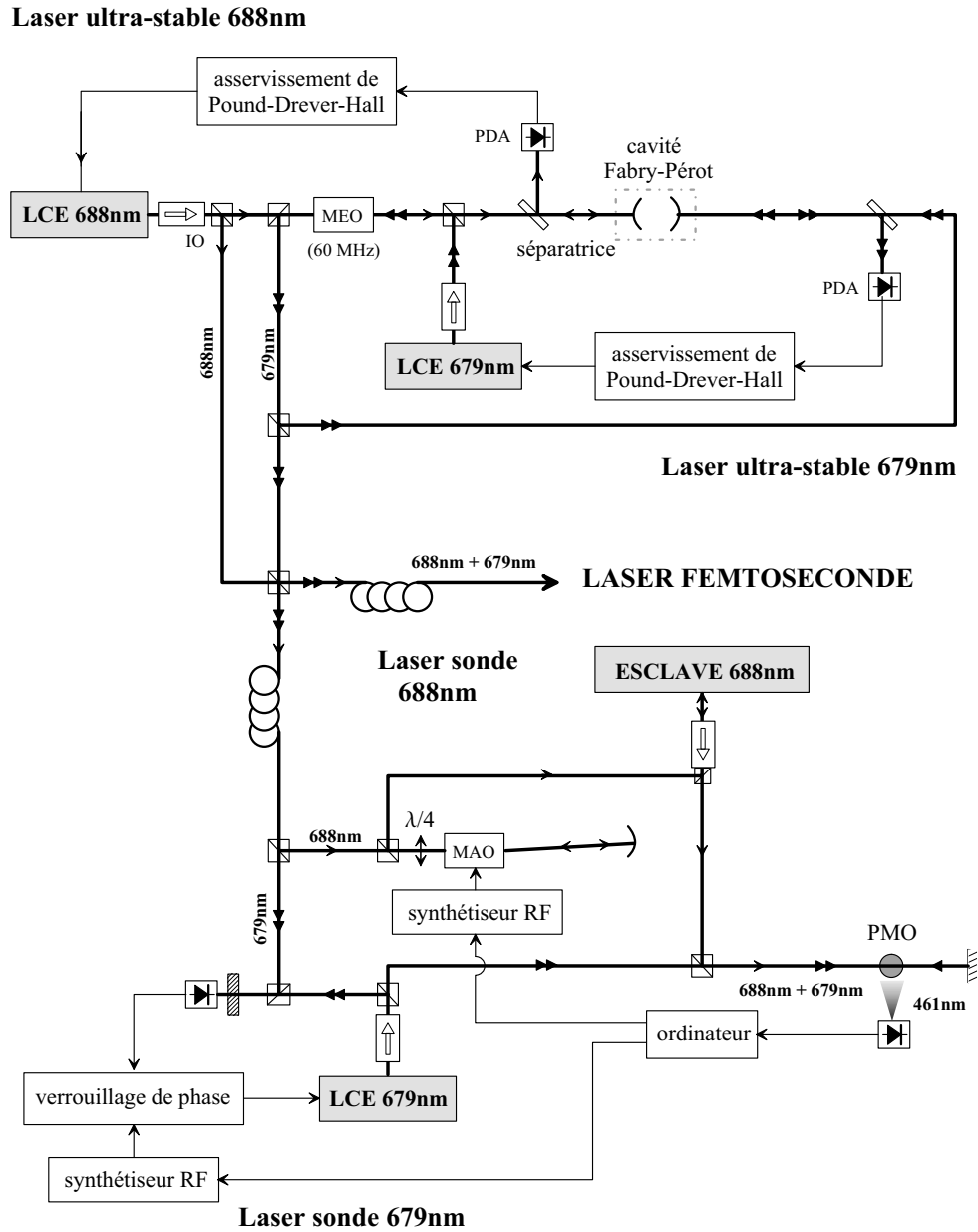
FIG. 5.22 – Schéma expérimental permettant d'interroger les atomes avec deux jeux de laser {laser ultra-stable; laser sonde} à 679 et 688 nm.
