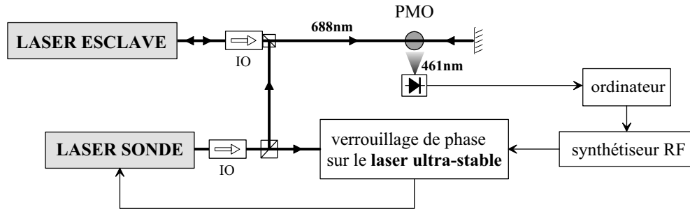
FIG. 5.11 – Le laser sonde injecte la diode esclave qui est utilisée pour interroger les atomes du PMO. La fluorescence induite par les faisceaux du piège à 461 nm permet de détecter la transition {}^3P_1 - {}^3S_1 à 688 nm.
