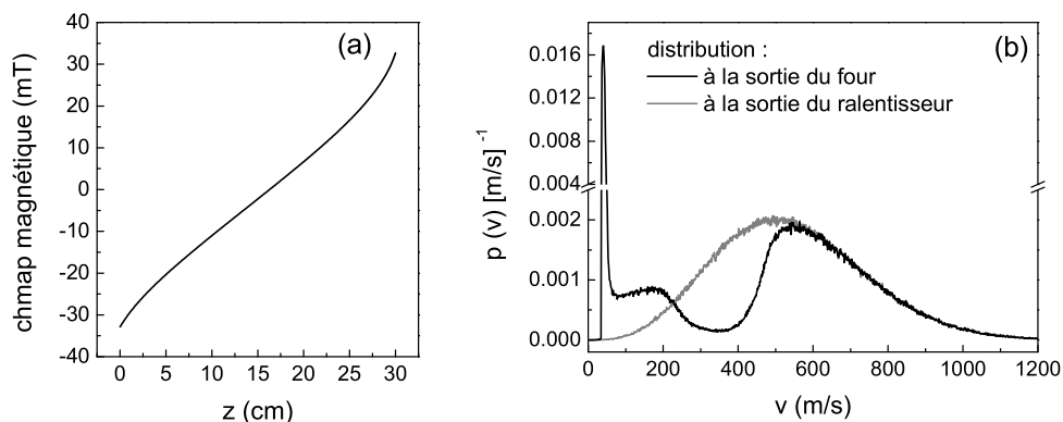
FIG. 2.9 – (a) Champ magnétique du ralentisseur pour le jeu de paramètres optimisant N_p : \eta = 0.4 , w_e=1 mm, w_s=8 mm avec P_L=30 mW, z_s=30 cm et pour \delta = -560 MHz. (b) Distribution de la vitesse longitudinale à la sortie de ce ralentisseur Zeeman. Simulation effectuée pour un four chauffé à 600^\circ\text{C} .
