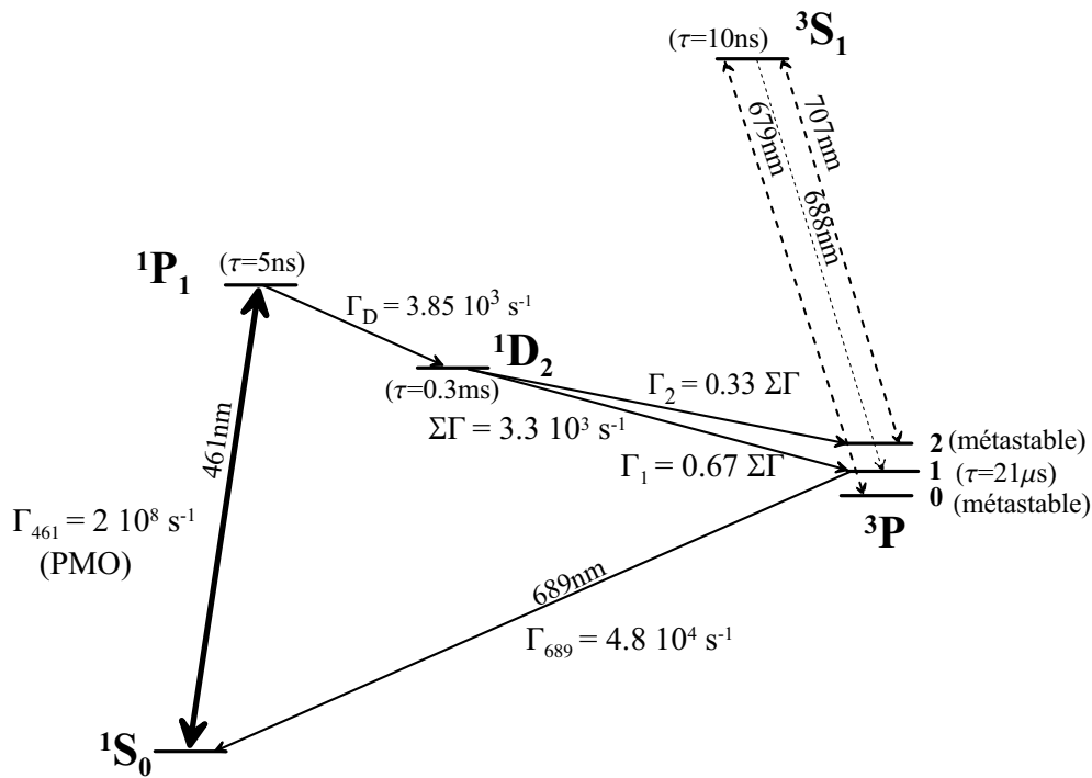
FIG. 3.10 – Niveaux atomiques du strontium.
