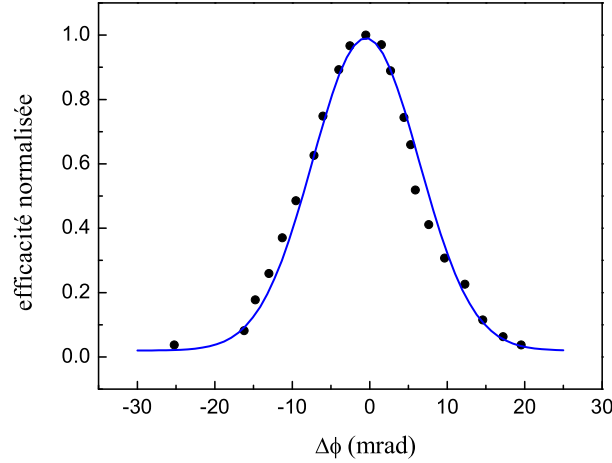
FIG. 1.6 – Efficacité de conversion de la somme de fréquence dans un cristal de KTP de 2 cm de long, tracée en fonction de l'écart angulaire \Delta\phi par rapport à l'angle optimal ( \phi = 81.3^\circ ).
