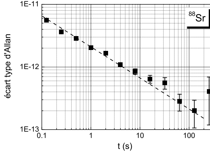
FIG. 5.5 – Écart type d'Allan en valeur relative d'une série de 11 mn de mesure de fréquence de la transition ^1S_0 - ^3P_1 du ^{88}\text{Sr} . Mesures effectuées avec un faisceau elliptique 670\ \mu\text{m} \times 3\ \text{mm} (diamètres à 1/e^2 ), avec une puissance de 250\ \mu\text{W} .
