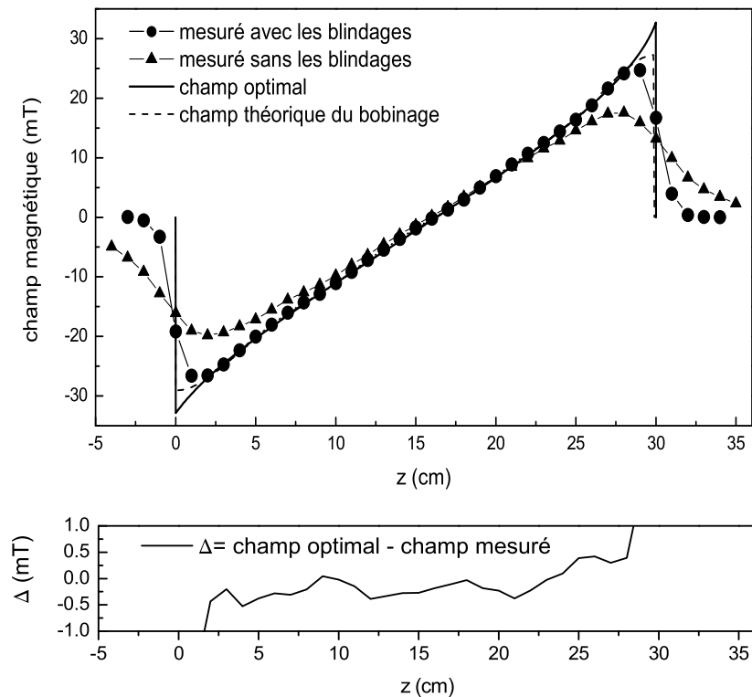
FIG. 2.11 – Comparaison entre les différents champ magnétiques : champ optimal obtenu suite à l'étude du ralentisseur Zeeman (trait continu), champ théorique pour le bobinage réalisé avec I=16 A (pointillés), mesures à cette intensité avec les bobines à l'intérieur du blindage magnétique (cercles) et sans le blindage (triangles).
