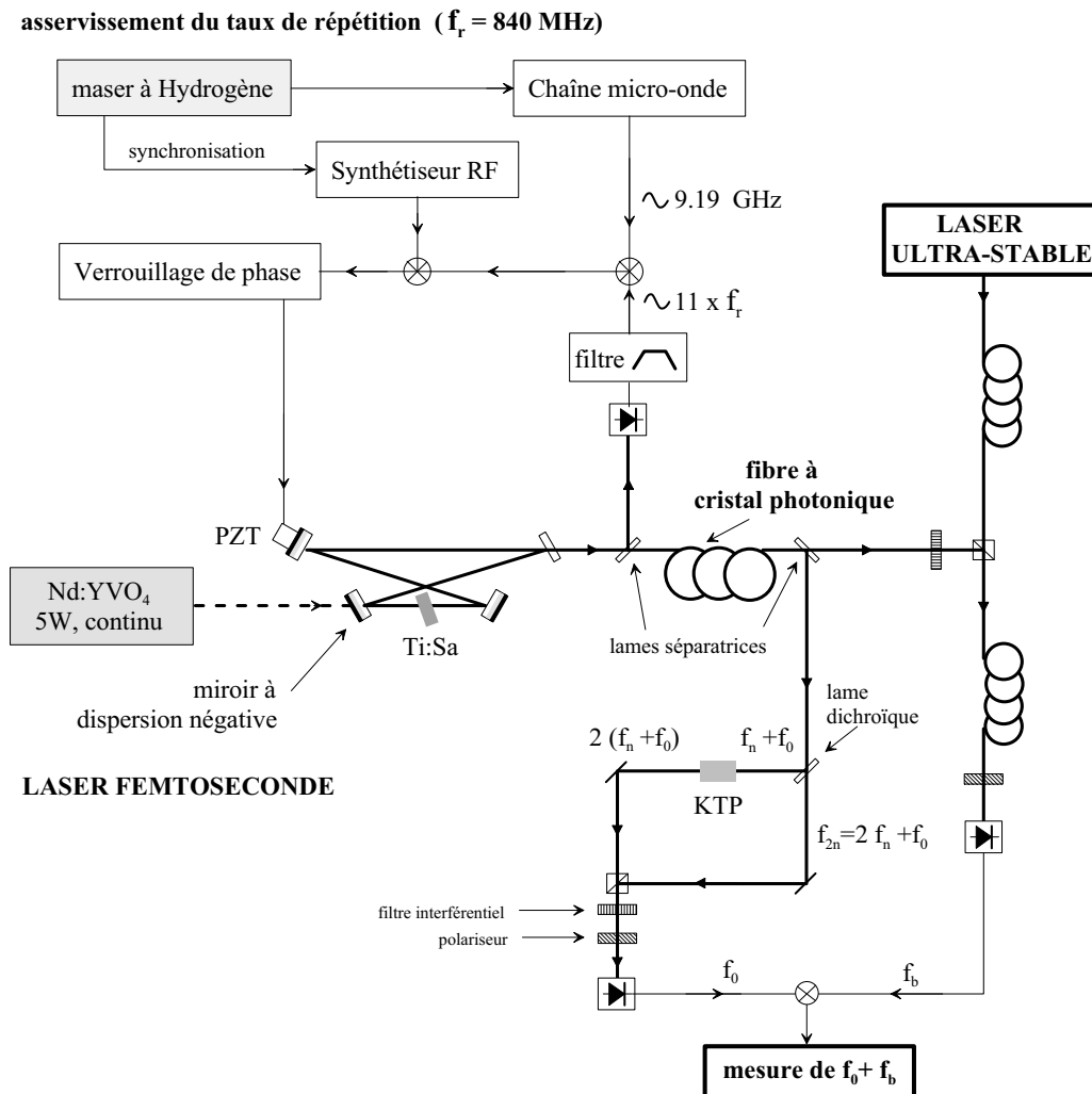
FIG. 4.10 – Schéma de principe de la mesure de fréquence du laser ultra-stable. Le laser femtoseconde est un laser Ti :Sa pompé par un laser Nd :YVO 4 . Le peigne de fréquence est élargi par une fibre à cristal photonique. Le taux de répétition ( f_r ) est asservi sur un maser à hydrogène. Pour mesurer le décalage à l'origine du peigne de fréquence ( f_0 ) on double la fréquence de la n^{\text{ième}} raie dans la partie infrarouge du peigne et on la mélange avec celle de la 2n^{\text{ième}} raie. f_b est le battement entre le laser ultra-stable et le mode le plus proche du peigne.
