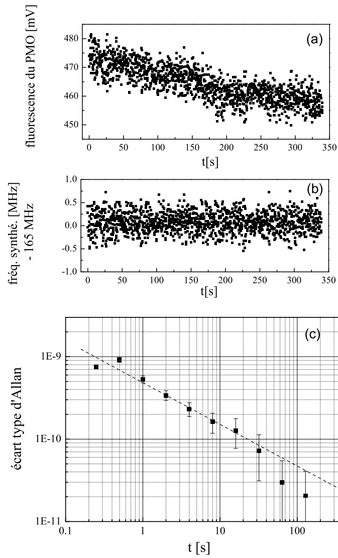
FIG. 5.13 – Mesure de la transition {}^3P_1 - {}^3S_1 du {}^{88}\text{Sr} . (a) : fluorescence moyenne du PMO. (b) : fréquence centrale du synthétiseur RF. (c) : écart type d'Allan en valeur relative de la fréquence absolue de la transition atomique.
