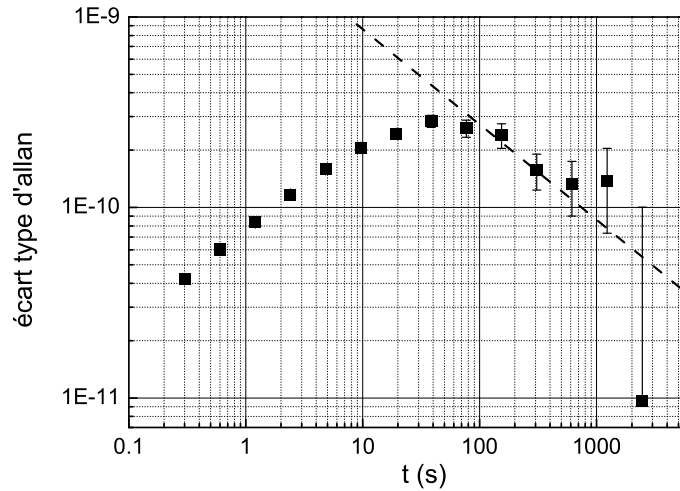
FIG. 6.10 – Écart type d'Allan en valeur relative de la fréquence du laser asservi sur la transition ^1S_0 - ^3P_0 . Série de 18 000 points de mesures effectués à la fréquence de 3 Hz.
