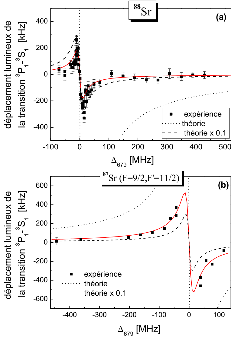
FIG. 5.25 – Déplacement lumineux de la transition {}^3P_1 - {}^3S_1 induit par le laser à 679 nm en fonction de \Delta_{679} , décalage de fréquence par rapport à la résonance {}^3P_0 - {}^3S_1 . Le zéro du déplacement lumineux correspond à la fréquence de la transition {}^3P_1 - {}^3S_1 mesurée sans le laser à 679 nm. Les mesures ont été effectuées avec des faisceaux lasers ayant un rayon w_{679}=1.3 mm et w_{688}=0.9 mm et une intensité moyenne I_{679}=180 mW/cm 2 et I_{688}=0.2 mW/cm 2 . En pointillés on a représenté le déplacement lumineux théorique pour un atome à deux niveaux avec \Gamma/(2\pi)=15.9 MHz et \Omega/(2\pi)=16.3 MHz.
