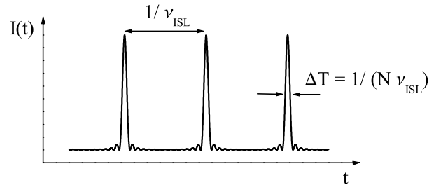
FIG. 4.6 – Intensité du laser en mode bloqué pour N=15 modes. Le taux de répétition est égal à l'intervalle spectral libre ( \nu_{ISL} ).
