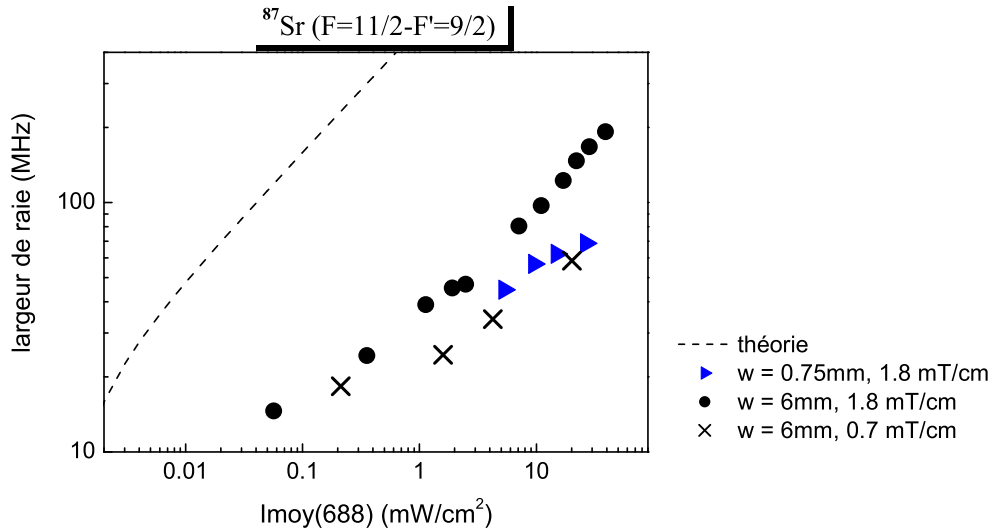
FIG. 5.15 – Largeur à mi-hauteur de la résonance {}^3P_1, F = 11/2 - {}^3S_1, F = 9/2 tracée en fonction de l'intensité du laser sonde moyennée sur la taille du piège (2 mm). On a fait varier la taille du faisceau ( w ) et le gradient de champ magnétique du PMO (mT/cm).
