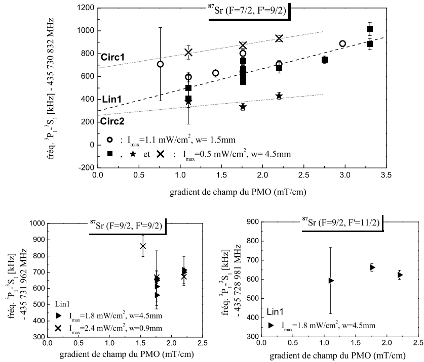
FIG. 5.18 – Effet du champ magnétique du PMO. La polarisation, l'intensité maximale ( I_{max} ) et le rayon ( w ) du laser à 688 nm sont spécifiées pour chaque transition.
