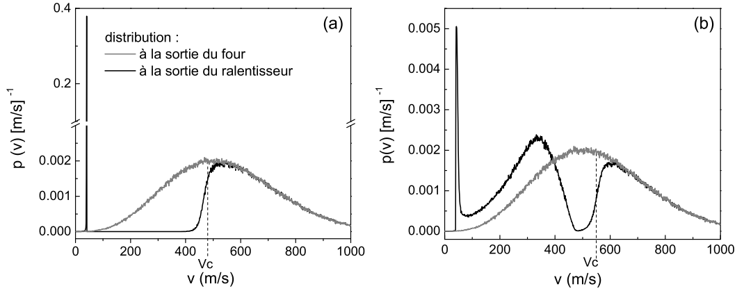
FIG. 2.3 – Distribution de la vitesse longitudinale à la sortie du four chauffé à 600^\circ\text{C} (en gris) et à la sortie du ralentisseur (en noir). (a) : Simulation effectuée en considérant un faisceau laser de 4 mm de diamètre avec un paramètre de saturation constant, égal à 1. (b) : Simulation effectuée en considérant un faisceau gaussien de 4 mm de rayon à 1/e^2 , avec s=2.8 au centre du faisceau ( P_L=30 mW). (a, b) : La longueur du ralentisseur est de 30 cm et \eta=0.7 . v_c est la vitesse de capture théorique.
