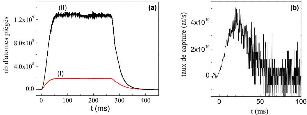
FIG. 3.13 – (a) Charge et décharge du PMO observées en chauffant le four à 630^{\circ}\text{C} , avec une puissance de 17 mW dans les faisceaux du piège et 32 mW dans celui du ralentisseur Zeeman. Les courbes (I) et (II) représentent le nombre d'atomes piégés calculé respectivement à partir de la fluorescence induite par le PMO ( N_p^{PMO} ) et renormalisé pour tenir compte de l'absorption dans les faisceaux du piège. (b) Taux de capture du piège qui est la dérivée de la courbe de chargement du PMO renormalisée.
