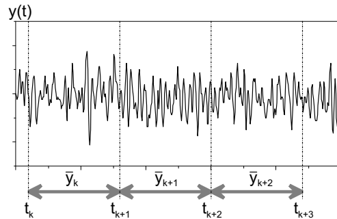
FIG. C.1 – Calcul de la variance d'Allan d'un signal aléatoire.
