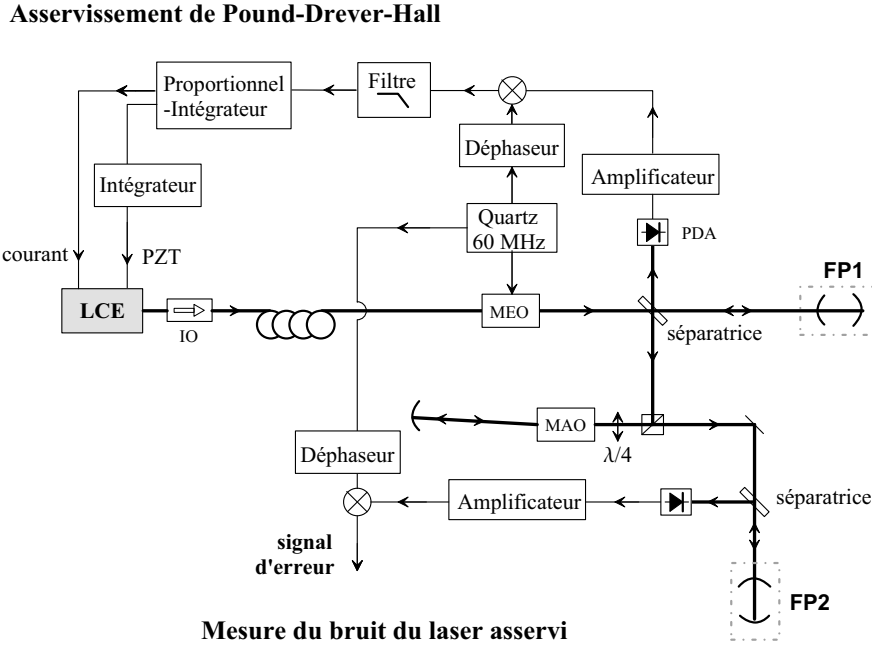
FIG. 4.4 – Montage expérimental utilisé pour asservir le laser sur la cavité Fabry-Pérot FP1 et pour caractériser son bruit avec FP2.
