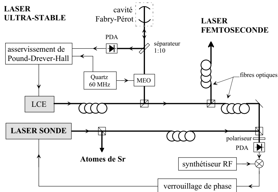
FIG. 4.1 – Schéma de principe des mesures absolues de fréquence des transitions atomiques. LCE : diode laser montée en cavité étendue.
