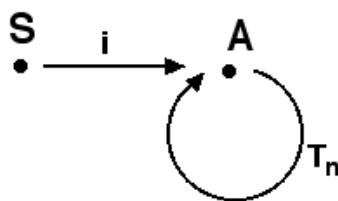
Figure 47 : Un mode à transposition limitée comme limite d'un diagramme à un seul objet et une seule flèche dans la catégorie des \mathbf{Z} -module \text{Mod}_{\mathbf{Z}}
