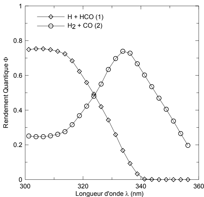
Figure VII.7 Rendements quantiques des deux voies de photolyse (réactions (1) et (2)) du formaldéhyde ( HCHO ) en fonction de la longueur d'onde d'irradiation à température et pression ambiantes (données sources : DeMore et al., 1997).
