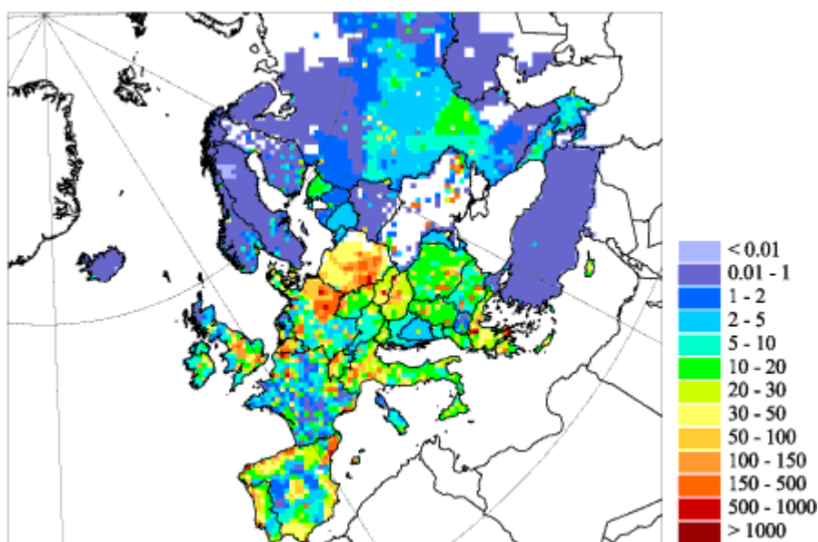
Figure I.3 Distribution spatiale (grille de résolution 50 km × 50 km) des flux d'émissions anthropiques de mercure en Europe en g/km²/an en 2000 (Ilyin et al. , 2003).
