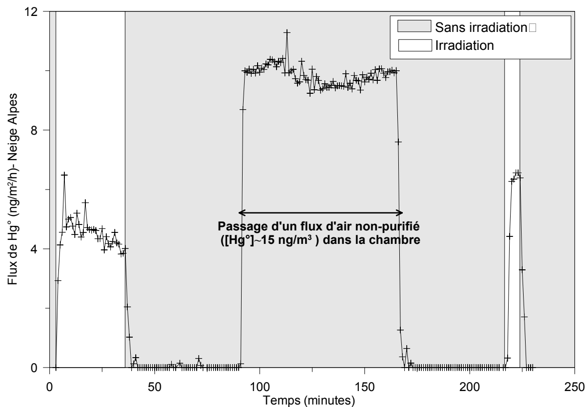
Figure VII.9 Flux de mercure gazeux ( ng/m^2/h ) mesurés pendant des périodes d'irradiation (en blanc) et d'obscurité (en gris) pour la neige des Alpes. Entre les deux périodes d'irradiation, un flux d'air de la pièce non purifié alimente la chambre. Les points reportés sur le graphe au cours de cette période ne représentent pas les flux provenant de la neige mais l'illustration du passage de l'air contaminé en mercure. L'intervalle de temps entre chaque mesure est de 5 minutes.
