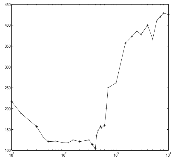
Figure VI.16 – Évaluation de la qualité de la reconstruction (au sens du critère (VI.4)) de polygones à 20 sommets. Ces courbes représentent la quantité \mathcal{H}(\mathbf{f}^\dagger, \hat{\mathbf{f}}^\dagger) (où n^\dagger = 64 \times 64 pixels) en fonction de \lambda , où \lambda est représenté aux échelles courante (a) et logarithmique (b).
