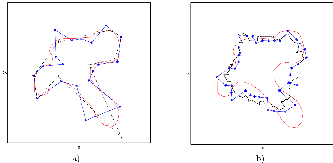
Figure VI.14 – Traitement du jeu de données (I) par l'approche polygonale ; estimation \hat{\mathbf{v}}_{\text{MC}}(n) par moindres carrés pour n = 10, 20, 50, 100 sommets. Outre l'objet réel, sont représentés : a) \hat{\mathbf{v}}_{\text{MC}}(10) et \hat{\mathbf{v}}_{\text{MC}}(20) , en traits pointillés et pleins, b) \hat{\mathbf{v}}_{\text{MC}}(50) et \hat{\mathbf{v}}_{\text{MC}}(100) , en traits étoilés et pleins.
