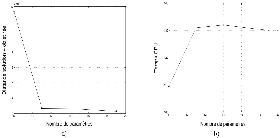
Figure VI.12 – Traitement des données (III) par la méthode harmonique. Influence du nombre n de paramètres du développement (paramètres a_i^k ) sur la qualité des reconstructions, mesurée par les deux critères définis au § VI.1.2, où n^\dagger = 128^3 voxels. Les temps CPU obtenus pour n = 16, 32 et 64 sont sensiblement égaux car la convergence de l’algorithme local est plus rapide dans les deux derniers cas.
