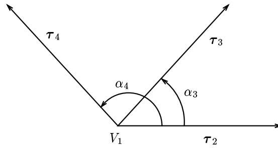
Figure E.1 – Tétraèdre plan. Cas où les directions adjacentes à V_1 sont situées dans le même demi-plan. L'angle solide vaut A_1(\mathcal{T}) = 0 .
