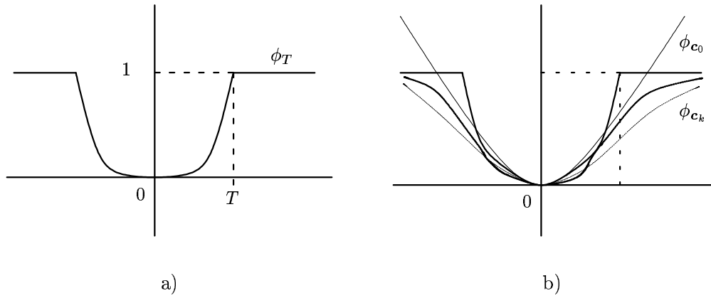
Figure II.2 – Principe du GNC. a) Régularisation par une loi gaussienne tronquée (fonction \mathcal{L}_2\text{-}\mathcal{L}_0 ). b) Fonctions \phi_{c_k} approximant \phi .
