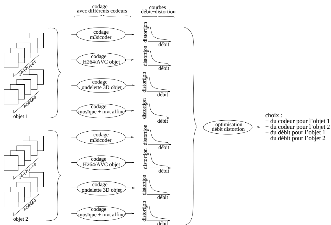
FIG. 2.1 – Schéma du codage dynamique que nous proposons. L'illustration est donné pour le codage dynamique de deux objets
