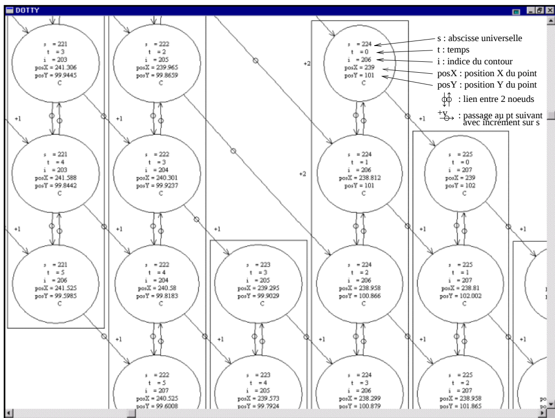
FIG. 2.8 – Visualisation sous dotted d'une partie du graphe résultant de l'alignement du groupe de contour. Chaque point de chaque contour possède une abscisse universelle
