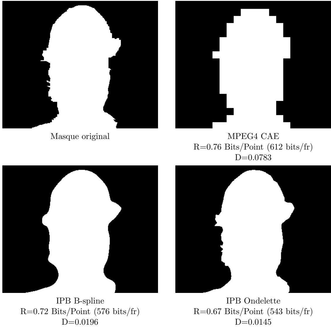
FIG. 3.2 – Comparaison des techniques de codage pour un débit d'environ 0.7 bits par élément de contour (environ 600 bits par images à 15Hz)
