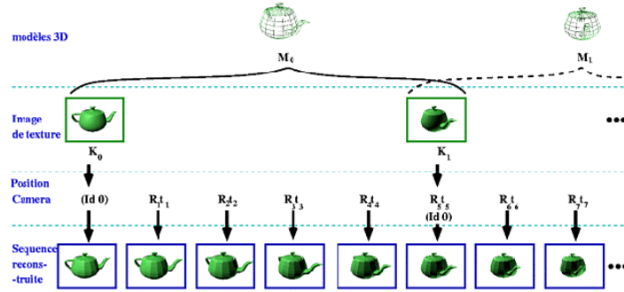
(b) partie synthèse du m3ddecoder. Reconstruction de la vidéo à partir : du modèle 3D, des positions caméra et de 2 images de texture
