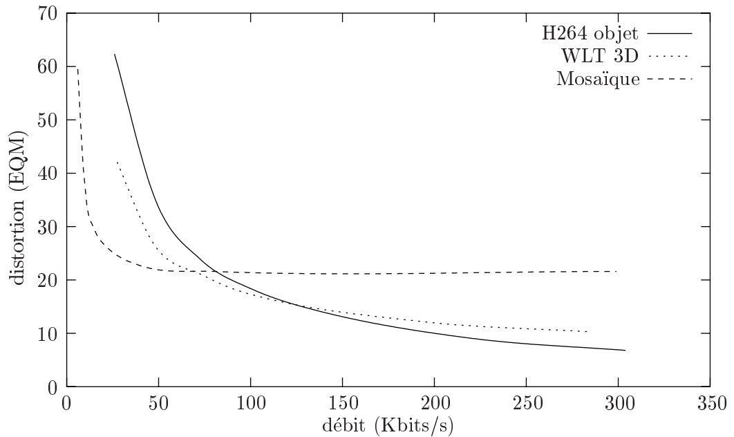
FIG. 3.1 – Courbe de la distortion (moyenne sur 60 images de l'erreur quadratique moyenne) en fonction du débit. Le codage porte sur l'arrière-plan de la séquence CIF Foreman à 15Hz. Les codeurs utilisés sont : H264/AVC adapté objet, ondelette 3D (WLT 3D) et mosaïque avec un mouvement affine
