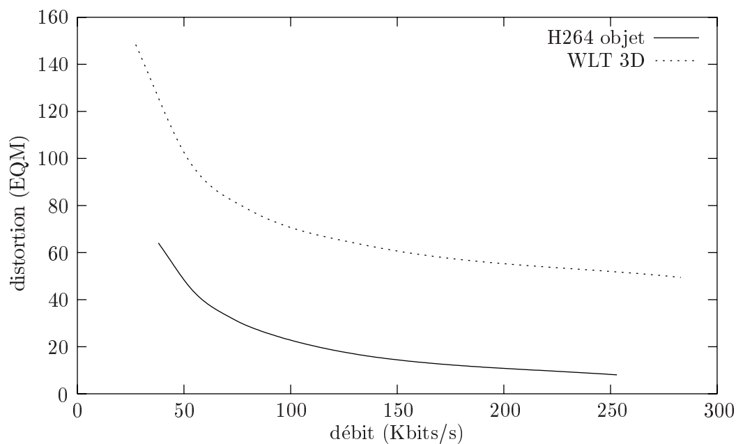
FIG. 3.2 – Courbe de la distortion (moyenne sur 60 images de l'erreur quadratique moyenne) en fonction du débit. Le codage porte sur l'avant-plan de la séquence CIF Foreman à 15Hz. Les codeurs utilisés sont : H264/AVC adapté objet, et ondelette 3D (WLT 3D)
