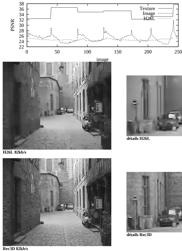
FIG. 2.3 – Comparaison H26L et m3ddecoder à 82Kb/s sur la séquence Rue CIF à 25 Hz. Les qualités PNSR sont d'environ 26dB pour m3ddecoder et 25 dB pour H26L. Par contre la qualité subjective est très largement supérieure pour le m3ddecoder
