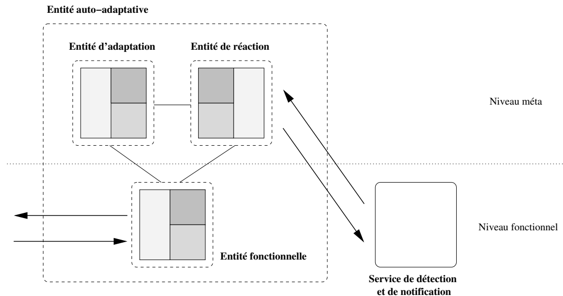
FIG. 5.13 – Structure d'une entité auto-adaptative
