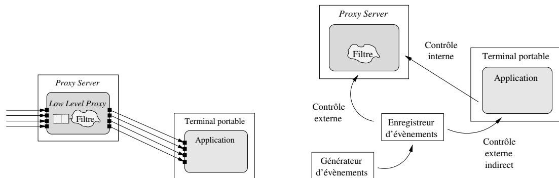
FIG. 3.7 – Low Level Proxy dans l'approche de Zenel et al.
