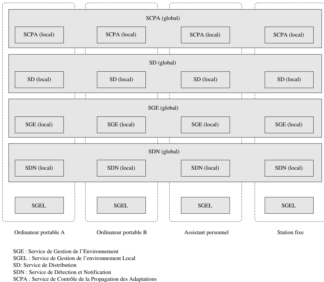
FIG. 6.8 – Architecture du système de gestion des ressources et de distribution des applications
