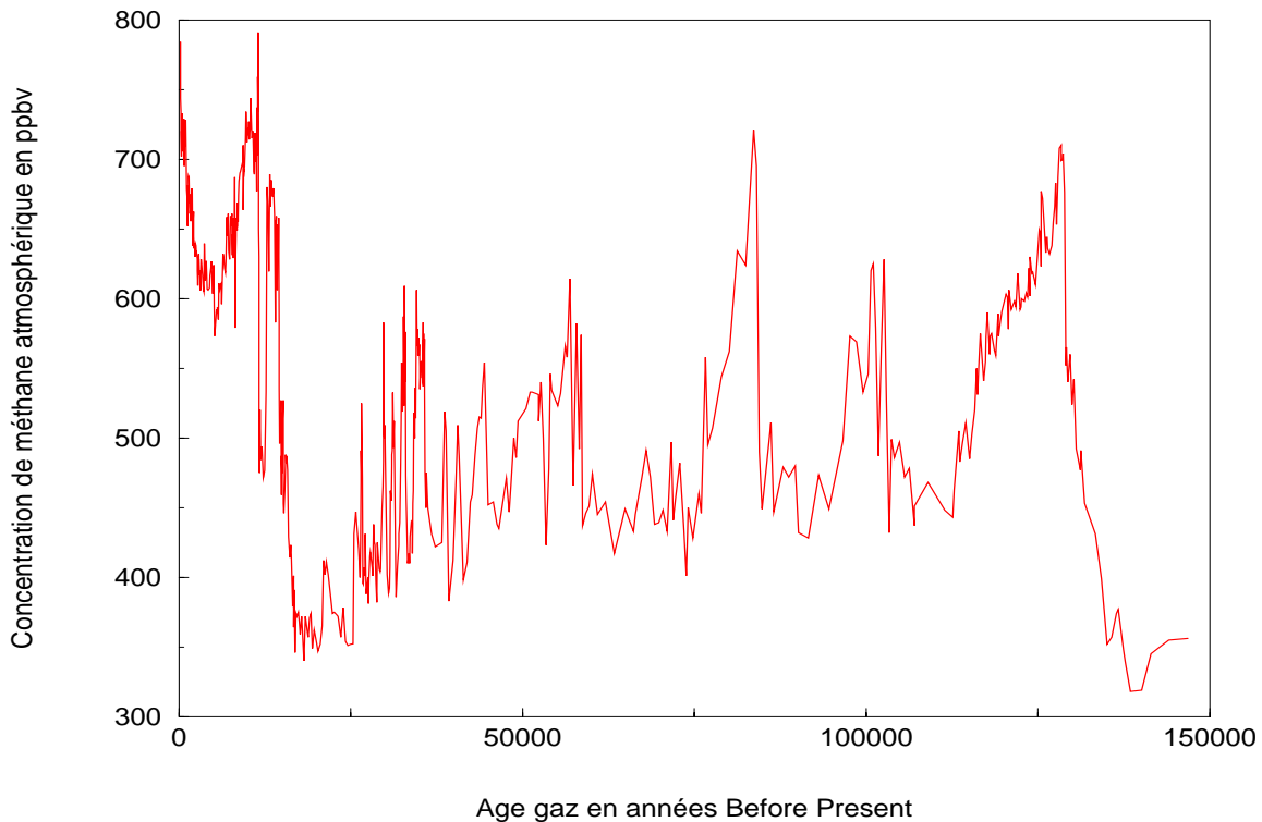
Fig. 4.1 : Concentrations en méthane atmosphérique depuis 150000 ans à partir des forages GRIP et GISP2 au Groenland, et à Vostok, reconstruites d'après Chappellaz et al. (1993) .
