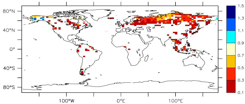
Profondeur maximale au Present
