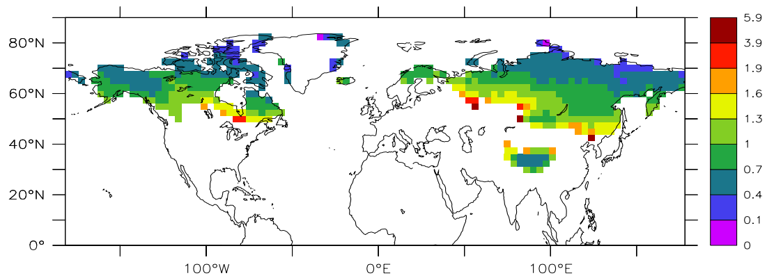
Profondeur de degel (0 k)
