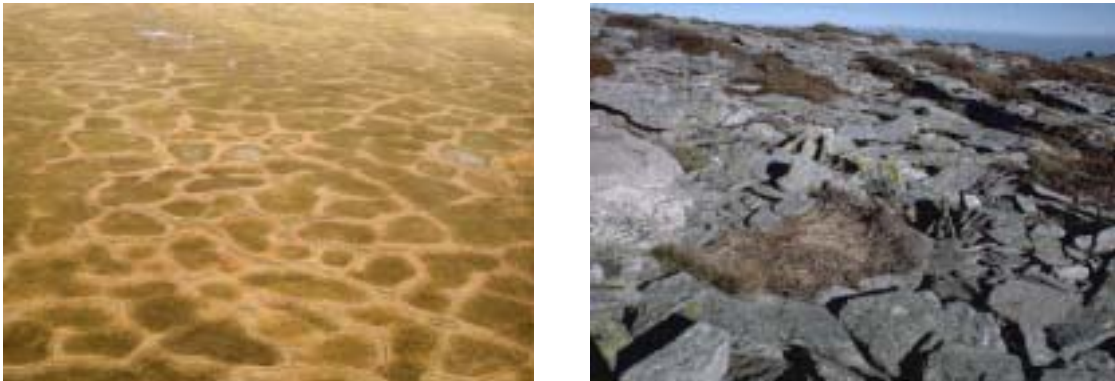
Fig. 2.4 : A gauche : réseau de fentes de gel en Terre de Baffin (Canada). A droite : cercles de pierres fossiles retrouvés au Mont Mézenc (France, 1753 m d'altitude, 45°N).
