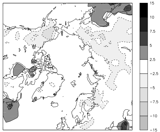
PD-NF - L&W (summer)
