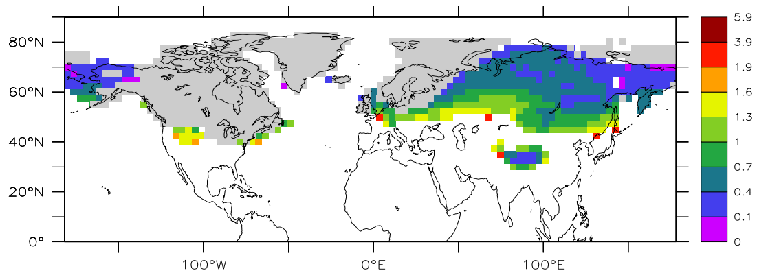
Profondeur de degel (21 k)
