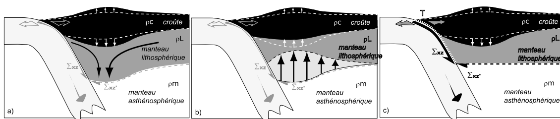
FIG. 3.5.21 – Trois processus pouvant accroître l'altitude. Les flèches noires désignent les mécanismes prépondérants. Les pointillés blancs indiquent la surface topographique et la Moho antérieurs à la mise en place du processus. a) Épaississement dû à une instabilité gravitaire du manteau lithosphérique ; b) Ablation convective du manteau lithosphérique ; c) Épaississement par les contraintes aux limites de la plaque (cisaillement sur le plan de Benioff et à la base de la lithosphère).
