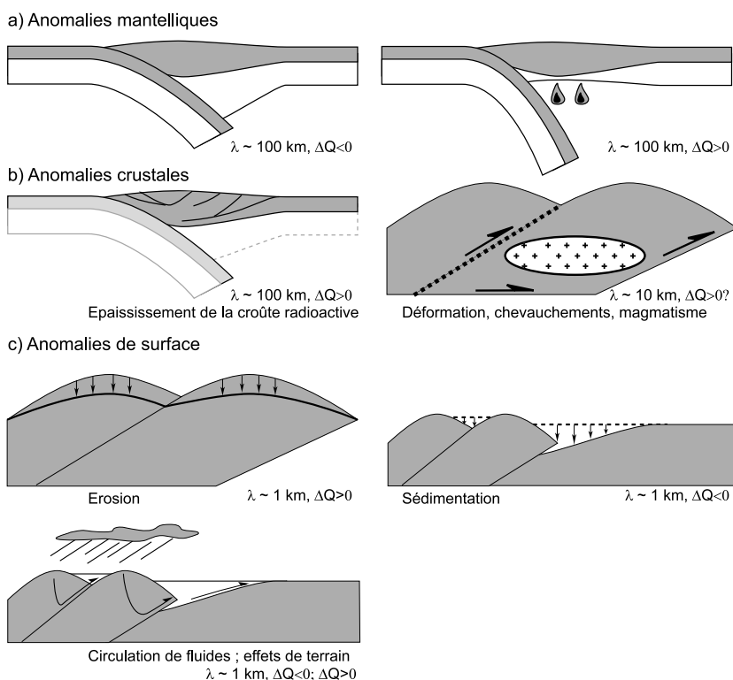
FIG. 1.4.6 – Contrôles géodynamique du régime thermique en domaine orogénique. \Delta Q désigne la polarité de l'anomalie thermique, et \lambda sa longueur d'onde. a) Anomalies mantelliques, lorsque la lithosphère est surépaissie ( \Delta Q < 0 , \lambda > \lambda_{orog} , à droite) ou qu'il y a au contraire délamination de la lithosphère ( \Delta Q > 0 , \lambda > 100 km, à gauche). b) Anomalies crustales : épaissement de la croûte radioactive ( \Delta Q > 0 , \lambda \sim 100 km), déformation ( \Delta Q > 0 , \lambda \sim \lambda_{orog} ), chevauchements ( \Delta Q < 0 ?, \lambda \sim 10 km), friction sur les failles ( \Delta Q > 0 , \lambda \sim 10 km), magmatisme ( \Delta Q > 0 , \lambda variable), c) anomalies de surface : érosion ( \Delta Q > 0 , \lambda \sim 1 km), sédimentation ( \Delta Q < 0 , \lambda \sim 1 km), circulation de fluides ( \Delta Q > 0 dans la chaîne, \Delta Q < 0 dans l'avant-pays, \lambda \sim 1 km.).
