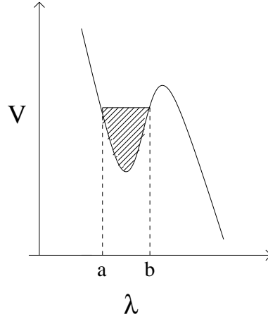
FIG. 3.1 – Distribution des valeurs propres dans un potentiel cubique V(z) = \frac{g}{3}z^3 + \frac{1}{2}z^2 . [a, b] est le support des valeurs propres et V_{eff}(\lambda) est constant le long de [a, b]
