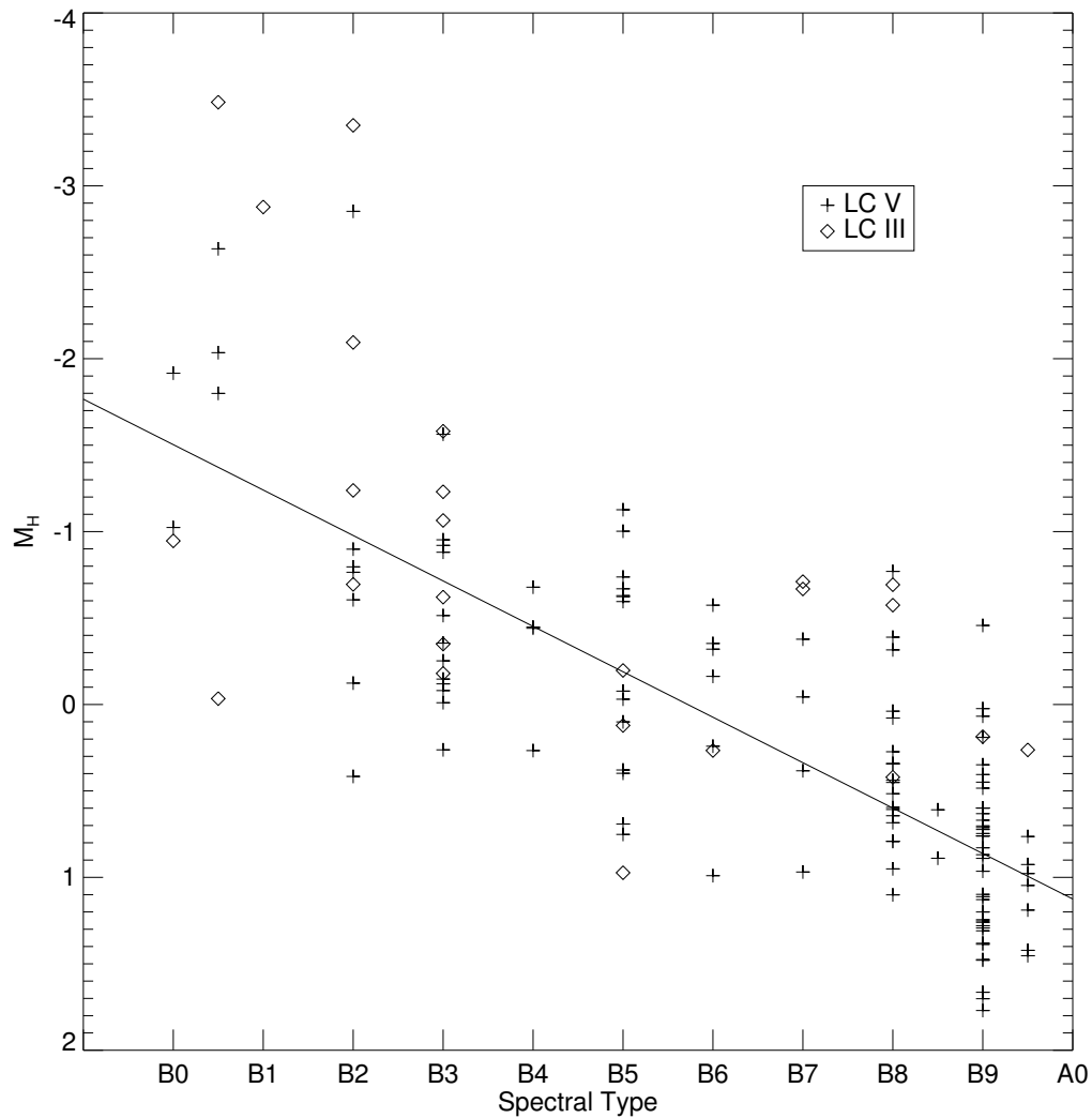
FIGURE 3.5 : Calibration M_H -type spectral pour les 145 étoiles retenues de l'échantillon. Les magnitudes absolues sont calculées en utilisant les distances moyennes aux associations OB, données dans DZ99, ou bien les parallaxes Hipparcos. La droite correspond à un ajustement aux étoiles de CL V.
