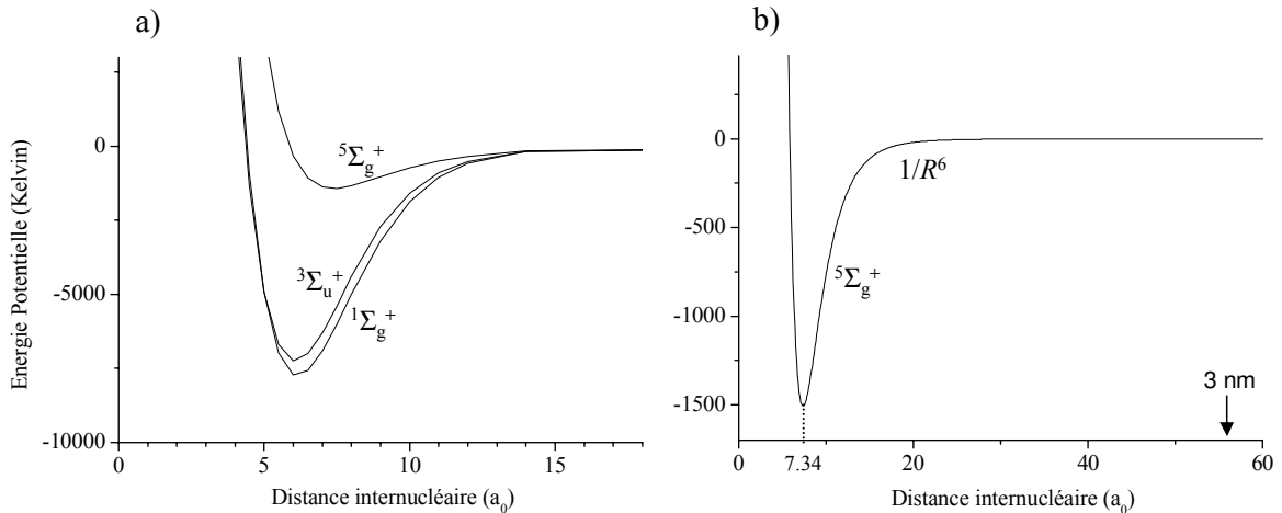
FIG. 4.1 – Potentiels d'interaction intervenant dans une collision entre deux atomes He^* . a) Potentiels tels que publiés par Müller et al. , dans le tableau 3 de la référence [90]. b) Potentiel ^5\Sigma_g^+ , d'après l'expression analytique approchée de Stärck et Meyer [54].
