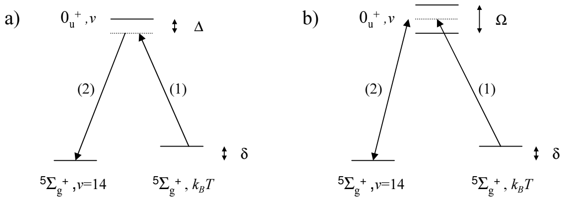
FIG. 9.5 – a) Représentation schématique d'une transition Raman stimulée entre une paire d'atomes He^* dans un état de diffusion à une énergie de collision de l'ordre de k_B T , et la même paire dans l'état lié v = 14 dans le même potentiel électronique ^5\Sigma_g^+ , en passant par un état virtuel désaccordé de \Delta par rapport à un état lié v dans le potentiel à purement longue portée 0_u^+ . b) Représentation schématique de la méthode de photo-association frustrée, avec les trois mêmes états moléculaires. Dans les deux méthodes, la mesure du désaccord \delta conduit à la mesure de l'énergie de liaison de l'état v = 14 .
