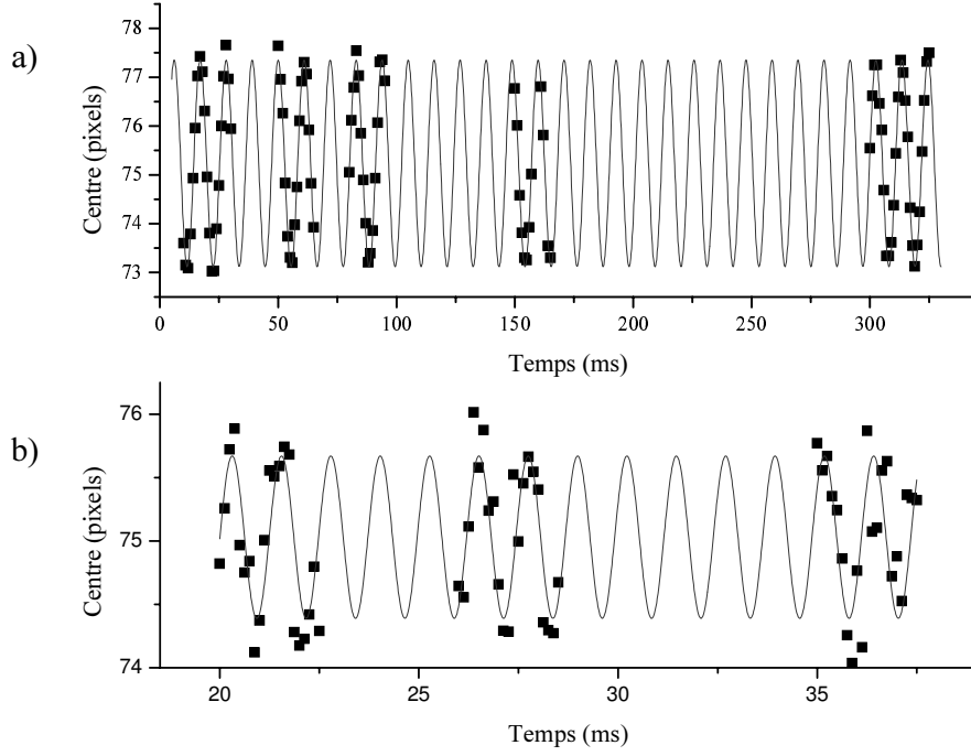
FIG. 2.4 – Oscillations du centre de masse d'un nuage préparé à 5 \mu\text{K} , a) le long de l'axe x (longitudinal): \omega_{\parallel} = 2\pi \times (90.8 \pm 0.1) \text{ Hz} , et b) le long de l'axe y (transverse): \omega_{\perp} = 2\pi \times (805 \pm 2) \text{ Hz}
