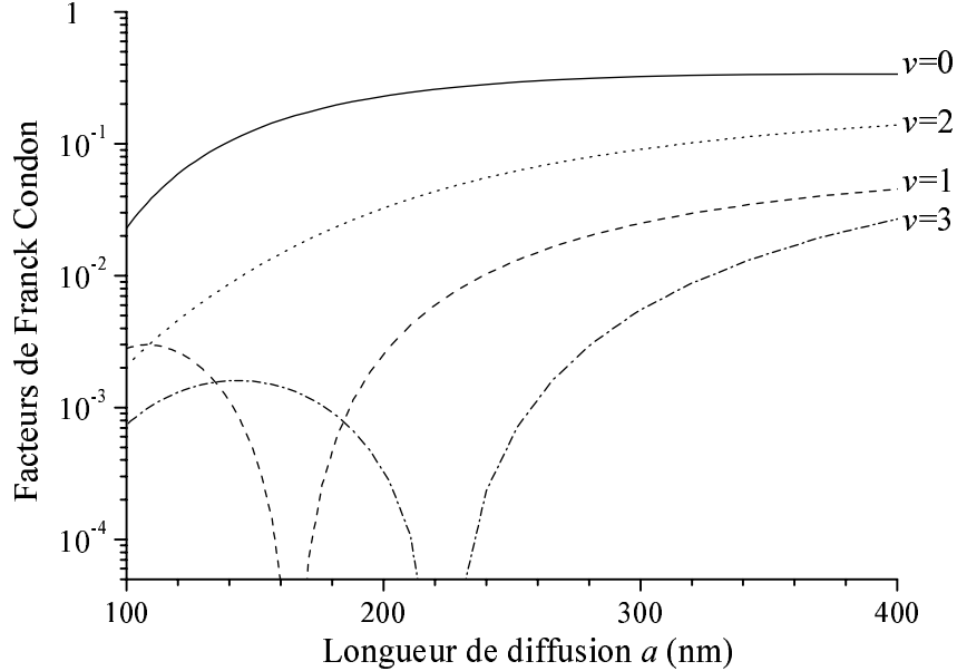
FIG. 9.4 – Calcul des facteurs de Franck Condon entre l'état {}^5\Sigma_g^+ , v = 14 et les états 0_u^+ , v = 0, 1, 2 , et 3. Ces courbes sont obtenues numériquement en calculant le carré de l'intégrale de recouvrement entre les fonctions d'ondes vibrationnelles obtenues au chapitre 7 pour les dimères géants, et la fonction d'onde vibrationnelle v = 14 obtenue à partir du potentiel de Starck et Meyer [54], dont on modifie légèrement la partie externe (en la multipliant par un coefficient proche de 1), pour faire varier la longueur de diffusion.
