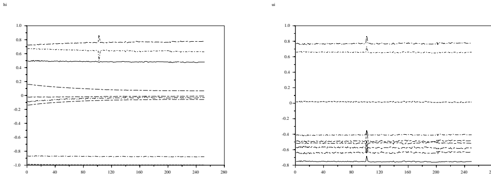
FIG. 3.12: Translation pure : Évolution des coefficients des vecteurs \mathbf{h}_i (gauche) et de ceux des vecteurs \mathbf{u}_i (droite) au cours de l'asservissement.
