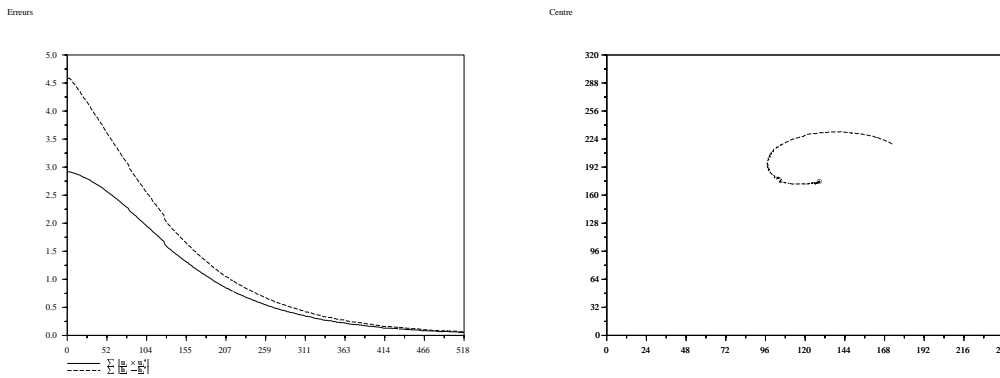
FIG. 3.17: Rotation pure : Évolution des erreurs (gauche) et trajectoire du centre du trièdre dans l'image (droite).
