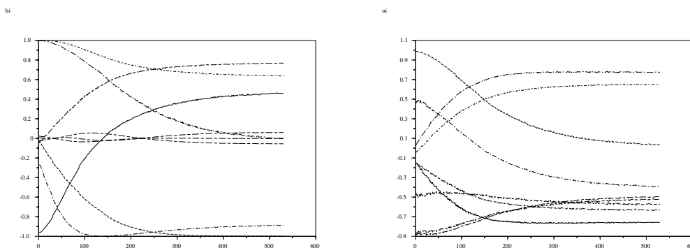
FIG. 3.19: Mouvement complexe : Évolution des coefficients des vecteurs \underline{h}_i (gauche) et de ceux des vecteurs \underline{u}_i (droite) au cours de l'asservissement.
