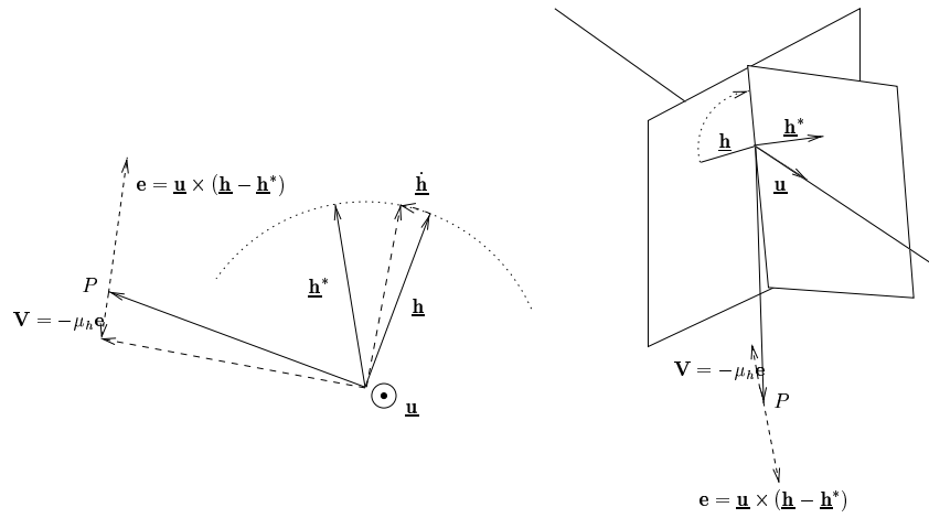
FIG. 2.3: L'effet de la vitesse \mathbf{V} = -\mu_h \underline{\mathbf{u}} \times (\underline{\mathbf{h}} - \underline{\mathbf{h}}^*) : à gauche, dans le cas où \underline{\mathbf{u}} = \underline{\mathbf{u}}^* et à droite, dans le cas contraire.
