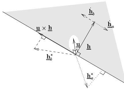
FIG. 2.4: La vitesse \mathbf{V} = -\mu_h \underline{\mathbf{u}} \times (\underline{\mathbf{h}} - \underline{\mathbf{h}}^*) oriente \dot{\underline{\mathbf{h}}} dans le sens du plus court chemin vers \underline{\mathbf{h}}^*
