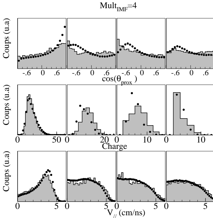
FIG. 6.13 – Distribution du \cos(\theta_{prox}) , de la charge et de la vitesse parallèle du fragment le plus lourd au plus léger (de gauche à droite) pour une cassure à 4 corps.
