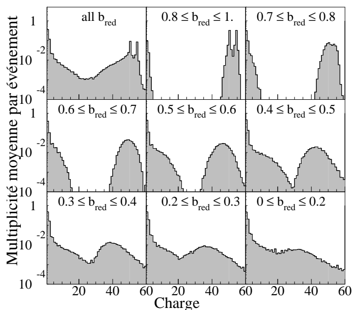
FIG. 4.8 – Distribution de charge avant désexcitation selon le degré de centralité de la collision : haut à gauche tous les événements puis de gauche à droite et de haut en bas les événements de plus en plus centraux. Le système est Xe + Sn à 50 \text{ MeV/u} .
