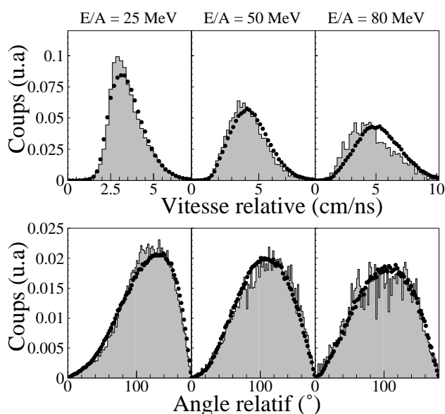
FIG. 5.8 – Distribution des vitesses relatives et angles relatifs pour les trois plus gros fragments pris deux à deux. Le système Xe + Sn aux trois énergies 25, 50 et 80 MeV/u est représenté pour les collisions centrales sélection (c) (en symbole noir les données expérimentales et en continu et fond gris la simulation).
