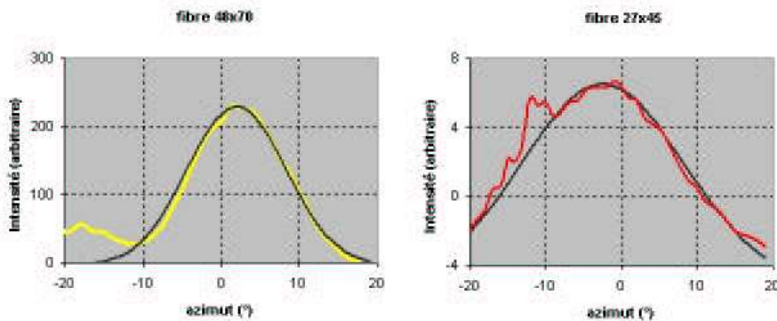
F . 9.6 – Profils d'intensité obtenus lors de la deuxième campagne de mesure. À gauche : fibre de 48 µm de cœur et de 70 µm de gaine. À droite : fibre de 27 µm de cœur et de 45 µm de gaine. Dans chaque cas, on a ajusté une gaussienne par la méthode des moindres carrés.
