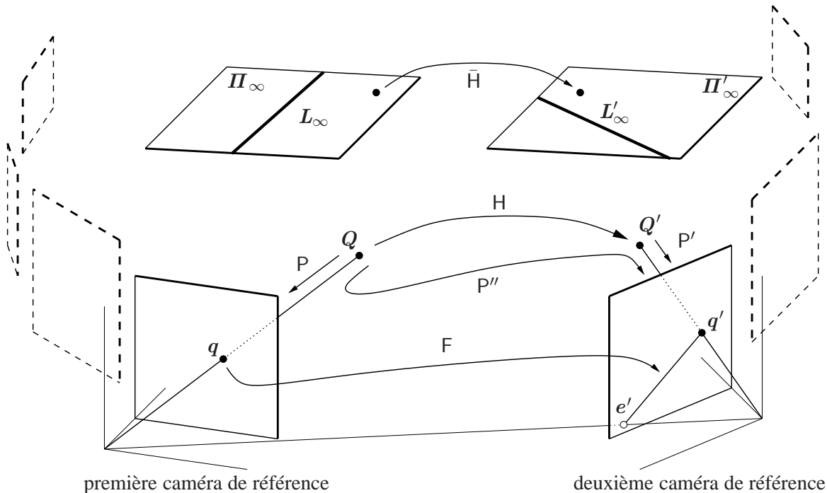
FIG. 7.2 – Le scénario considéré pour l'interprétation géométrique de combinaisons de blocs de la matrice d'homographie pour droites 3D. P \sim \begin{pmatrix} I & \mathbf{0} \end{pmatrix} est la matrice de projection de la première caméra de référence et P' \sim \begin{pmatrix} I & \mathbf{0} \end{pmatrix} de la deuxième caméra de référence, chacune exprimée dans la base de reconstruction qui lui est propre. P'' \sim P'H est la matrice de projection de la deuxième caméra de référence, exprimée dans la première base.
