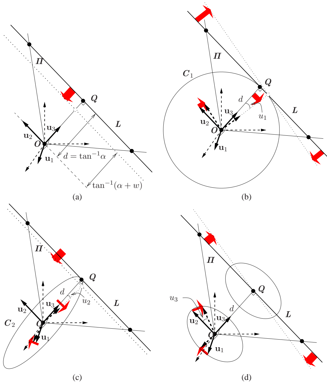
FIG. 6.3 – Interprétation géométrique de la mise à jour de la représentation orthonormale ( U = (\mathbf{u}_1 \ \mathbf{u}_2 \ \mathbf{u}_3), W = R_{2D}(\alpha) ) d'une droite 3D L selon le schéma de mise à jour (6.13) de paramètres \mathbf{x}^T = (u_1 \ u_2 \ u_3 \ w) . Les flèches rouges indiquent le mouvement subi par la droite. (a) : le paramètre w modifie la distance entre L et O ( L est traduite dans le plan \Pi parallèlement à elle-même). (b) : le paramètre u_1 provoque une rotation d'angle u_1 de L autour du cercle C_1 de centre O , de rayon d et contenu dans le plan \Pi . (c) : le paramètre u_2 provoque une rotation d'angle u_2 de L autour du cercle C_2 de centre O , de rayon d et contenu dans le plan défini par \mathbf{u}_1 et \mathbf{u}_3 . (d) : le paramètre u_3 provoque une rotation d'angle u_3 de L autour de l'axe défini par les points O et Q .
