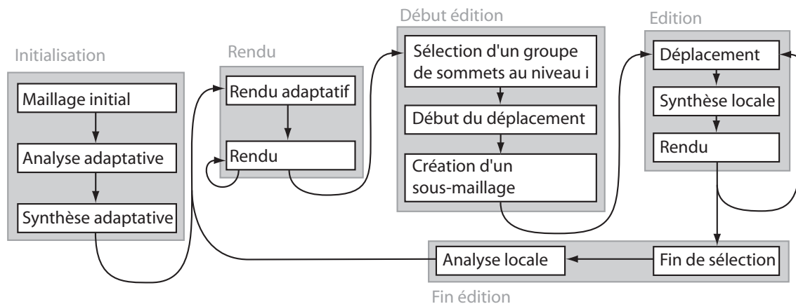
FIG. 1.51: Diagramme de fonctionnement du système d'édition multirésolution interactif proposé par [ZSS97].
