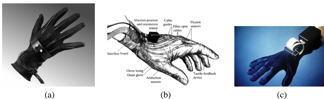
FIG. 1.91: Le VPL-Dataglove (a) et son schéma (b) (images extraites de [Kal93]). (c) le 5th glove de General Reality (image extraite de www.genreality.com ).
