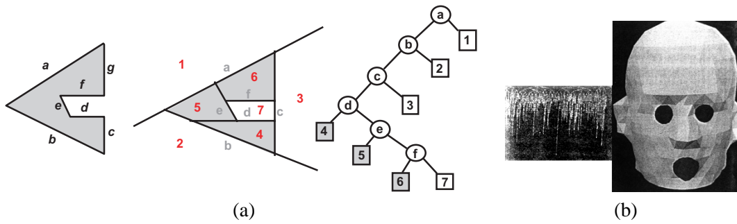
FIG. 1.3: (a) exemple de partitionnement d'un polygone, avec l'arbre correspondant, (b) exemple de modèle construit avec le système avec, à gauche, une évocation de l'arborescence correspondante (figure extraite de [Nay90]).
