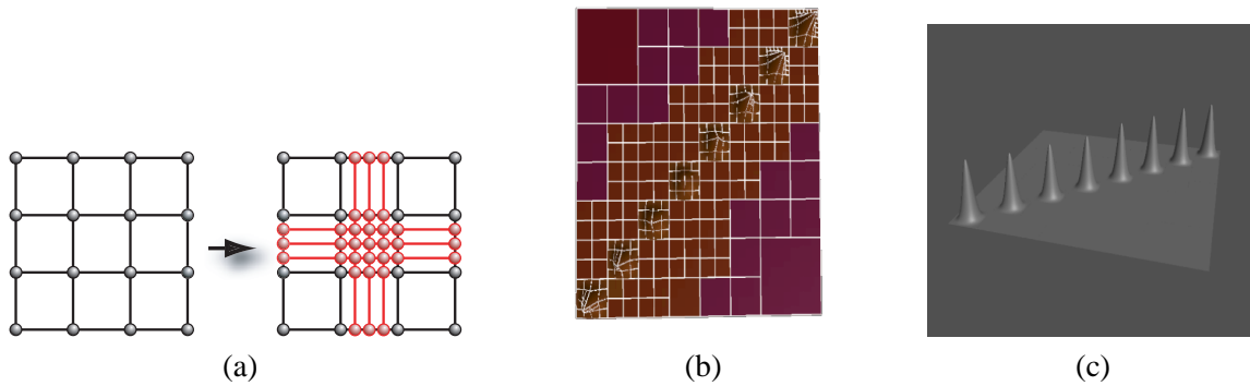
FIG. 1.9: (a). Raffinement classique d'un carreaux paramétrique : la subdivision du carreau central entraîne celle des deux domaines de paramètres adjacents. (b) et (c) en subdivisant les carreaux situés sur la diagonale, tous les domaines seraient inutilement subdivisés (cas le pire), ce que les overlays de [FB88] évitent (images extraites de la page web de D. Forsey).
