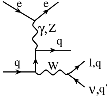
FIG. 1.12 – Diagramme de production de boson vecteur W .
