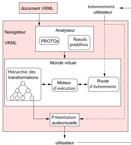
FIG. 2.13 – Structure générale d'un navigateur VRML
