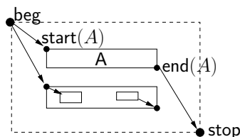
FIG. 4.2 – Description générale d'un opérateur
