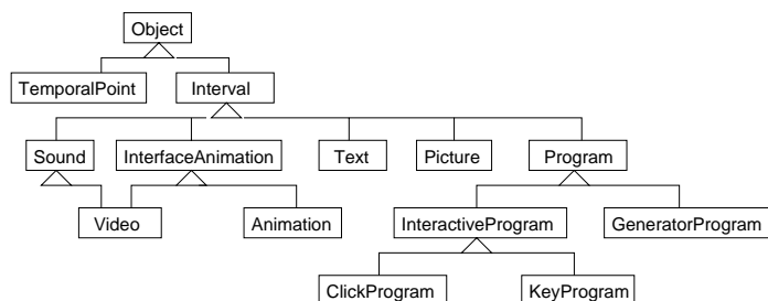
FIG. 4.1 – Hiérarchie des objets primitifs TAO
