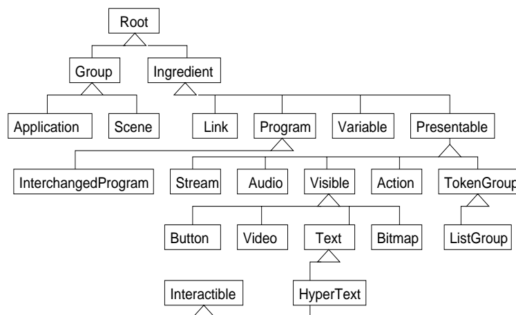
FIG. 3.5 – Hiérarchie des objets MHEG
