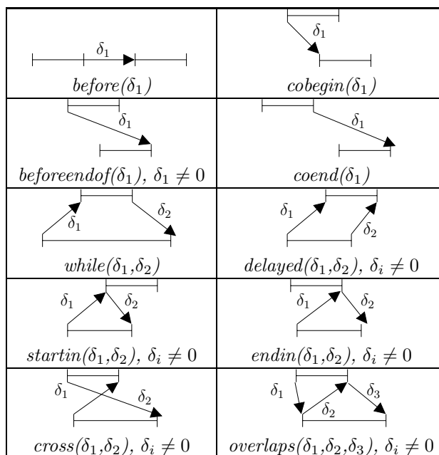
FIG. 3.2 – Les relations de Wahl-Rothermel
