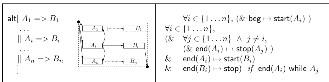
FIG. 4.5 – Opérateur TAO alternatif
