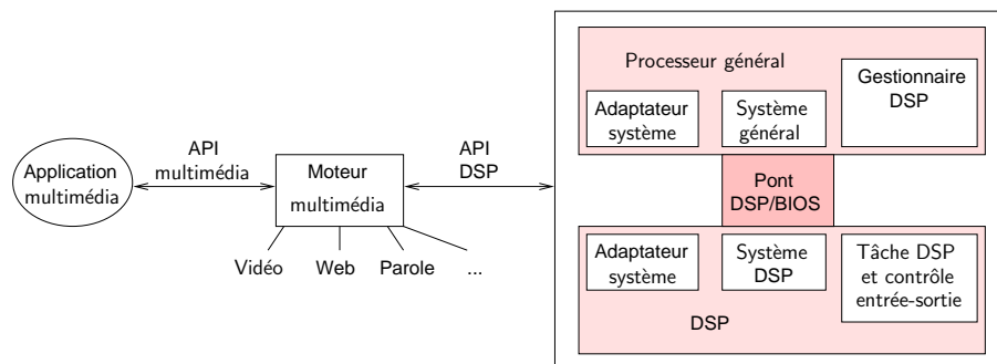
FIG. 2.6 – Plate-forme OMAP TM
