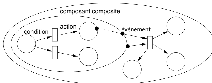
FIG. 3.3 – Modèle de connecteurs hypermédias
