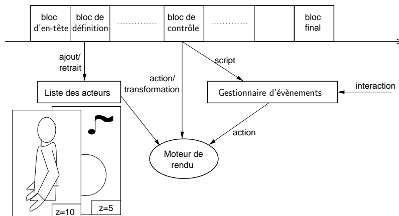
FIG. 2.9 – Structure du format Flash
