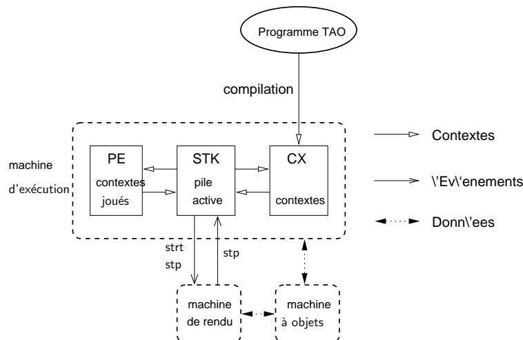
FIG. 5.2 – Schéma de la machine de présentation
