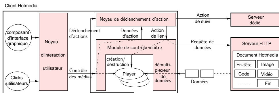
FIG. 2.11 – Architecture de la plate-forme Hotmedia
