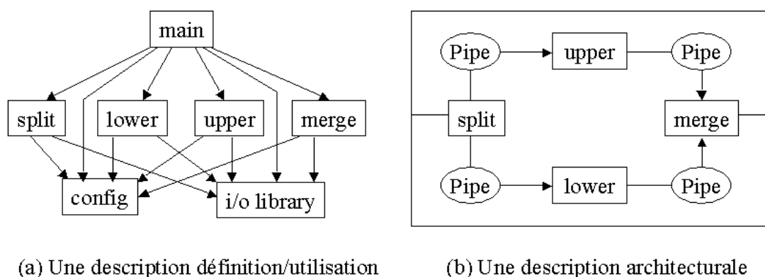
FIG. 4.1 – Description définition/utilisation vs Description architecturale
