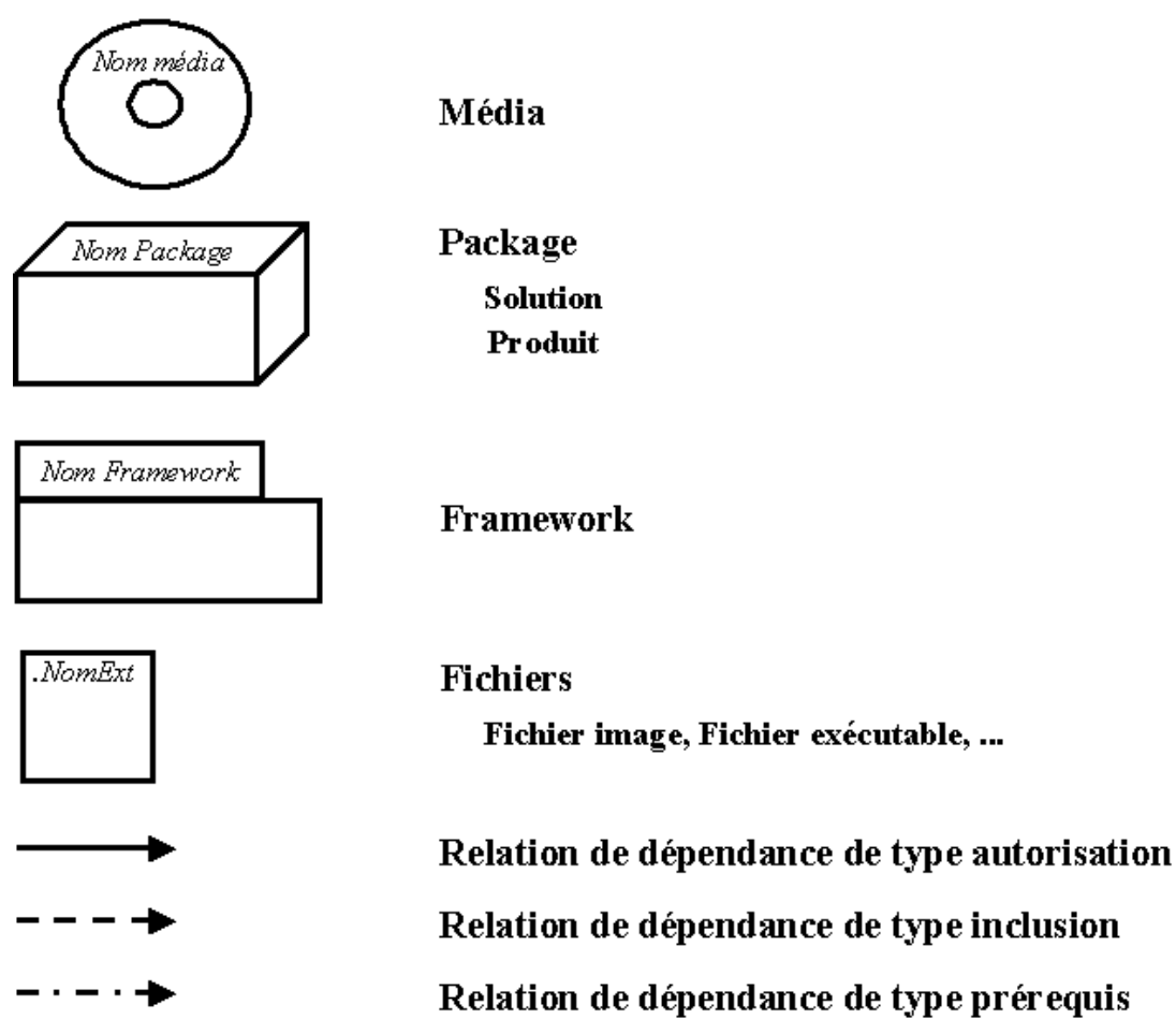
FIG. E.7 – Syntaxe graphique pour l'architecture produit
