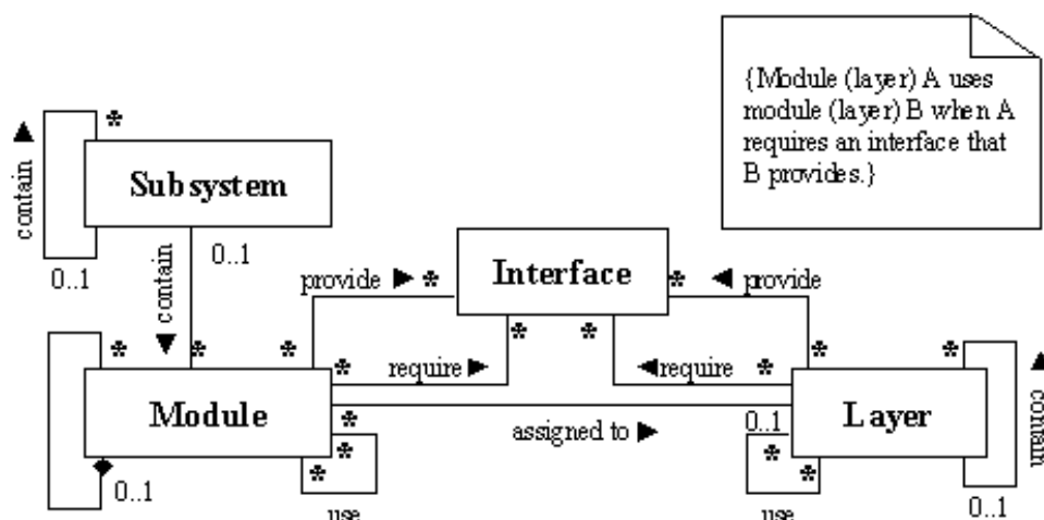
FIG. D.3 – Méta-modèle de la vue module
