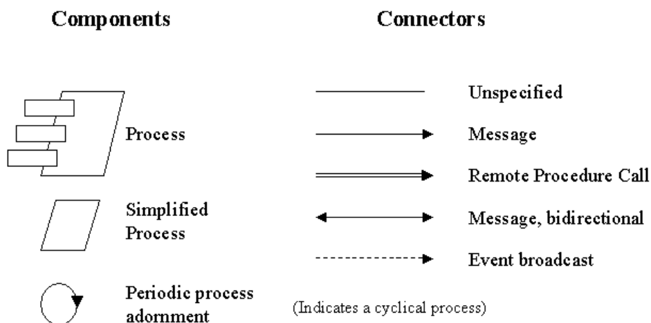
FIG. C.3 – Notation pour la vue processus
