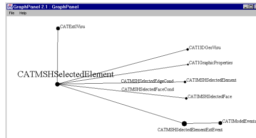
(d) GraphPanel
