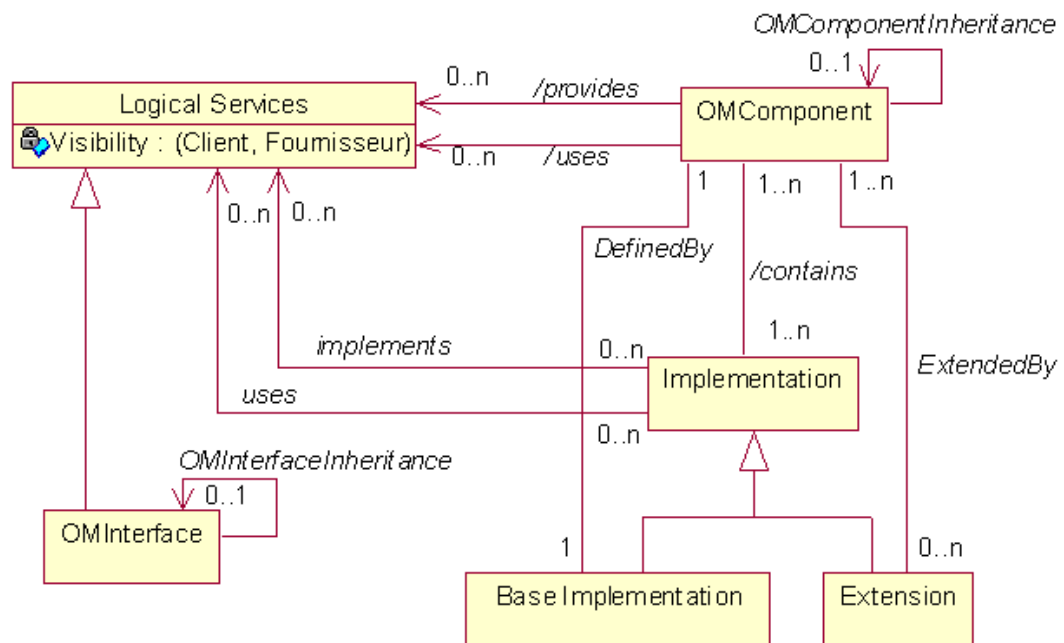
FIG. E.2 – Le méta-modèle de l'Object Modeler
