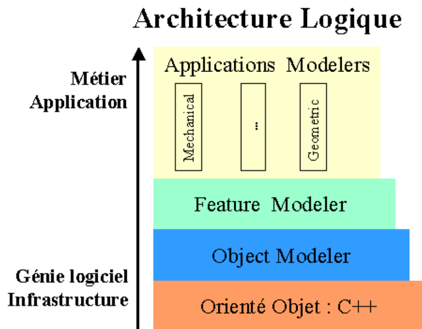
FIG. 6.1 – Les modeleurs de l'architecture logique
