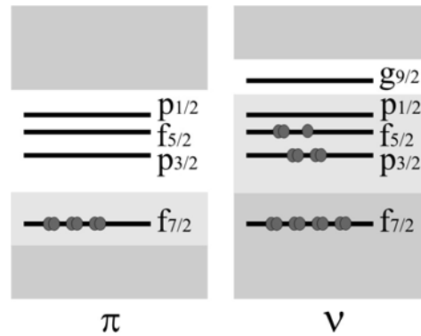
Figure 3.2.21. Espace de valence utilisé pour le calcul du facteur g du ^{61\text{m}}\text{Fe} . En gris foncé, espace extérieur qui ne contribue pas dans la construction de la fonction d'onde, en gris clair espace à partir duquel nous permettons un nombre total limité t d'excitations vers ( p_{3/2} , f_{5/2} , p_{1/2} ) pour les protons et vers g_{9/2} pour les neutrons.
