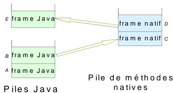
Figure 2-11. Piles d’un thread invoquant des méthodes Java et des méthodes natives
