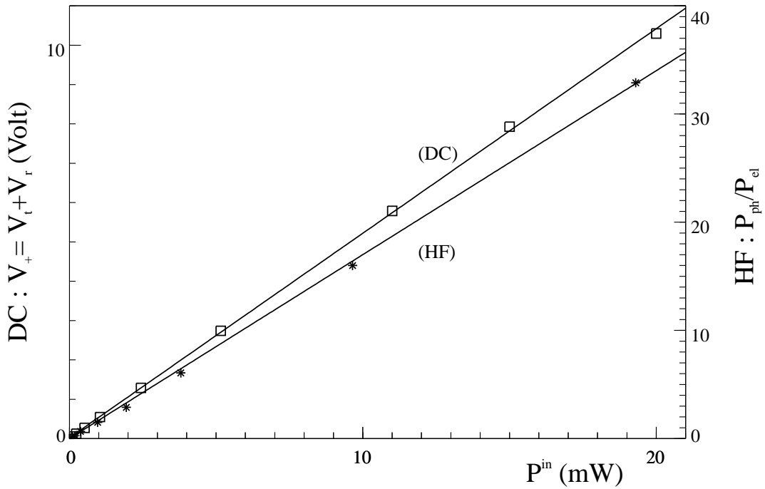
Fig. 69: Caractéristique puissance-tension du dispositif de détection équilibré. La droite ( DC ) décrit le comportement de la tension V_+ qui est égale à la somme des tensions à la sortie des voies DC des deux détecteurs. La droite ( HF ) représente le rapport des puissances de bruit de photon P_{ph} et de bruit électronique P_{el} à une fréquence d'analyse de 2\text{ MHz}
