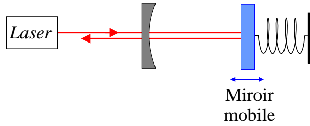
Fig. 6: Cavité Fabry Perot à miroir mobile
