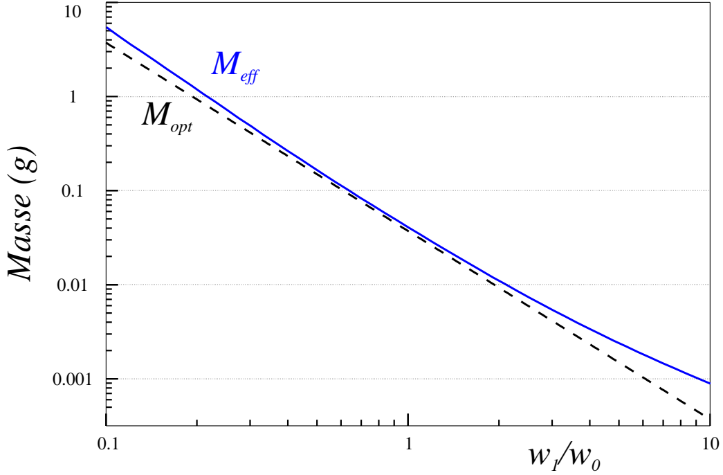
Fig. 29: Variation des masses effective et optimale en fonction du col du faisceau lumineux
