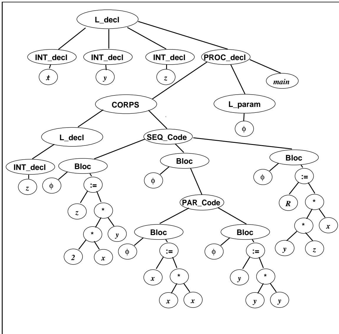
Figure 4.6: Arbre syntaxique produit par l'analyseur
