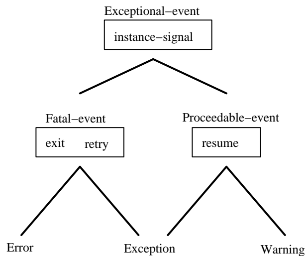
Fig. 4.4 : hiérarchie d'exceptions
