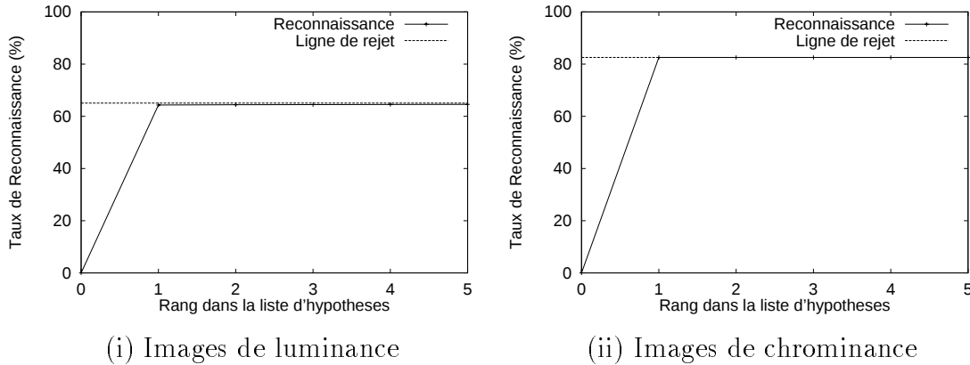
FIG. 3.5 – Évaluation de la reconnaissance par une imagerie issue de la base d'apprentissage. Les graphes présentent le pourcentage de points reconnus aux rangs 1 et 5. 20 à 30 % d'images au dessus de la "ligne de rejet" correspondent au cas [c] (trop d'images similaires).
