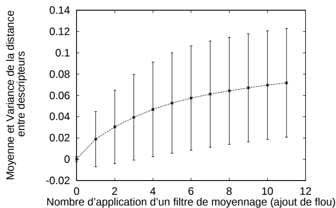
FIG. 4.5 – Stabilité par rapport à un bruit de flou. Ce graphe montre l’évolution de la distance entre vecteurs de mesures se correspondant par rapport à un flou croissant (simulation d’une mauvaise mise au point de la caméra). Cette évolution est visualisée par sa moyenne et son écart-type.
