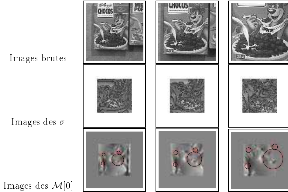
FIG. 3.17 – (1) Images brutes , (2) Images des \sigma sélectionnées (ces valeurs correspondent aux maxima du Laplacien normalisé) et (3) Quelques correspondances visualisées sur \mathcal{M}[0] (la dérivées premières après réglage de l'échelle) .
