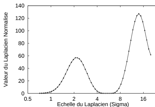
FIG. 3.18 – Exemple de détection de maxima du Laplacien Normalisé. Cet exemple montre un point où deux maxima sont disponibles et donc deux échelles caractéristiques. Les cercles sont tracés en prenant pour centre le point évalué et pour rayon 2\sigma avec \sigma les paramètres d'échelles sélectionnés.
