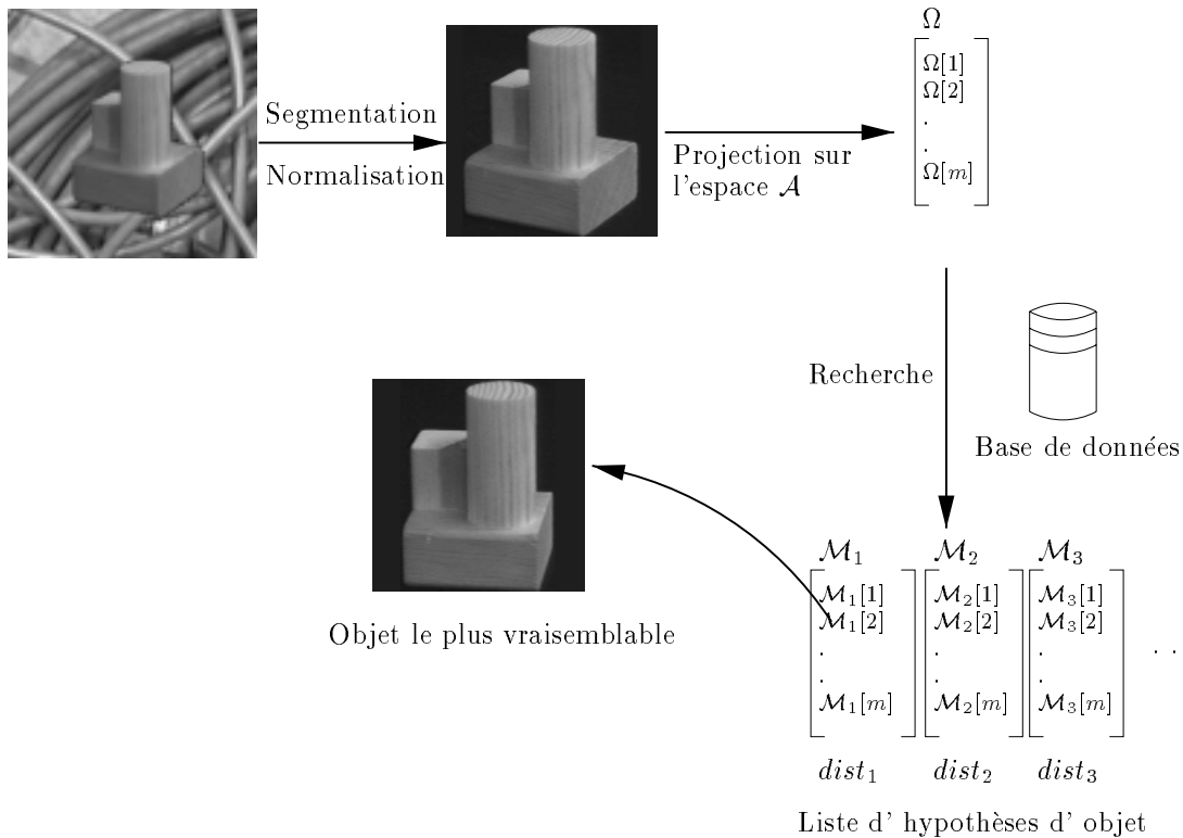
FIG. 2.3 – Reconnaissance d'une image. Ce schéma illustre la stratégie de reconnaissance d'objets proposée par MURASE et NAYAR . Une image de la scène est capturée, puis l'objet contenue dans celle-ci est segmenté puis normalisé en taille. L'image obtenue est projetée sur l'espace de description \mathcal{A} . Le vecteur \Omega obtenu est recherché dans la base de modèles. Les vecteurs \mathcal{M}_k des variétés les plus proches sont appariés à ce vecteur. La distance dist_k entre \Omega et \mathcal{M}_k donne un indice de confiance sur les appariements. Sur l'exemple, le vecteur \mathcal{M}_1 correspond à une hypothèse d'image modèle correcte.
