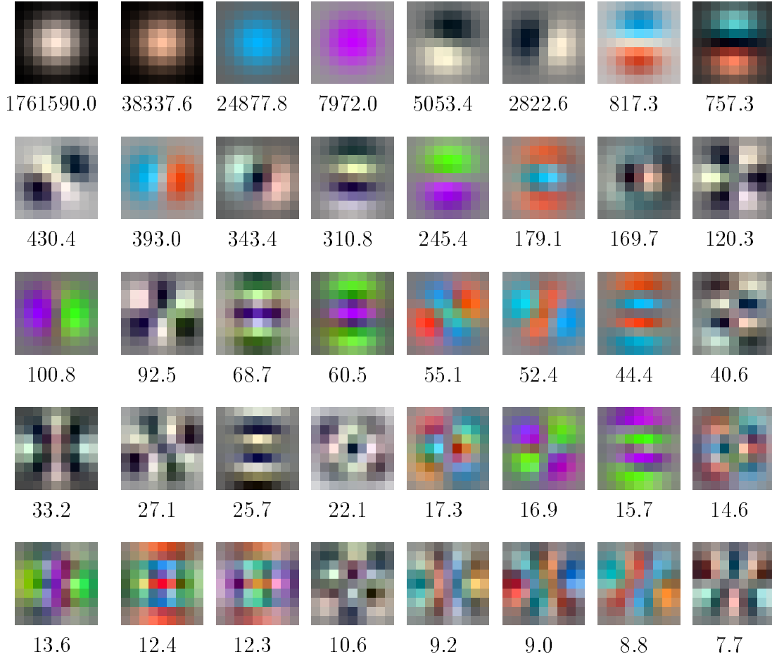
FIG. 3.4 – Vecteurs Propres et Valeurs Propres associées.
