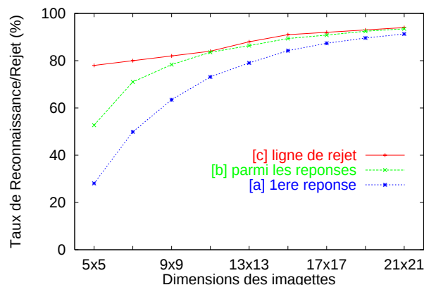
FIG. 3.7 – Évaluation de l'influence de la taille des fenêtres sur la reconnaissance par une imagerie quelconque de la base de test. La reconnaissance augmente avec la taille de l'imagette mais la localité de l'approche diminue avec l'augmentation de la taille. Un compromis peut être choisi autour de 10 \times 10 .
