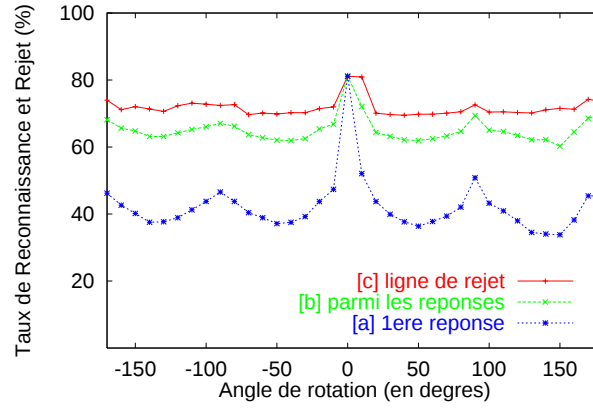
FIG. 3.13 – Évaluation expérimentale de la reconnaissance en fonction de l'angle de vue avec détection automatique de l'orientation local en chaque point. Ce graphe montre 25% d'imagettes rejetées en moyenne et moins de 5% de faux appariements. Le rejet important s'explique par la présence de nombreuses imagettes de niveau de gris constant.
