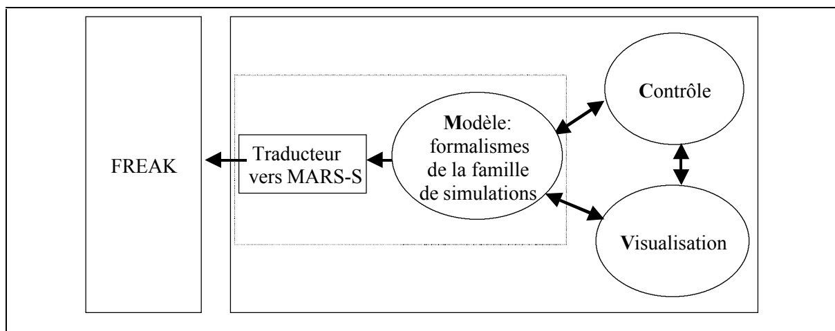
Figure 6-7 Architecture d'une application du sous-framework du domaine
