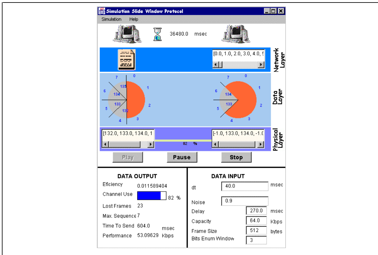
Figure 8-9: SimSlide : Simulation d'un protocole de fenêtre glissante
