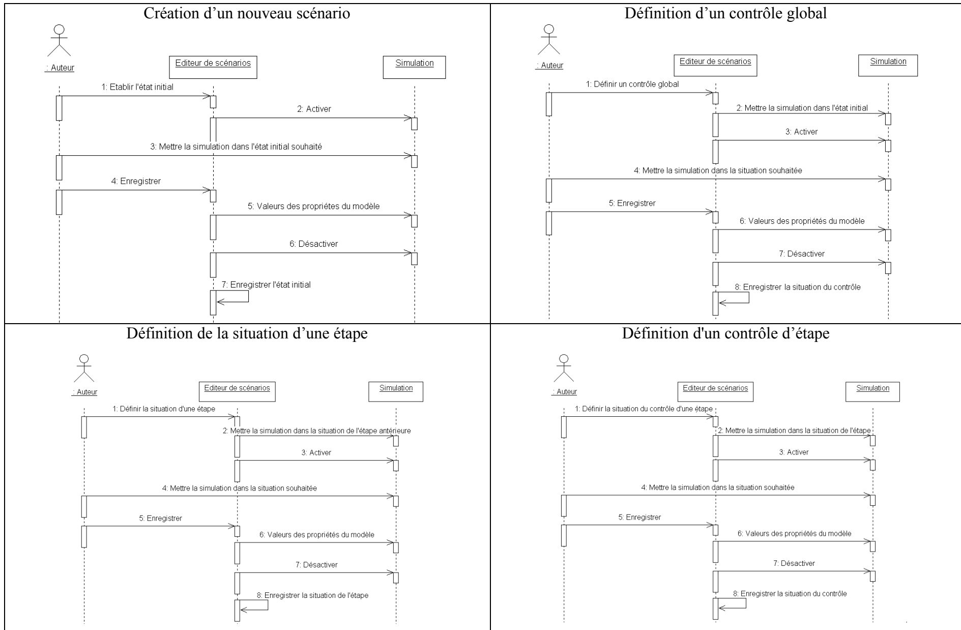
Figure 7-4: Diagrammes de séquence pour la définition de situations en OASIS
