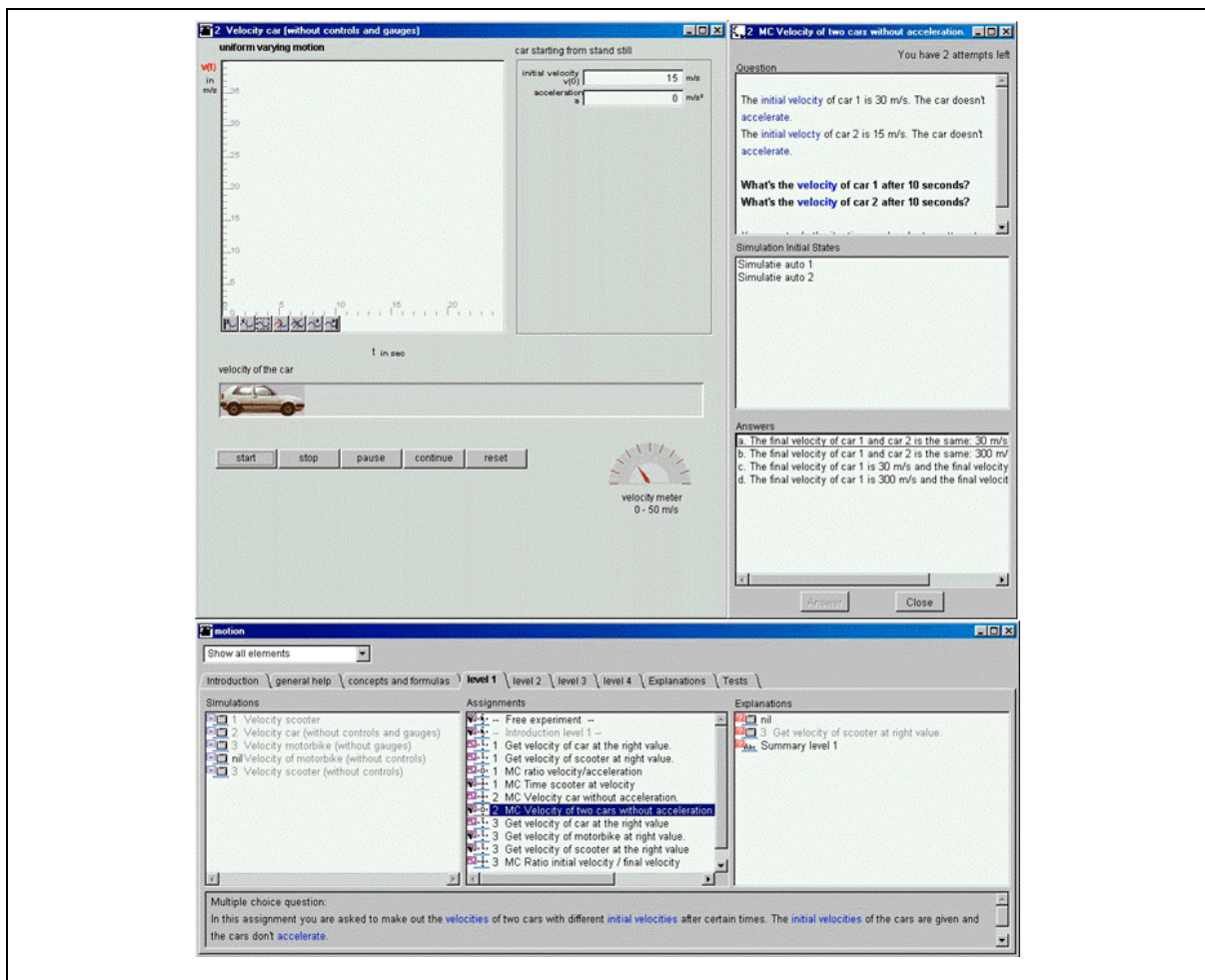
Figure 3-9: Environnement Apprenant de SimQuest (D'après [SER 99])
