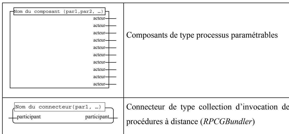
Figure 8-2: Notations graphiques pour les extensions de paramétrage
