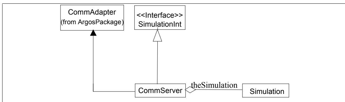
Figure 8-11: Schéma de classes du serveur de simulation
