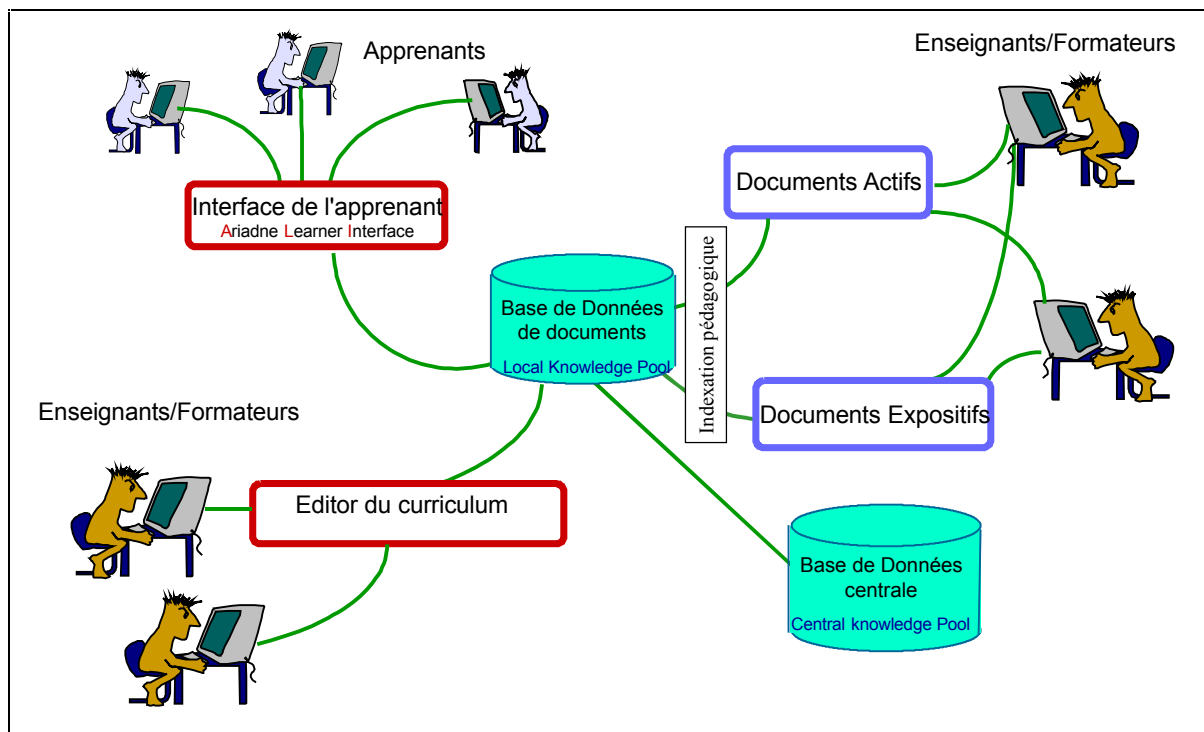
Figure 4-3: Schéma du projet ARIADNE
