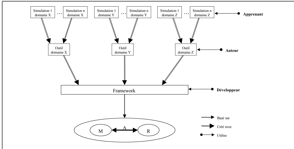
Figure 6-1: Objectif du framework
