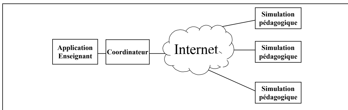
Figure 8-7: La séance de TD virtuel
