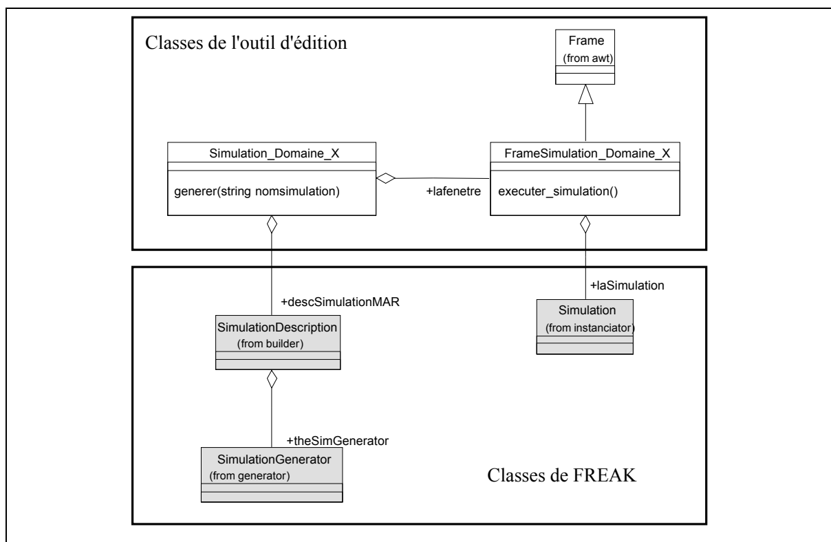
Figure 6-9: Exemple d'utilisation de la partie stable
