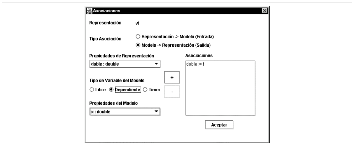
Figure 6-15: Interfaces pour la définition d'associations de FENIX
