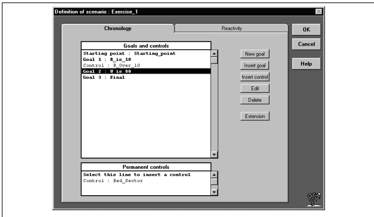
Figure 3-10: Editeur de scénarios d'OASIS
