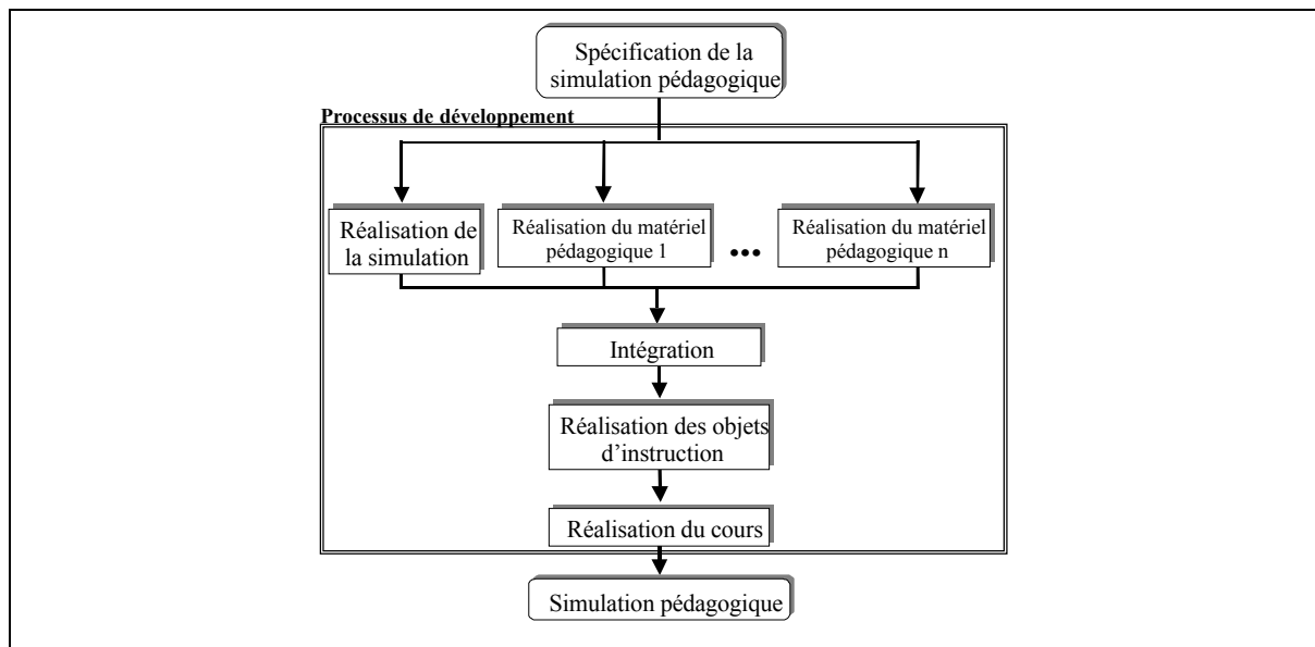
Figure 2-2: Processus de développement avec SAM
