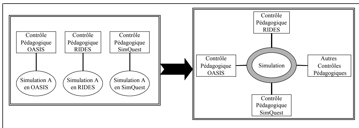
Figure 3-12: Indépendance de l'espace scénario et du système de simulation
