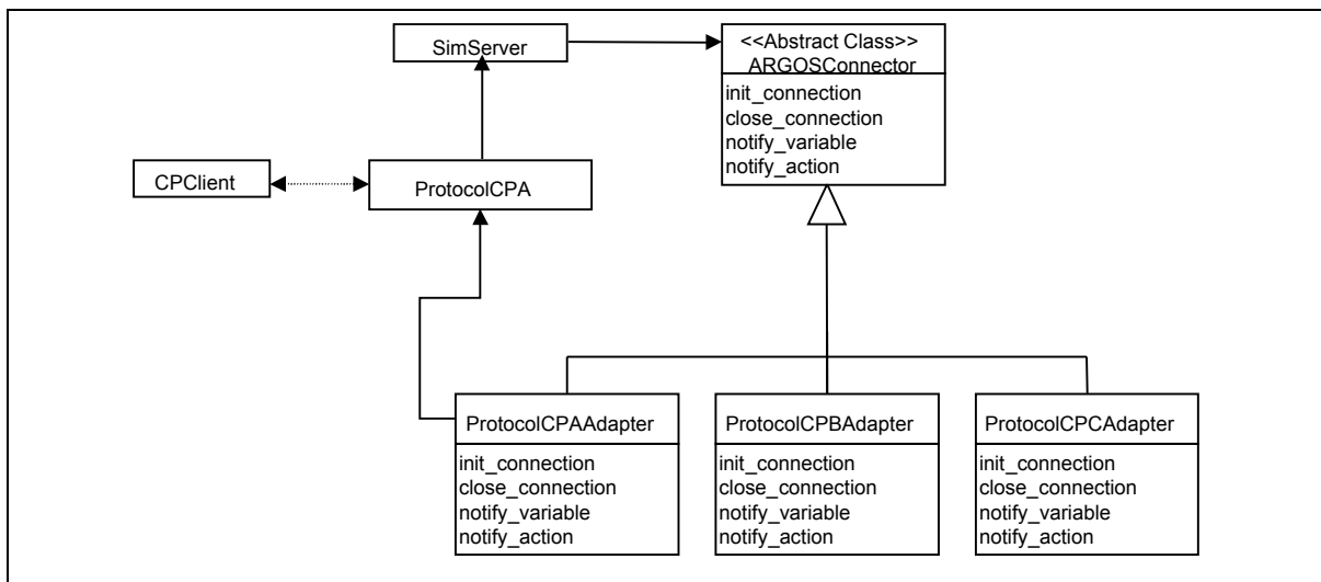
Figure 8-6: Schéma de classes du connecteur ARGOSConnector
