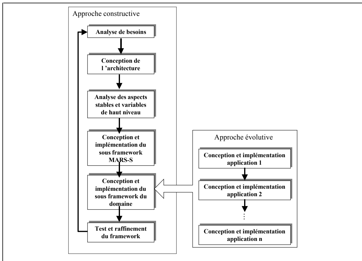
Figure 6-4: Processus de développement du framework
