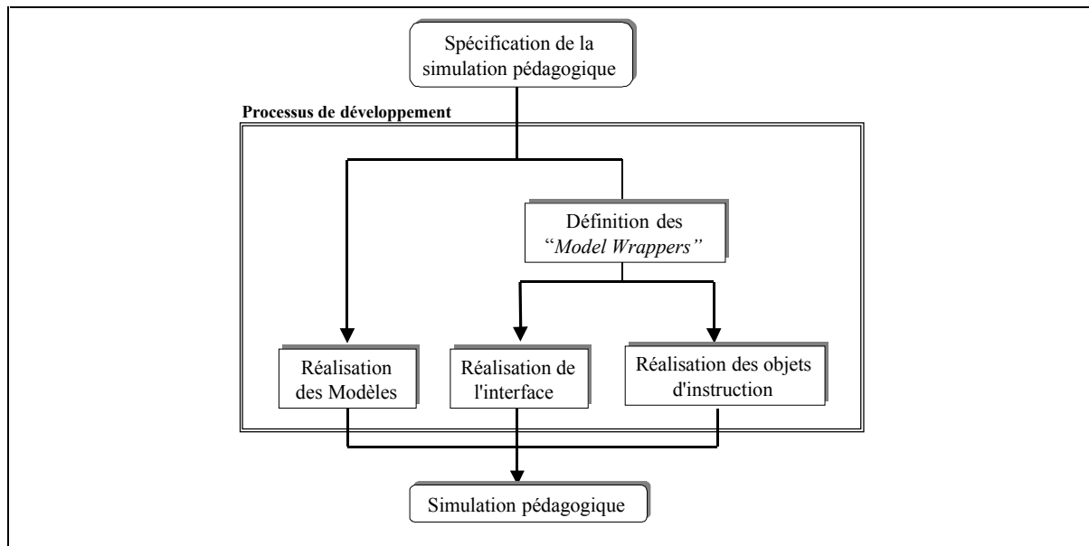
Figure 2-7: Processus de développement avec SimQuest
