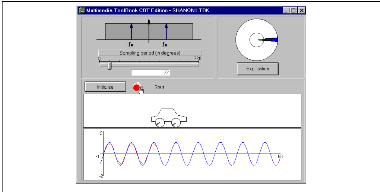
Figure 4-6: Interface de la simulation du Théorème de Shannon
