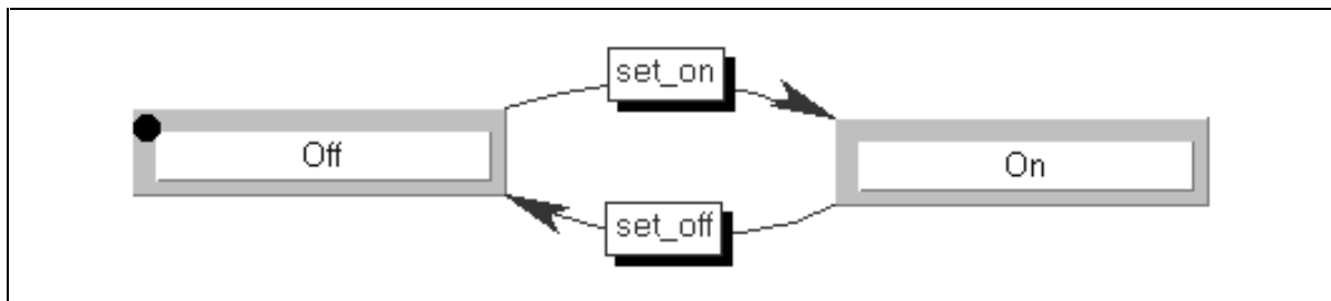
Figure 6-3: Graphe d'états et de transitions de la simulation
