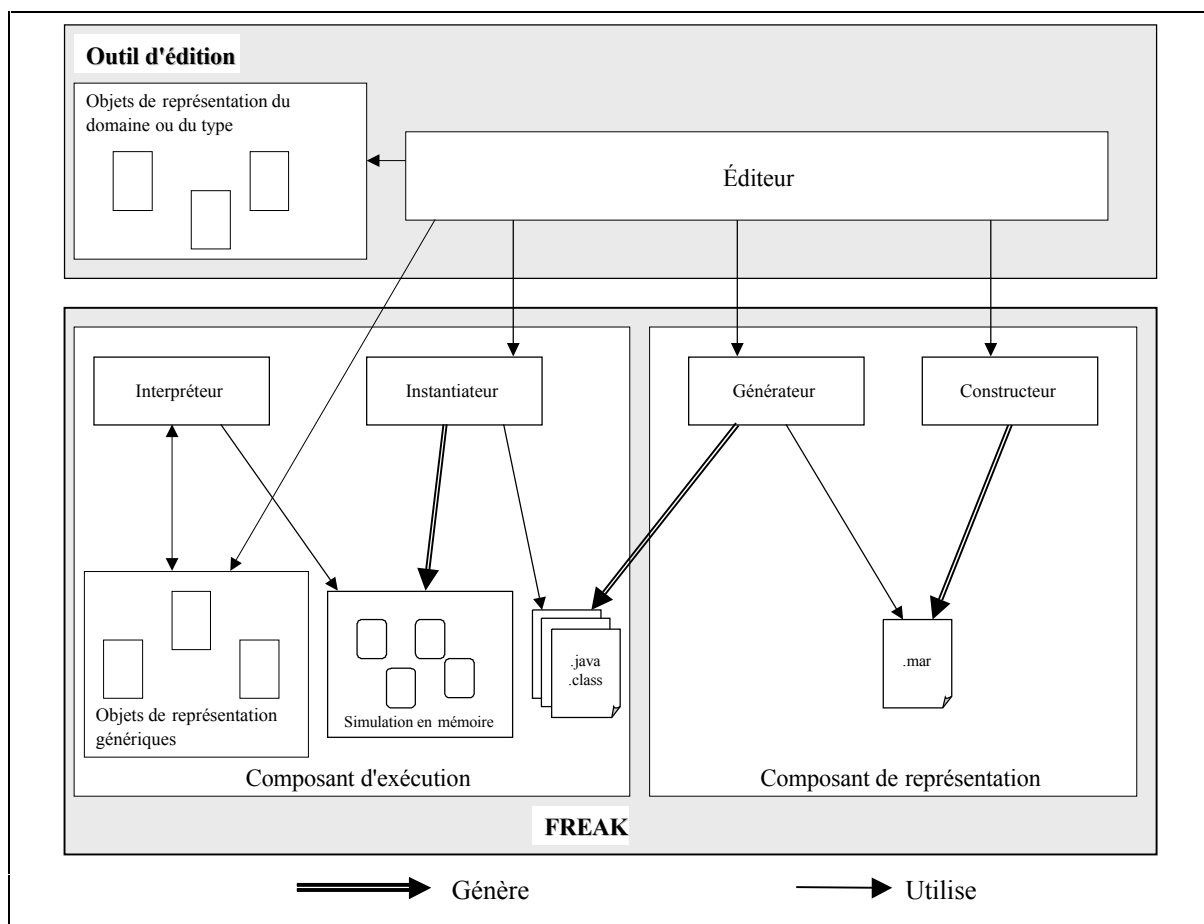
Figure 6-6: Architecture générale du framework
