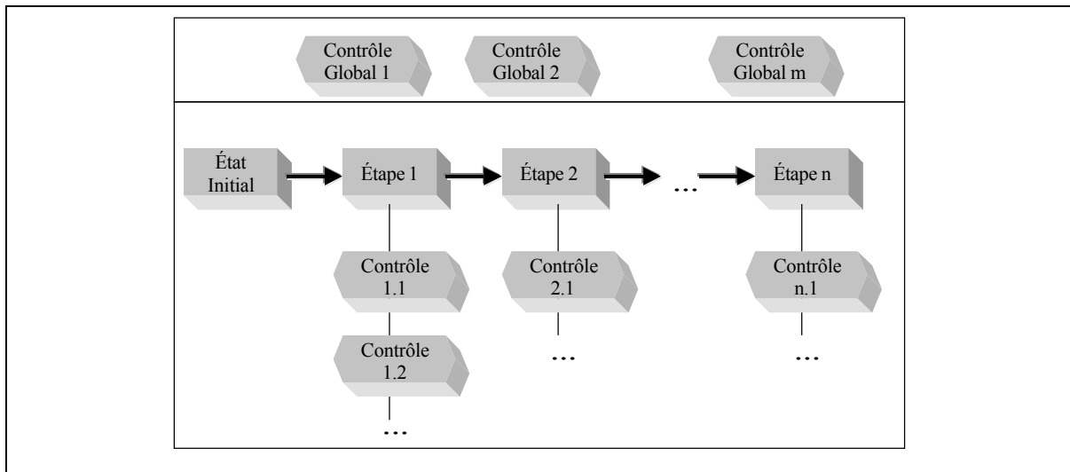
Figure 3-2: Scénario de contrôle pédagogique d'OASIS
