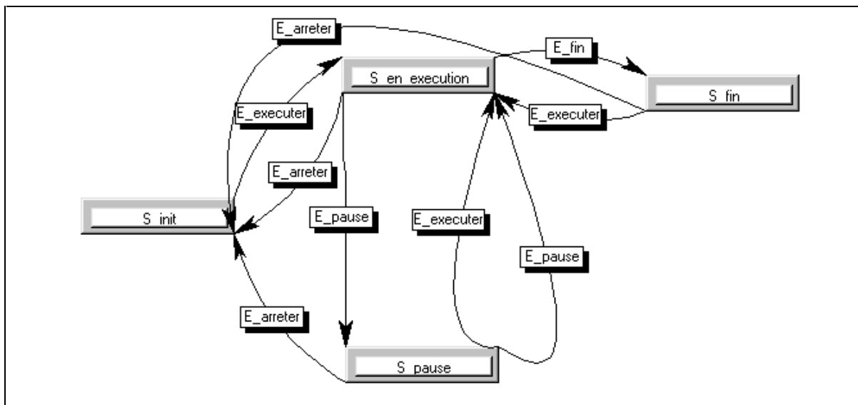
Figure 6-13: Graphe d'état des simulations en FENIX
