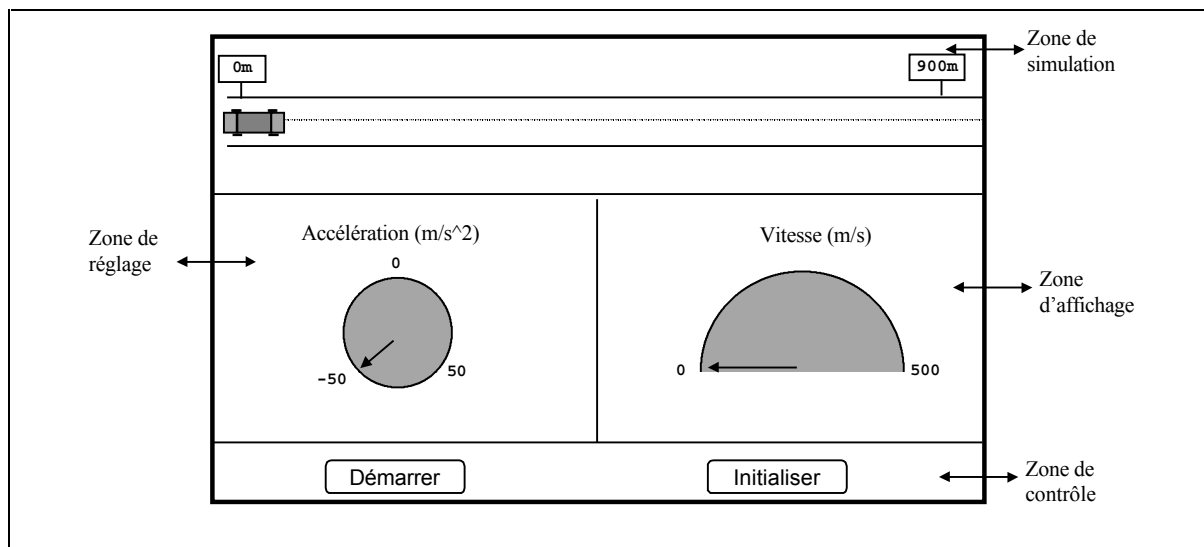
Figure 6-2: Maquette de l'interface de la simulation
