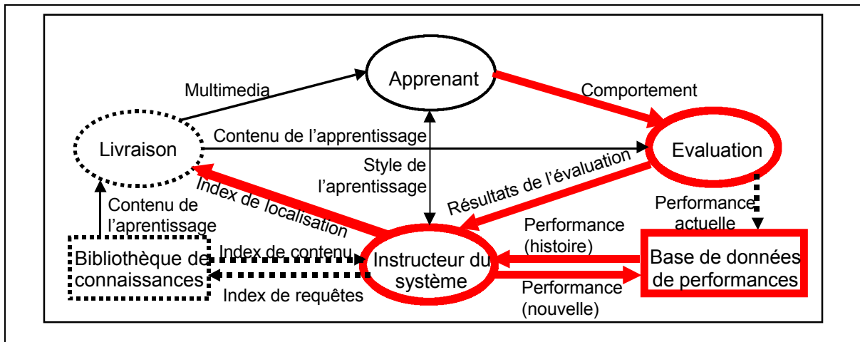
Figure 7-2: Aspects de l'architecture LTSA concernant le groupe Communication Outil/Agent
