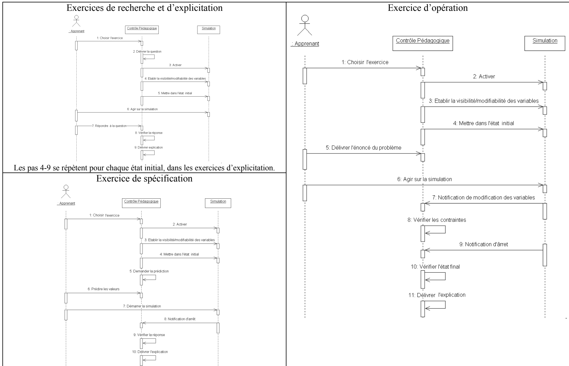
Figure 7-6: Diagrammes d'interaction en exécution des composants d'instruction de SimQuest
