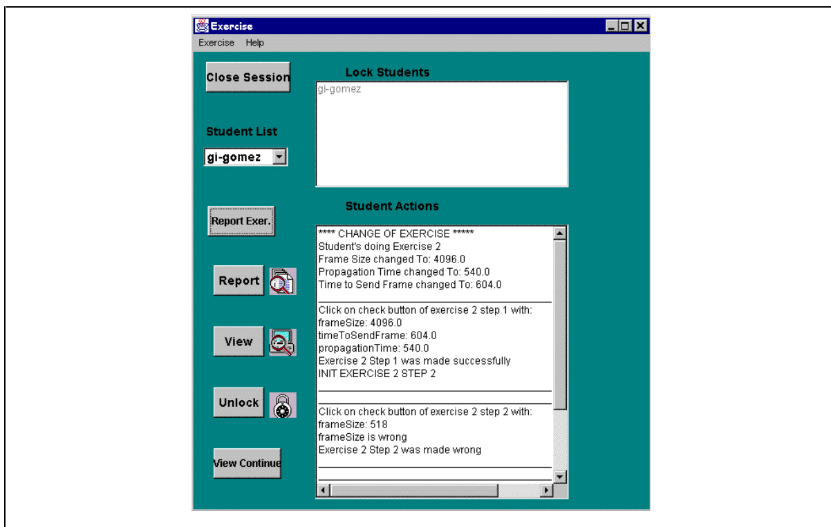
Figure 8-8: Interface de l'enseignant dans le TD à distance
