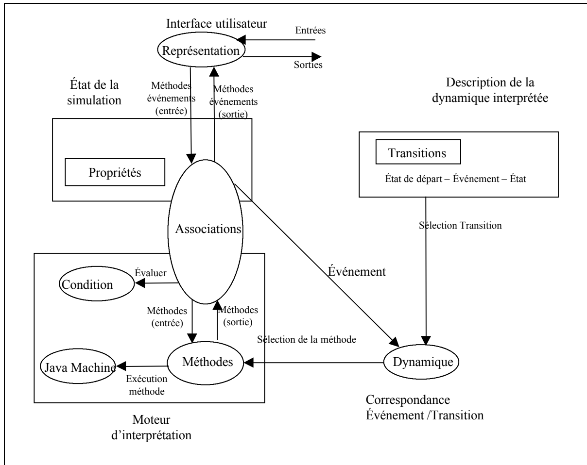
Figure 6-8 Architecture de l'interpréteur de simulations MARS-S
