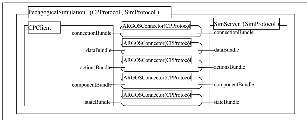
Figure 8-3: Diagramme général d'ARGOS
