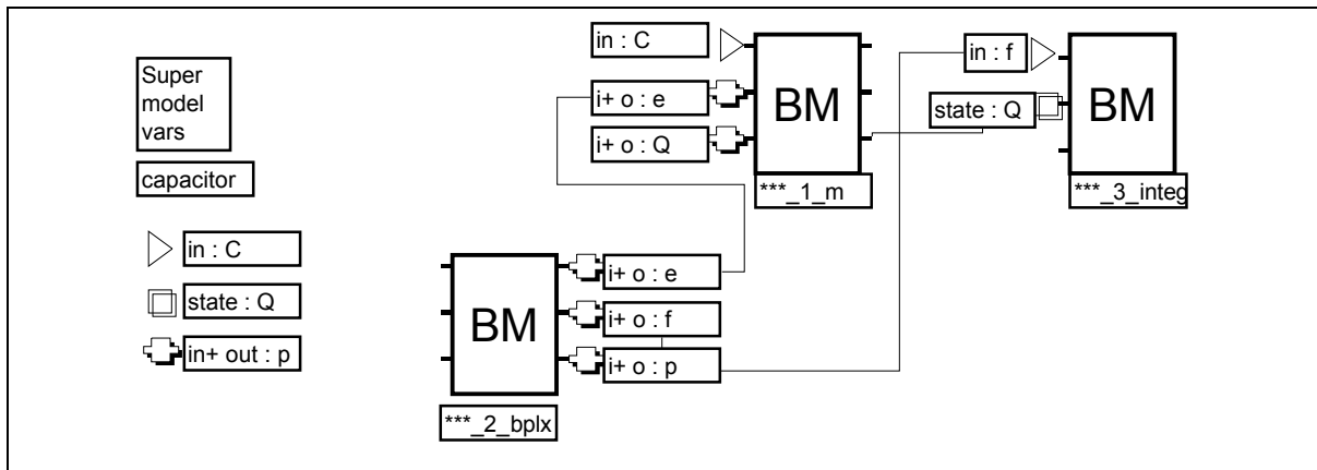
Figure 2-10: Exemple d'un modèle en SimQuest
