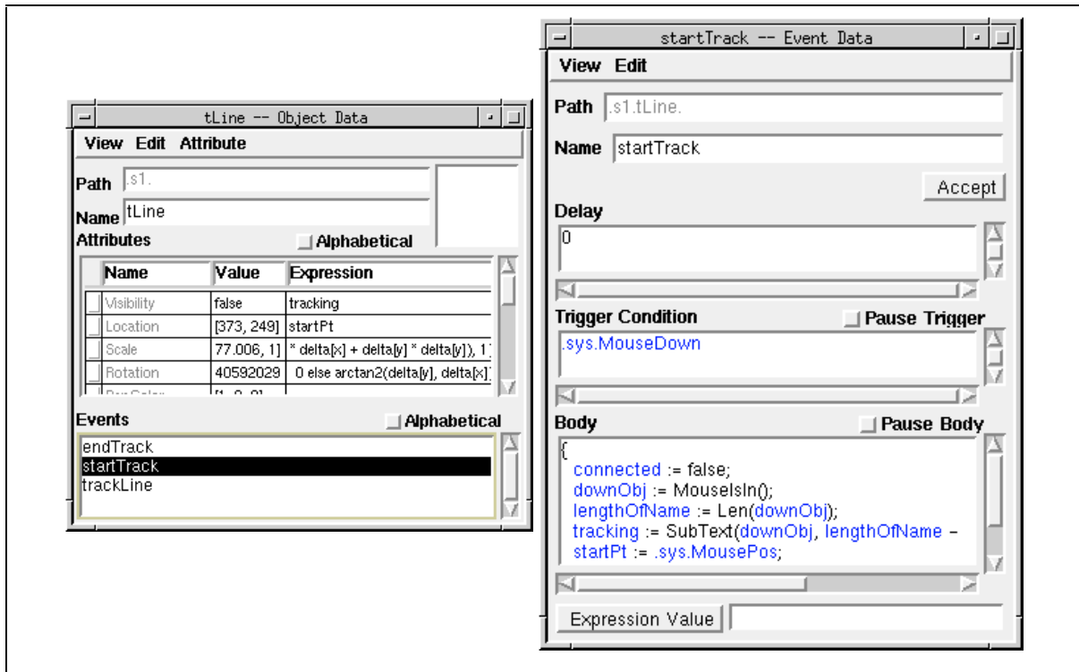
Figure 2-13: Interfaces de RIDES pour l'édition du modèle (d'après [Mun 95a])
