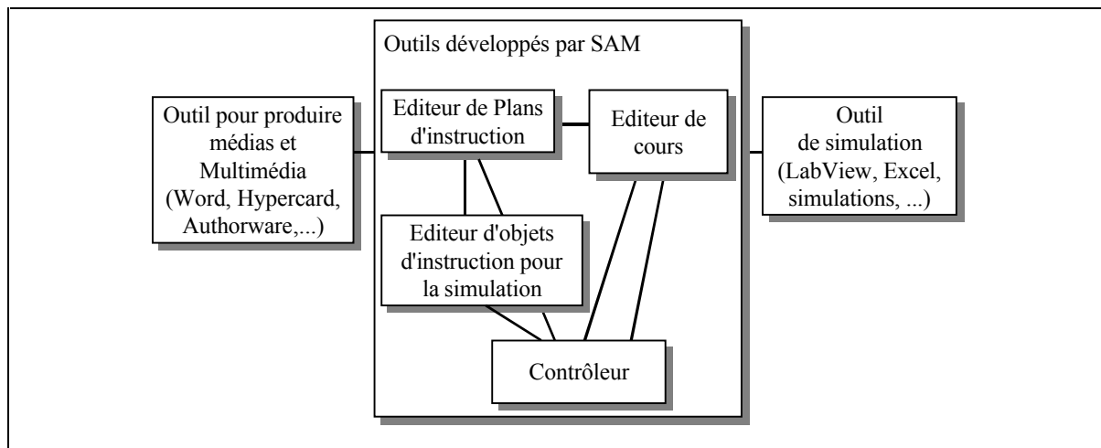
Figure 2-1 : Architecture proposée par SAM
