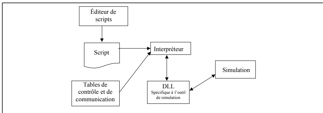
Figure 7-3: SAM : Réalisation et exécution de programmes pour le contrôle de simulations
