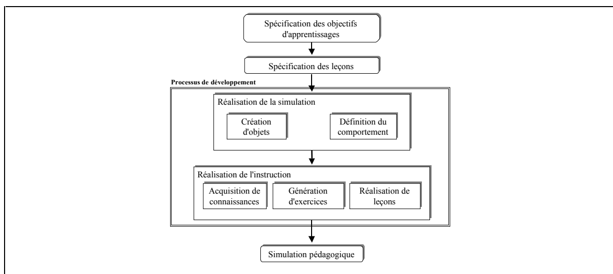
Figure 2-3: Processus de développement avec RIDES
