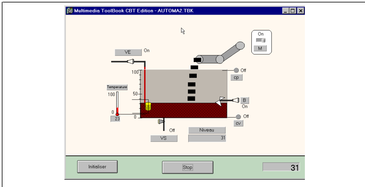
Figure 4-7: Interface de la simulation de la machine pour le dosage automatique
