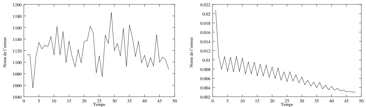
FIG. V.5 – La norme de l'erreur d'initialisation (à gauche) et optimale (à droite) en fonction du temps quand \beta = 1 .
