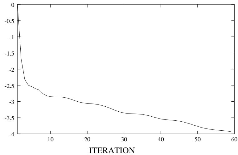
FIG. IV.8 – La variation de \log(\|\nabla J_k\|/\|\nabla J_0\|) en fonction des itérations k sur l'assimilation de 30 jours.
