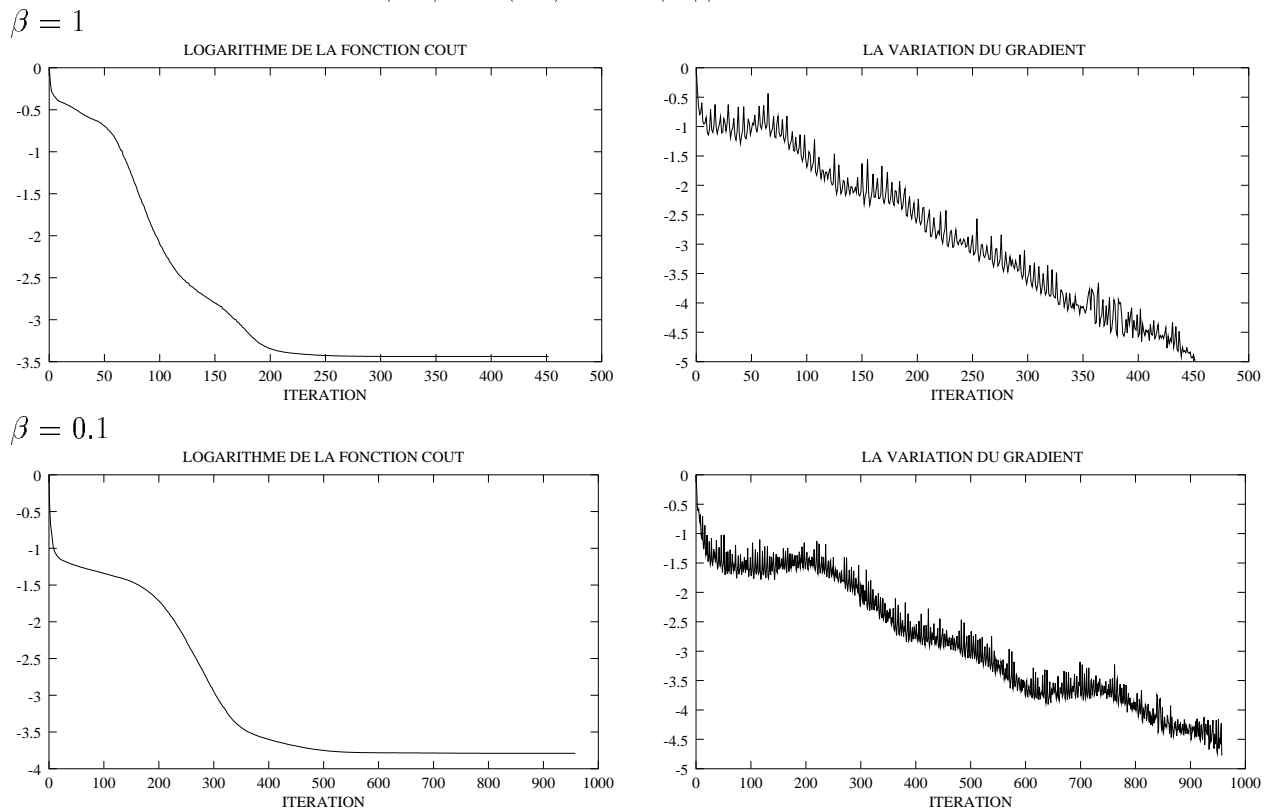
FIG. V.4 – Les figures à gauche décrivent la variation de \log(J_k/J_0) en fonction des itérations k , alors qu'à droite décrivent la variation de \log(\|\nabla J_k\|/\|\nabla J_0\|) .
